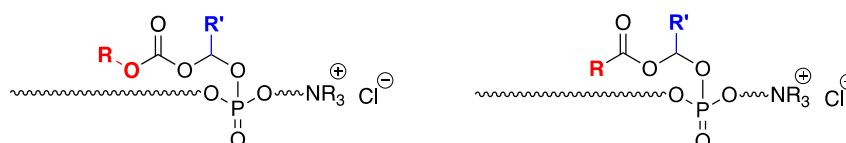
Figure 45. Structure générale des pro-APLs en série phosphoacétal de carbonate et phosphoacétal d'ester.
