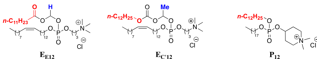
Figure 48. Nomenclature simplifiée des pro-APLs avec trois exemples en série "érufossine" et "pérfossine".
