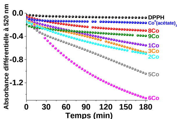
Figure 14 : Réactivité (oxygénation/activation) des différents complexes de cobalt(II) en présence de DPPH ; [Complexe] \sim 3 \times 10^{-4} M , [Complexe]/[DPPH] = 1,0 , solvant : dioxane, l = 1 cm , T = 25,0(2) ^\circ C .
