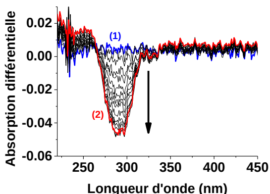
Figure 5 : Spectres d'absorption différentielle mesurés à intervalles réguliers durant la première phase d'oxygénation de 8Co ; (1) t = 0 , (2) t = 2 h, [8Co] = 2 \times 10^{-4} M, solvant : dioxane:H 2 O (1:1 v/v), l = 1 cm.
