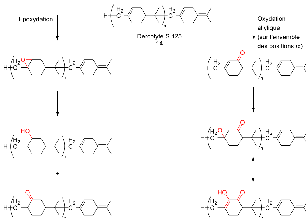
Schéma 12 : Produits d'oxydation suggérés et leur mécanisme de formation putatif. Pour l'oxydation allylique, les deux positions \alpha peuvent être impliquées, seuls les produits d'oxydation résultant d'une position \alpha sont décrits ici.
