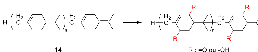
Schéma 11 : Oxydation aérobie assistée par catalyse métallique proposée pour l'additif polymérique 14 .
