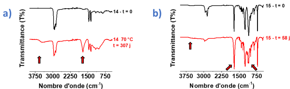
Figure 17 : Spectres IRTF de 14 (a) et 15 (b) initialement et après 307 et 68 jours d'oxydation à 70\text{ °C} respectivement.
