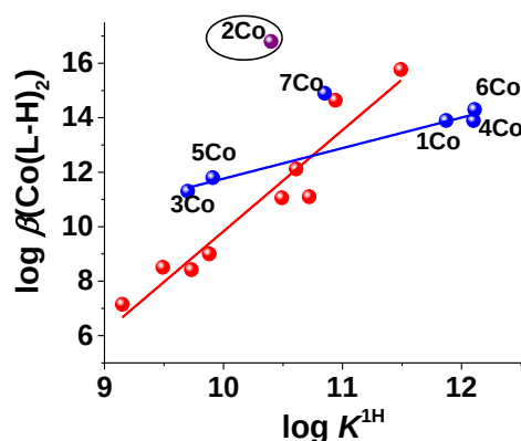
Figure 3 : Relation entre la constante globale de stabilité des complexes de cobalt(II) et les propriétés acido-basiques d'une large gamme de bases de Schiff, incluant celles d'intérêt dans cette étude.
