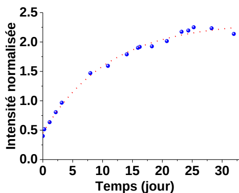
Figure 12 : Cinétique d'oxydation de 1Co et de conversion en trischélate de cobalt(III) suivie par RMN ^1\text{H} ; solvant : (\text{CD}_3)_2\text{SO} .
