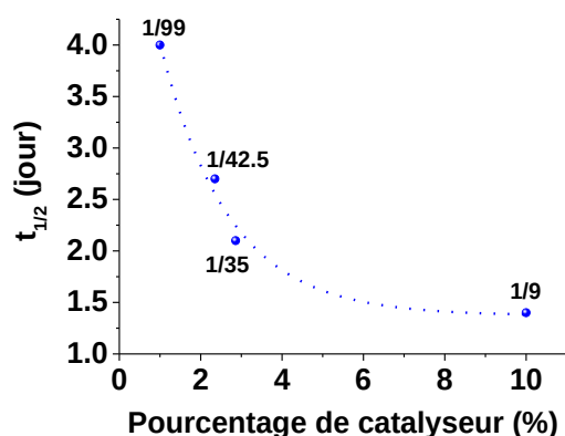
Figure 22 : Temps de demi-vis de la réaction d'oxydation de l'additif 15 en présence de cobalt(II) stéarate 9Co-2 à température ambiante en fonction du ratio catalyseur/additif.
