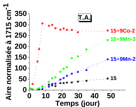
Figure 21 : Aire normalisée à 1715 \text{ cm}^{-1} démontrant l'oxydation de l'additif 15 à température ambiante que ce soit seul ou en présence de catalyseur métallique.
