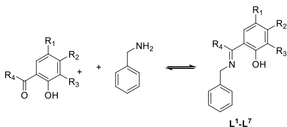
Schéma 6 : Synthèse des bases de Schiff.
