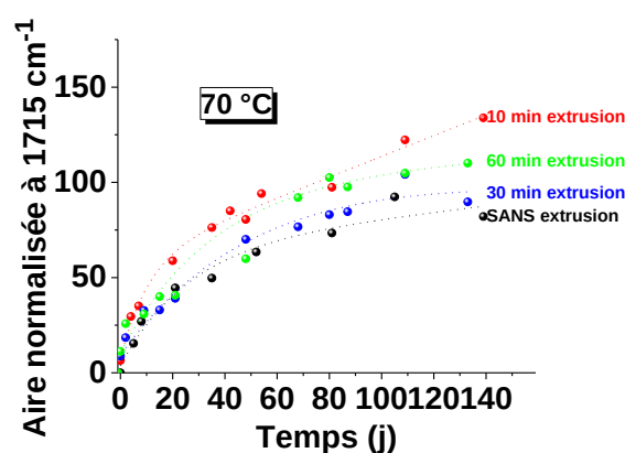
Figure 19 : Aire normalisée à 1715\text{ cm}^{-1} illustrant l'oxydation de 14 avec 9Mn-2 à 70\text{ °C} après 0, 10, 30 et 60 minutes d'extrusion.
