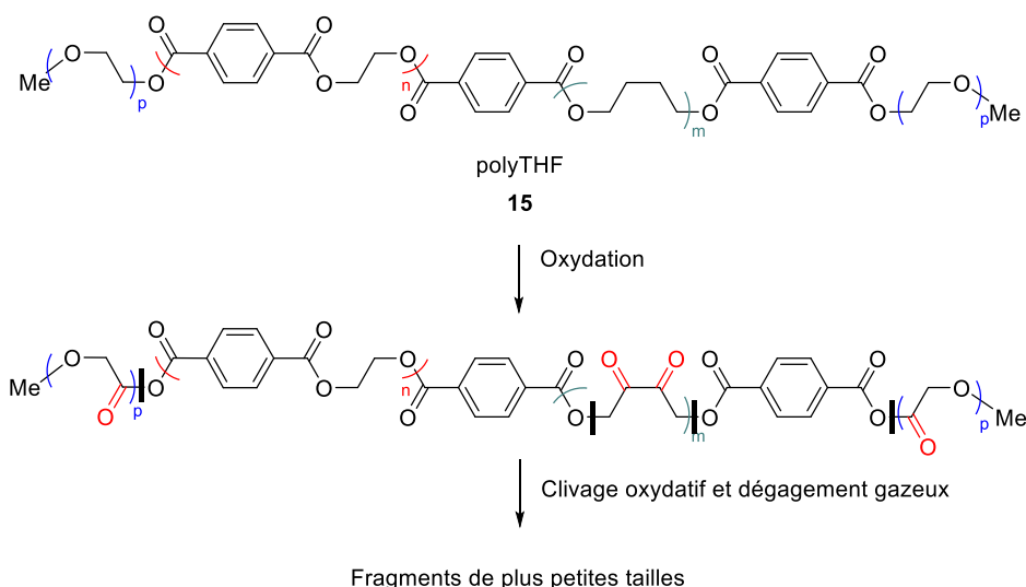
Schéma 14 : Sites d'oxydation putatifs et produits formés à partir du clivage oxydatif de l'additif 15. Les lignes noires indiquent les potentiels points de clivage.
