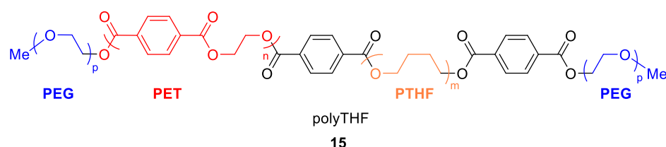
Schéma 13 : Structure chimique de l'additif polymérique 15 (PEG : polyéthylène glycol ; PET : polyéthylène téréphthalate ; PTHF : polytétrahydrofurane)
