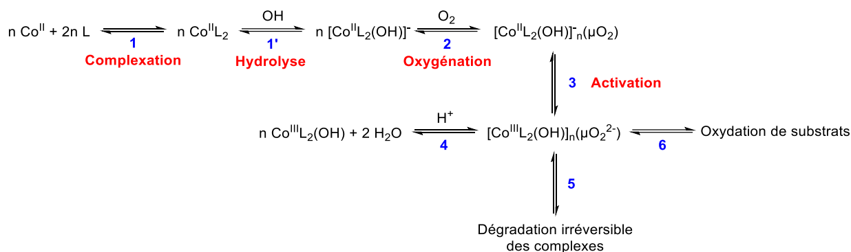
Schéma 1 : Mécanisme putatif de complexation, oxygénation et activation de complexes de cobalt(II).
