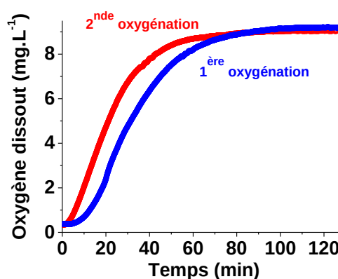
Figure 7 : Superposition des deux courbes d'oxygénation de 1Co durant les deux phases d'oxygénation ; [1Co] = 6 \times 10^{-4} M , solvant : dioxane:H 2 O (1:1 v/v).
