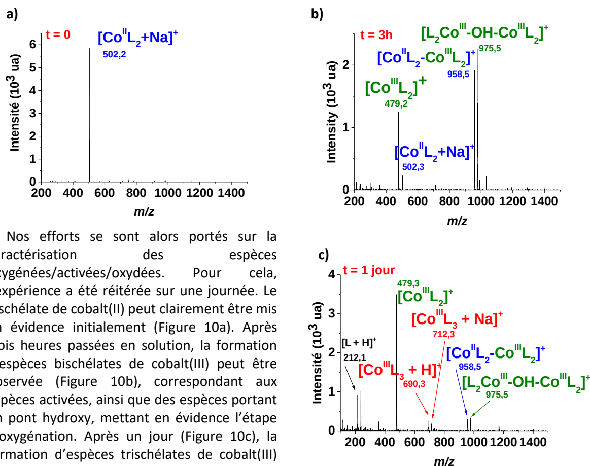
Figure 10 : Spectres de masse de 1Co enregistrés pendant une journée : a) t = 0 , b) t = 3 \text{ h} , c) t = 1 \text{ jour} , [1\text{Co}] = 6,97 \times 10^{-4} \text{ M} , solvant : dioxane, + 100 V.
