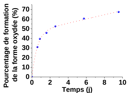
Figure 9 : Pourcentage de formation de l'espèce oxydée de 1Co pendant 10 jours.
