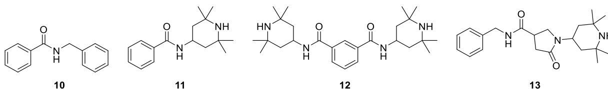
Schéma 4 : Additifs organiques modèles étudiés dans le cadre de ce travail de thèse.
