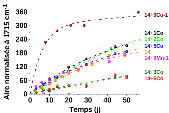
Figure 16 : Aire normalisée à 1715\text{ cm}^{-1} représentant l'oxydation de 14 à 70\text{ °C} en présence des différents catalyseurs métalliques.
