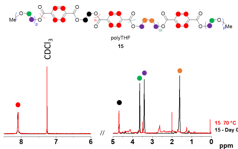
Figure 24 : Spectres RMN ^1\text{H} du polyTHF 15 avant (noir) et après (rouge) une oxydation prolongée à 70 °C, enregistrés dans le \text{CDCl}_3 à 500 MHz.
