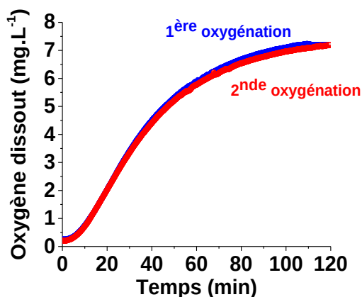
Figure 6 : Superposition des deux courbes d'oxygénation de 8Co durant les deux phases d'oxygénation ; [8Co] = 2 \times 10^{-4} M , solvant : dioxane:H 2 O (1:1 v/v).
