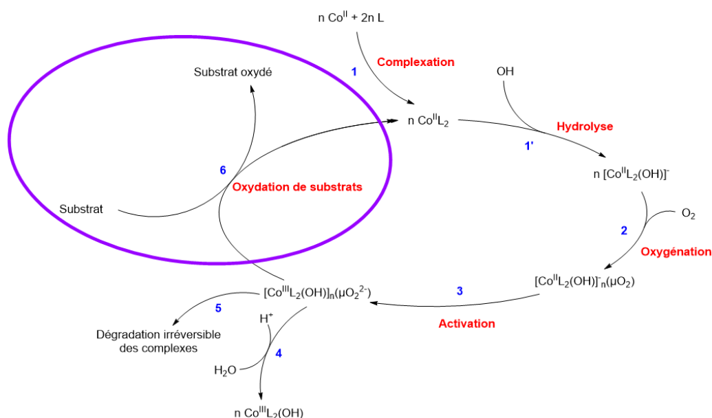
Schéma 8 : Mécanisme putatif de complexation, oxygénation et activation des complexes de cobalt(II).
