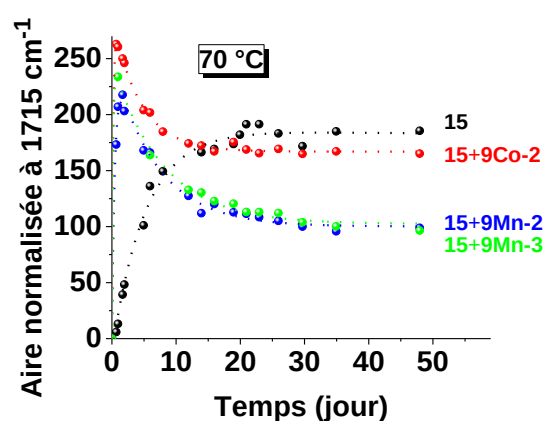
Figure 23 : Aire normalisée à 1715 cm -1 représentant l'oxydation de l'additif 15 seul ou avec 9Co-2 , 9Mn-2 ou 9Mn-3 à 70 °C.
