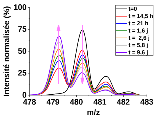
Figure 8 : Spectres de masse de 1Co enregistrés pendant 10 jours – zoom entre m/z = 478 et 483 ; [1Co] = 1,0 \times 10^{-4} M , solvant : CH 3 CN:H 2 O (1:1 v/v), + 170 V.
