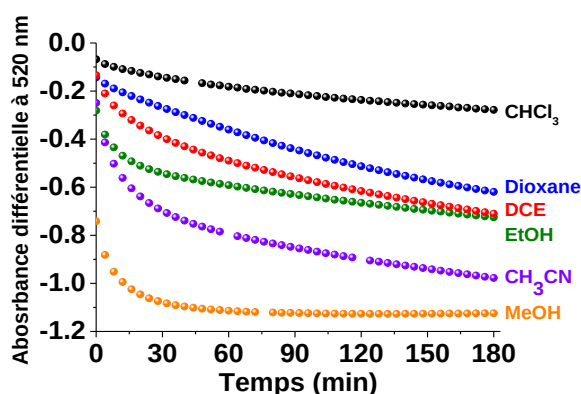
Figure 13 : Cinétique d'oxygénation/d'activation du complexe 1Co suivi en présence de DPPH dans différents solvants ; [1Co] \sim 3 \times 10^{-4} M , [1Co]/[DPPH] = 1,0 , l = 1cm , T = 25,0(2) ^\circ C .
