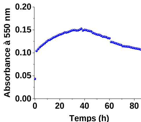
Figure 4 : Variations de l'absorbance à 550 nm de 1Co au cours du temps ; [1Co] = 2,51 \times 10^{-3} M, solvant : dioxane:H 2 O (1:1 v/v), l = 1 cm.
