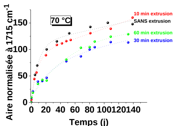
Figure 18 : Aire normalisée à 1715\text{ cm}^{-1} illustrant l'oxydation de 14 avec 9Co-2 à 70\text{ °C} après 0, 10, 30 et 60 minutes d'extrusion.
