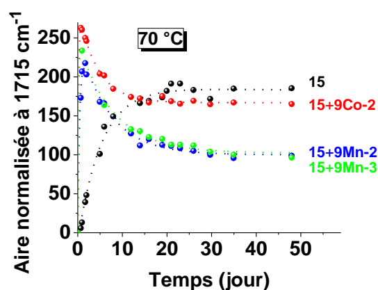
Figure 23 : Aire normalisée à 1715 \text{cm}^{-1} représentant l'oxydation de l'additif 15 seul ou avec 9Co-2 , 9Mn-2 ou 9Mn-3 à 70 °C.
