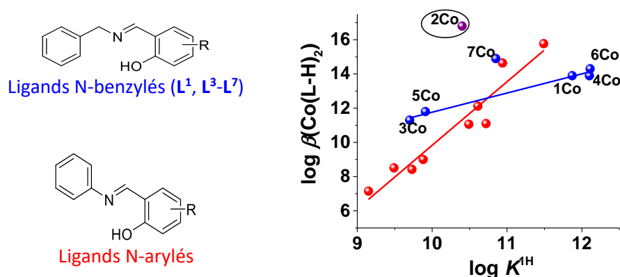
Figure 3 : Relation entre la constante globale de stabilité des complexes de cobalt(II) et les propriétés acido-basiques d'une large gamme de bases de Schiff, incluant celles d'intérêt dans cette étude.
