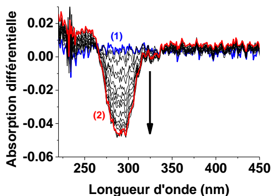
Figure 5 : Spectres d'absorption différentielle mesurés à intervalles réguliers durant la première phase d'oxygénation de 8Co ; (1) t = 0 , (2) t = 2 h, [8Co] = 2 \times 10^{-4} M , solvant : dioxane:H 2 O (1:1 v/v), l = 1 cm.
