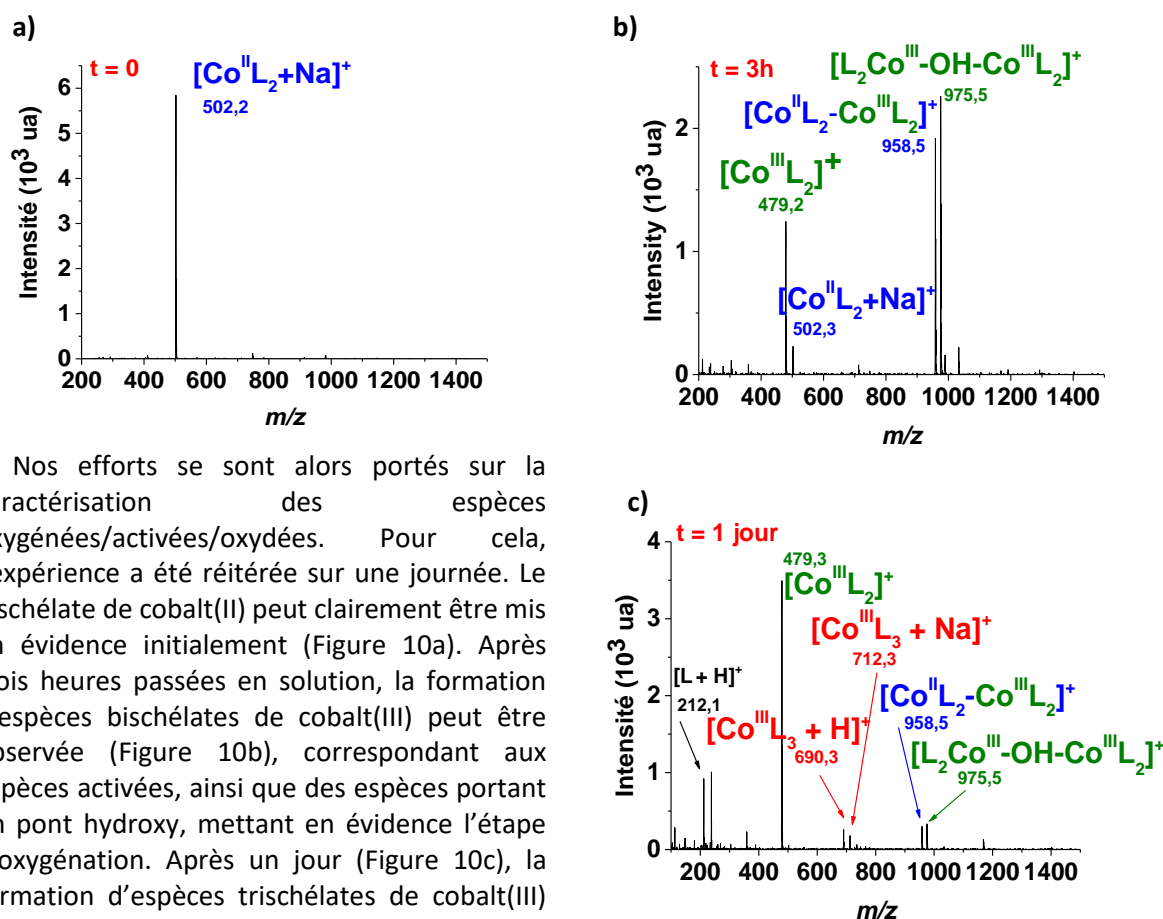
Figure 10 : Spectres de masse de 1Co enregistrés pendant une journée : a) t = 0 , b) t = 3 h, c) t = 1 jour, [1Co] = 6,97 \times 10^{-4} M, solvant : dioxane, + 100 V.
