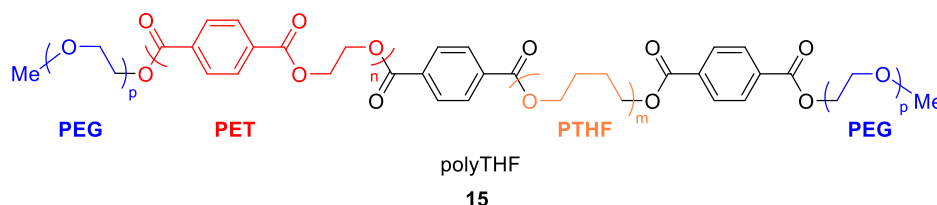
Schéma 13 : Structure chimique de l'additif polymérique 15 (PEG : polyéthylène glycol ; PET : polyéthylène téréphtalate ; PTHF : polytétrahydrofurane)
