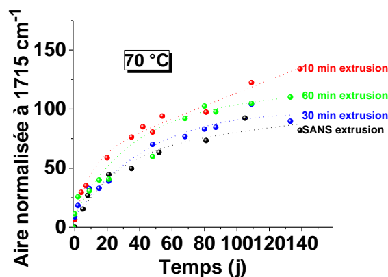
Figure 19 : Aire normalisée à 1715\text{ cm}^{-1} illustrant l'oxydation de 14 avec 9Mn-2 à 70\text{ °C} après 0, 10, 30 et 60 minutes d'extrusion.
