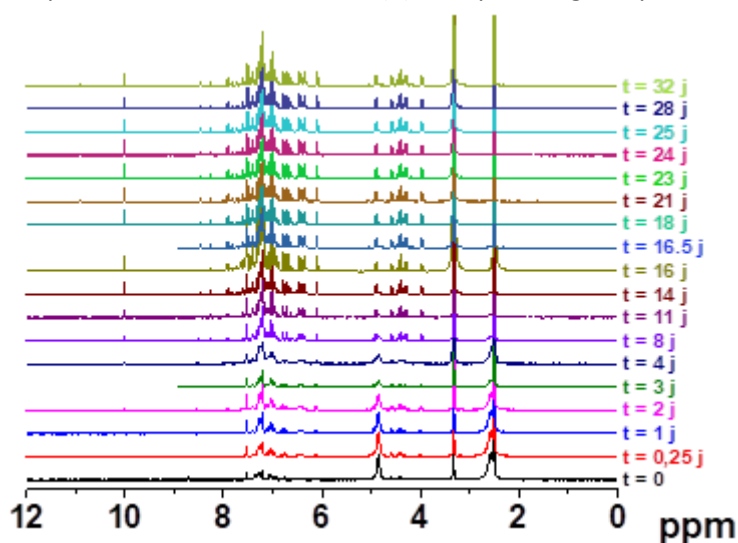
Figure 11 : Spectres RMN ^1H de 1Co enregistrés au cours du temps ; solvant : (CD_3)_2SO .
