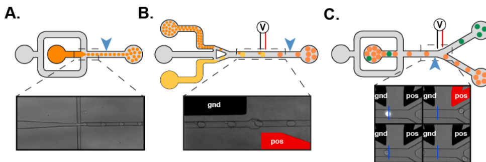
Figure 1 : Représentation schématique des modules microfluidiques. (A) Le générateur de gouttelettes pousse la phase aqueuse de PCR (en orange) vers l'huile fluorée (en gris) pour former des gouttelettes. La flèche bleue indique un point de mesure pour surveiller la monodispersité de l'émulsion par fluorescence. (B) Représentation du module de fusion. L'émulsion de PCR est réinjectée pendant qu'une deuxième émulsion est générée dans la puce (en jaune). Les deux émulsions sont synchronisées et fusionnées entre deux électrodes. (C) Schéma de la puce de tri des gouttelettes par leurs fluorescences (FADS). La fluorescence de chaque gouttelette est mesurée au niveau de la flèche bleue. Lorsque la gouttelette d'intérêt est détectée, un champ électrique est appliqué et extrait la gouttelette dans le canal de tri, sinon toutes les gouttelettes sont dirigées vers un autre canal.
