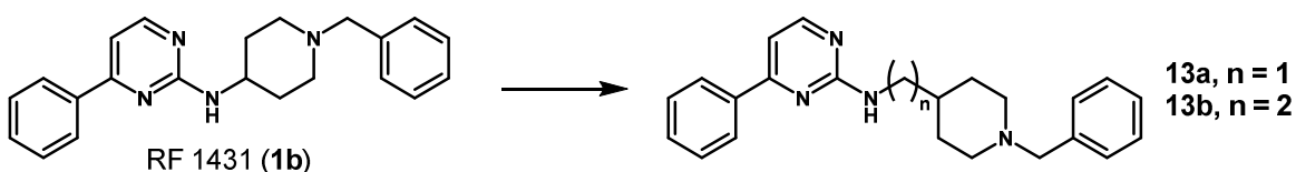
Figure 26. Eloignement de la plateforme 1-benzylpipéridine
