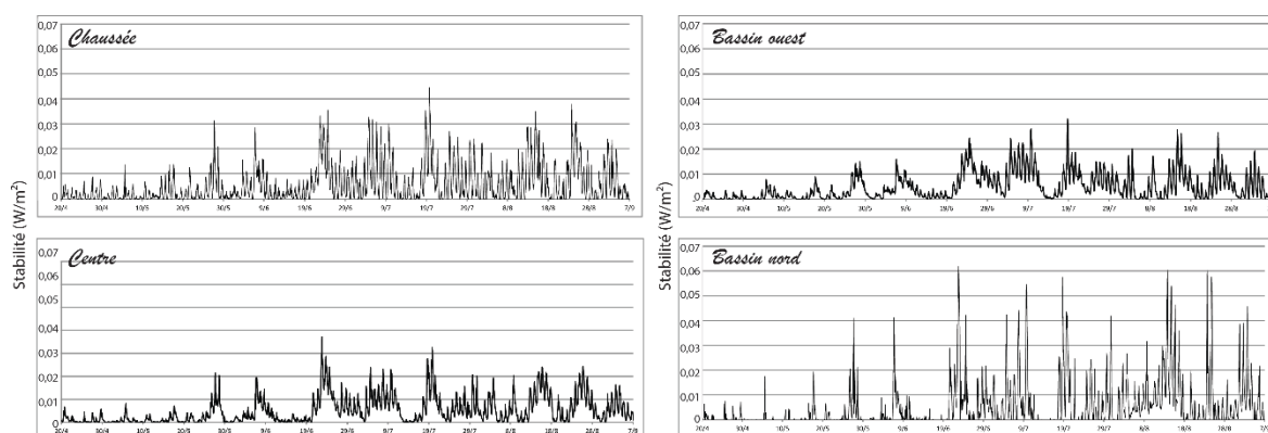
Figure 91: Variations horaires de la stabilité (en W/m^2 ) en plusieurs points de l'étang de la Ramade
