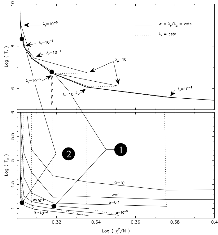
FIG. 4.2 – Exemple de ‘courbes L’ obtenues par inversion de six mois de données GONG (mois d’observations 4 à 10) avec différents choix de paramètres de régularisation. Ces données comprennent le développement sur des polynômes orthogonaux (jusqu’à a_9 ) des splittings de N = 2103 modes ayant des fréquences comprises entre 1200\mu\text{Hz} et 5000\mu\text{Hz} . Le logarithme des termes de régularisation en rayon (figure du haut) et en latitude (figure du bas) sont donnés en fonction du logarithme du \chi^2 normalisé par le nombre de mode. Les points correspondant au même choix de \lambda_r sont reliés par une ligne pointillée et les points correspondant au même choix du rapport \alpha = \lambda_r/\lambda_\mu sont reliés par une ligne pleine. Le point 1 montre le choix de \lambda_r = 10^{-3} et \lambda_\mu = 10^{-1} qui semble optimal d’après l’analyse de ces courbes (voir texte) alors que le point 2 montre un choix de paramètres qui correspond à une inversion moins régularisée qui peut s’avérer utile par exemple pour l’étude de la tachocline (voir chapitre 5)
