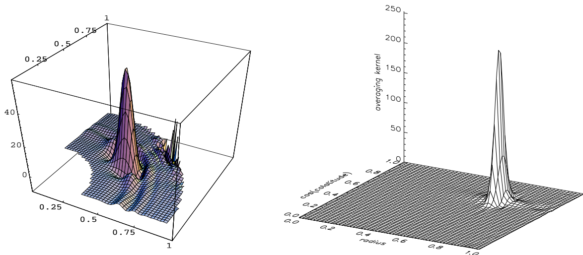
FIG. 3.9 – Exemples de noyaux de résolution 2D. A gauche , un noyau obtenu en ( r_0 = 0.55R_\odot , \mu_0 = 0.707 ) par une méthode RLS (graphique polaire) à partir des modes observés par BBSO (soit \sim 2300 coefficients a pour des modes 5 \leq l \leq 60 ). D'après Corbard et al. (1995). A droite , un noyau obtenu par une méthode OLA R^1 \otimes R^1 en r_0 = 0.7R_\odot , \mu_0 = 0.707 à partir de données simulées comprenant 70000 splittings ayant des degrés jusqu'à l = 250 (simulation de données GONG). D'après Sekii (1997). Il est à noter que les deux résultats ne sont pas directement comparables car le rayon r_0 ainsi que l'ensemble des modes utilisés diffèrent. Le manque de modes de degrés élevés dans les données BBSO peut notamment être en partie à l'origine des pics obtenus en surface par la méthode RLS. Néanmoins, d'après la figure précédente, ceux-ci restent une caractéristique de la méthode RLS.
