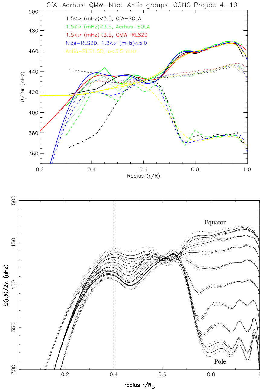
FIG. 4.4 – (a, en haut) Comparaison des profils de rotation obtenus pour trois latitudes (équateur, 30^\circ et 60^\circ ) par différentes méthodes d'inversion. Chaque méthode a été mise en oeuvre par un groupe différent au sein de la collaboration GONG. Les données utilisées correspondent aux données GONG du tableau 4.1, le domaine de fréquences retenu par chaque groupe étant indiqué sur la figure. Les résultats de l'inversion RLS 2D (groupe 'Nice') ont été obtenus avec le choix des paramètres de régularisation désignés par le point 1 sur la figure 4.2 des 'courbes L' (Résultats compilés par A. Eff-Darwich, communication privée). (b, en bas) Détails de la solution 2D RLS (groupe 'Nice') pour dix latitudes entre l'équateur et le pôle. L'examen des noyaux de résolution indique que la solution n'est pas fiable pour des rayons inférieurs à 0.4R_{\odot} et des latitudes supérieures à 60^\circ .
