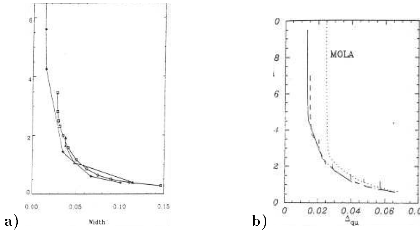
FIG. 3.6 – Exemples de ‘courbes L’ donnant le compromis entre la résolution ( \Delta_{qu} : largeur des noyaux de résolution, cf. §3.2.2) et les erreurs ( \sigma(\langle \Omega(r_0) \rangle) , cf. Eq. (3.33)) obtenues en r_0 = 0.5R_{\odot} . (a) Les trois courbes du cadre de gauche sont pour des méthodes MOLA (carrés), RLS (losanges), et asymptotique (triangles). D’après Christensen-Dalsgaard et al. (1990). (b) Le cadre de droite donne une comparaison entre les méthodes SOLA (trait plein) et MOLA (trait pointillé). D’après Pijpers & Thompson (1994).
