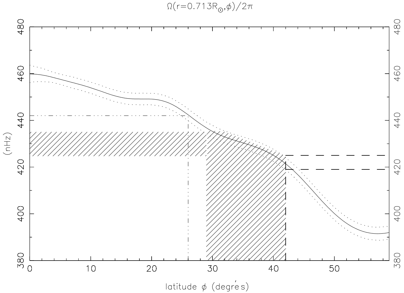
FIG. 5.6 – Variation de la rotation au fond de la zone convective ( r_{zc} = 0.713R_{\odot} ) en fonction de la latitude correspondant à la solution (Fig. 4.5) obtenue par inversion 2D des données MDI (—). Les lignes (.....) montrent les incertitudes à 1\sigma . La prédiction théorique de Spiegel et Zahn (1992) donne la valeur de la rotation rigide de la zone radiative comme étant égale à celle du fond de la zone convective à \Phi = 42^{\circ} de latitude qui conduit à une valeur de \Omega_0 comprise entre 419 nHz et 425 nHz (-----). Le domaine hachuré donne l'intervalle de confiance à 1\sigma pour \Omega_0 tel qu'il est déduit des données ( \Omega_0 = 430 \pm 5\text{nHz} , voir §4.3.2). Ceci correspond à un angle \Phi compris entre 29^{\circ} et 42^{\circ} . Les lignes (-.....) correspondent à la théorie de Gough (1985).
