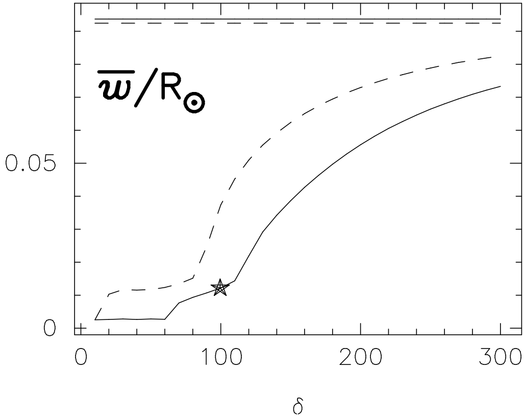
FIG. 5.4 – Variation, en fonction du paramètre \delta , de la largeur de la tachocline déduite de l'ajustement de la solution ARTUR par une fonction erf (cf. Eq. 5.20) (ligne pleine). Ce résultat correspond à l'inversion des données LOWL, le choix optimal de \delta ( \delta=100 ) désigné par les simulations de Monte-Carlo est montré par une étoile. La ligne pointillée indique le résultat obtenu, pour chaque \delta , par un ajustement de la solution avec une fonction erf sans partie linéaire (Eq. 5.1). Les lignes horizontales montrent le résultat (indépendant de \delta ) de l'ajustement de la solution RLS (Tikhonov). La largeur corrigée par une déconvolution locale utilisant les noyaux de résolution est w \simeq 0.06R_{\odot} .
