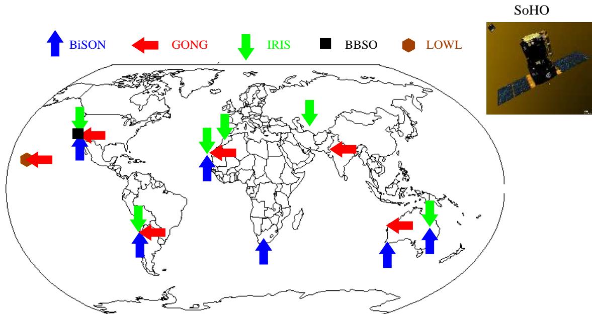
FIG. 5 – Localisation des principaux instruments dont les données ont été utilisées pour ce travail. IRIS, BiSON et GONG sont des réseaux d'observatoires, LOWL et BBSO deux instruments isolés et le satellite SoHO est situé au point de Lagrange L_1 entre la terre et le Soleil et comprend notamment les instruments VIRGO/LOI, GOLF et MDI (voir texte). Adapté de Pallé (1997)
