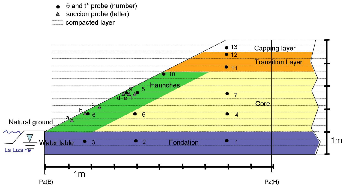
Figure 37 : localisation des capteurs au sein de l'ouvrage TerDOUEST. Leur emplacement permet d'observer les tendances dans les parties d'ouvrage suivantes : la couche de forme (blanc), la partie supérieure des terrassements (orange), le cœur de remblai (jaune), le talus (vert) et la base de remblai (violet)
