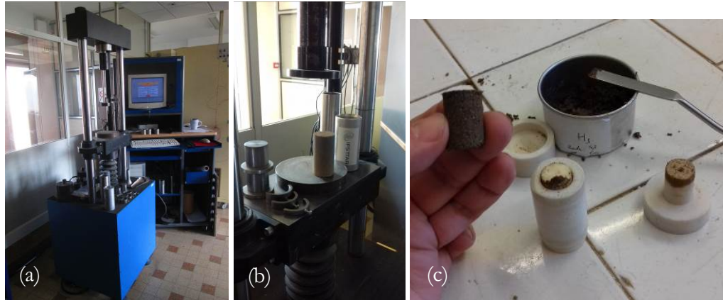
Figure 101 : Matériel de compactage utilisé (a) presse hydraulique, (b) vue d'une éprouvette 5×10 et du matériel de compactage, (c) vue d'une éprouvette 1,5×2 et du matériel de compactage manuel.
