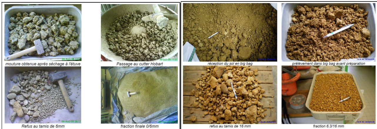
Figure 71 : Préparation de l'argile A3/A4 et du limon A2 du projet TerDOUEST (Froumentin, 2012)
