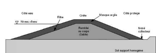
Figure 1.14 : Digue zonée à masque étanche sur fondation homogène ; à noter la nécessité d'une protection contre la dessiccation du masque en argile
