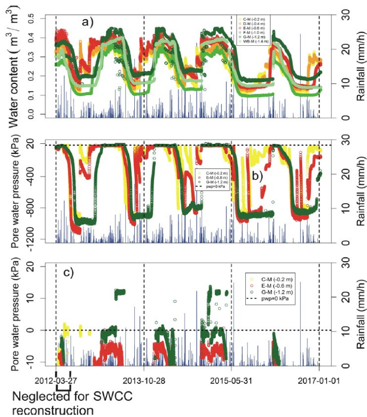
Figure 179 : (a) Teneur en eau (b) Mesure de succion (c) Mesure de succion dans la gamme -10 à 20 kPa. Evolution et relations avec la pluviométrie durant la période observée à Montuè (Italie) de 2012 à 2017 (Bordoni et al., 2017).
