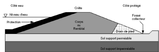
Figure 1.8 : Digue homogène sur fondation perméable sans ancrage étanche
