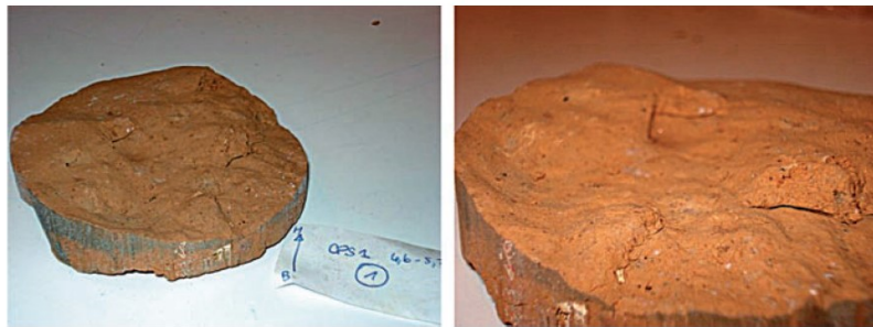
Figure 80 : Aspect de la discontinuité observée dans une carotte [du remblai expérimental] (Vinceslas et al., 2009)
