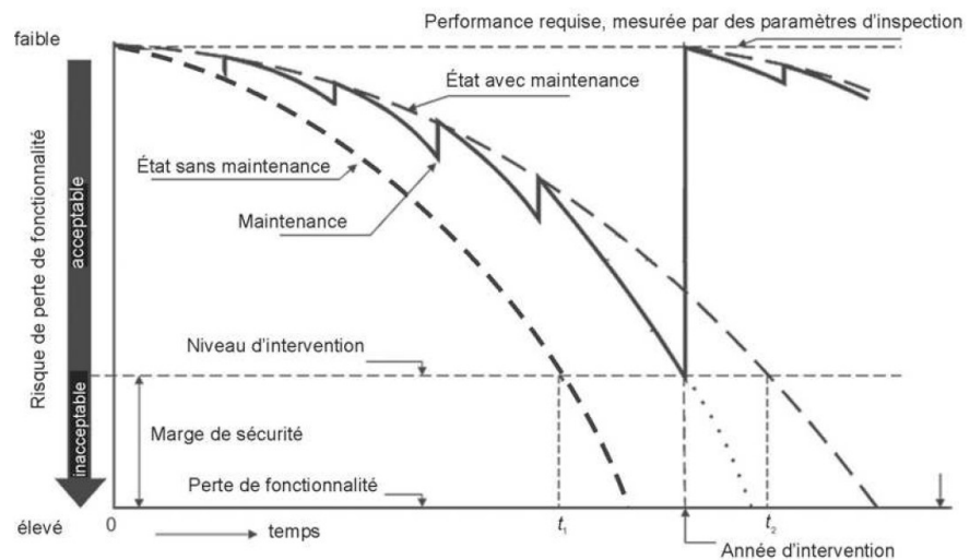
Figure 14 : Courbe de dégradation d'un ouvrage en enrochement avec maintenance (trait plein) et sans maintenance (en tireté gras) (Ciria, 2003)
