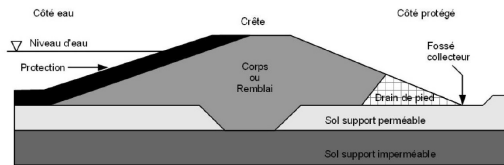
Figure 1.9 : Digue homogène sur fondation perméable avec ancrage d'étanchéité
