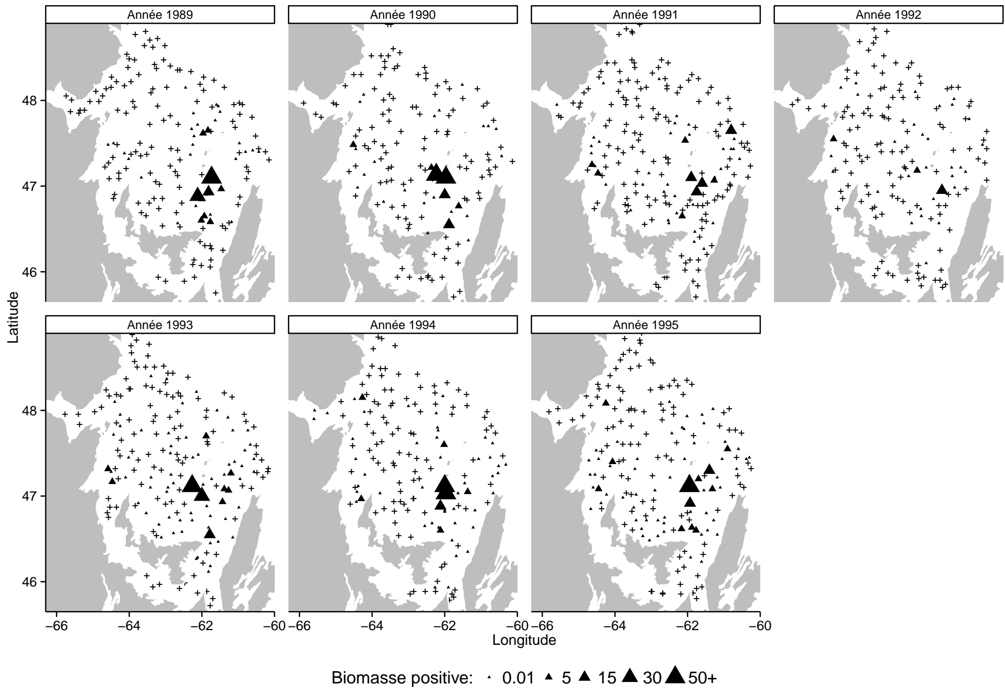
FIGURE 5.14 : Quantité de biomasses de concombre de mer récoltées sur l'ensemble su sGSL pour les années 1989 à 1995. Les triangles représentent les quantités de biomasses non nulles, les croix représentent l'absence de l'espèce.
