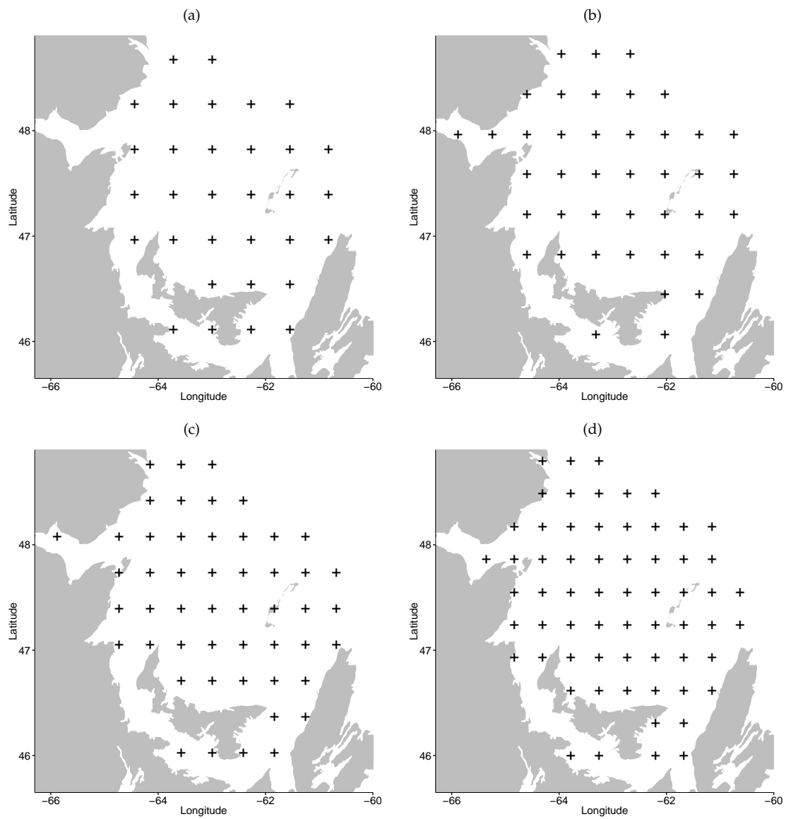
FIGURE 5.5 : Grilles régulières construites sur l'ensemble du sud du golfe du Saint-Laurent. (a) Grille régulière de 32 points séparés de 47 km . (b) Grille régulière de 41 points séparés de 42 km . (c) Grille régulière de 50 points séparés de 38 km . (d) Grille régulière de 63 points séparés de 35 km .
