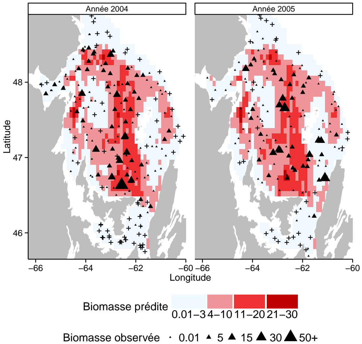
FIGURE 5.12 : Prédications et observations des quantités de biomasses d'oursins sur l'ensemble du sGSL pour les années 2004 et 2005 (les croix représentent les quantités de biomasses observées nulles).
