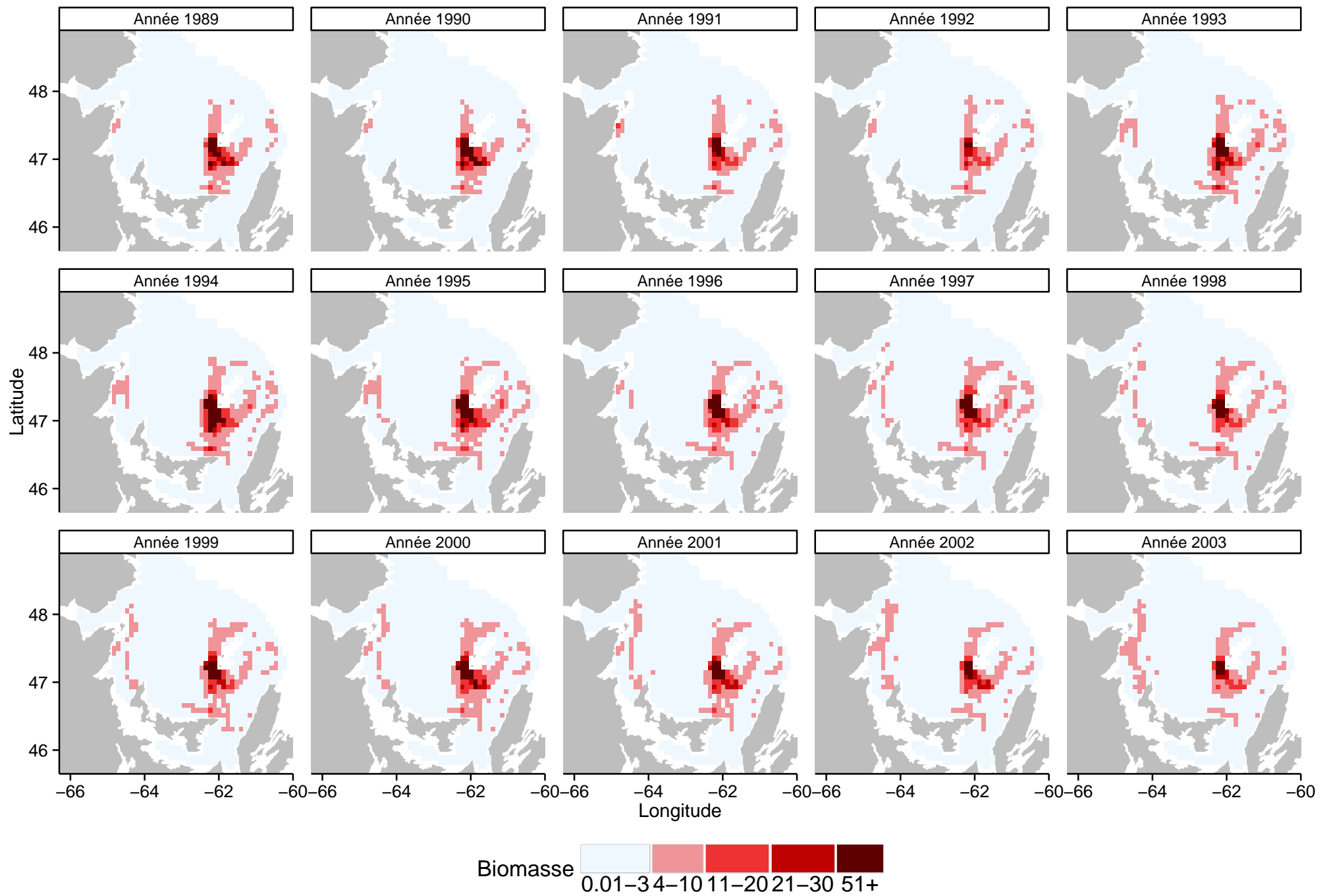
FIGURE 5.16 : Biomasse de concombre de mer prédite sur l'ensemble su sGSL pour les années 1989 à 2003 (grille régulière, \phi = 18 et G = 63 ).
