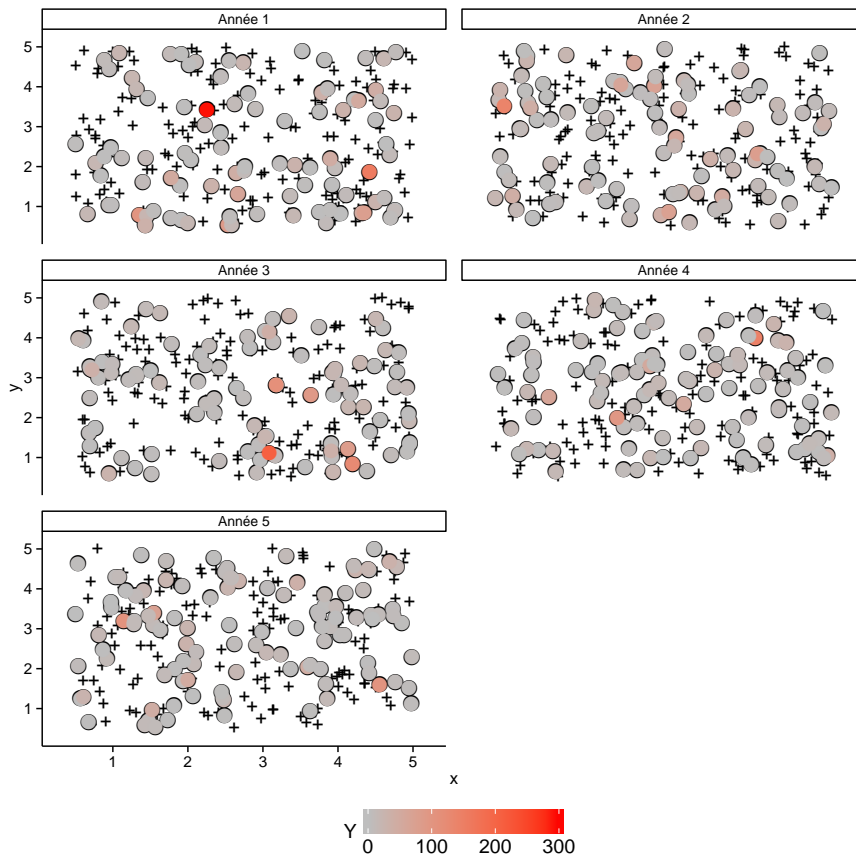
FIGURE 5.3 : Données simulées pendant 5 années ( a = 1 , b = 0.2 , \mu = 0.1 , \sigma_x = 2 , \phi = 0.5 , \sigma_v = 0.1 , et \delta = 0.9 ).
