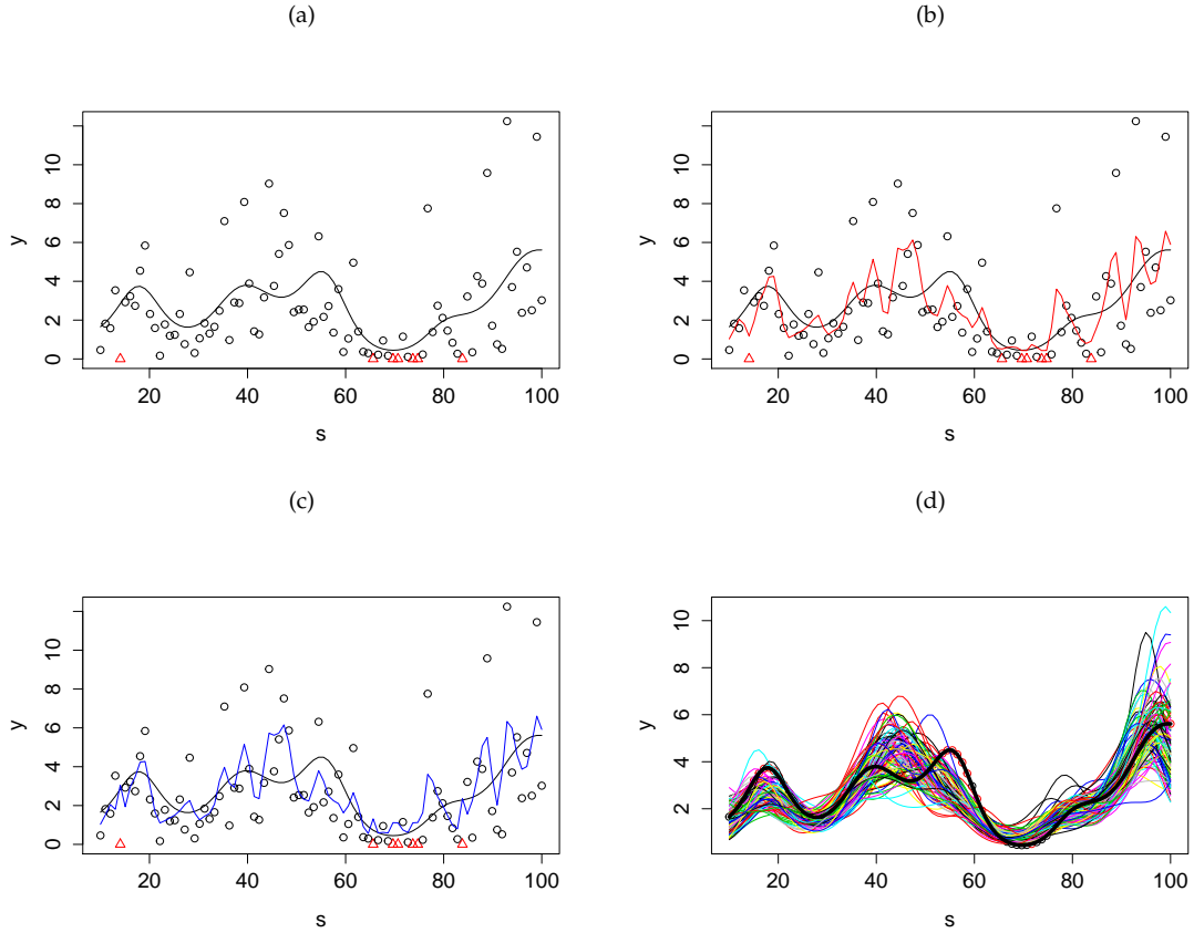
FIGURE B.1 : Visualisation d'une configuration de grille linéaire. (a) Couche latente et données. (b) Estimateur obtenu par lissage. (c) Estimateur débiaisé. (d) 100 Champs latents auxiliaires.
