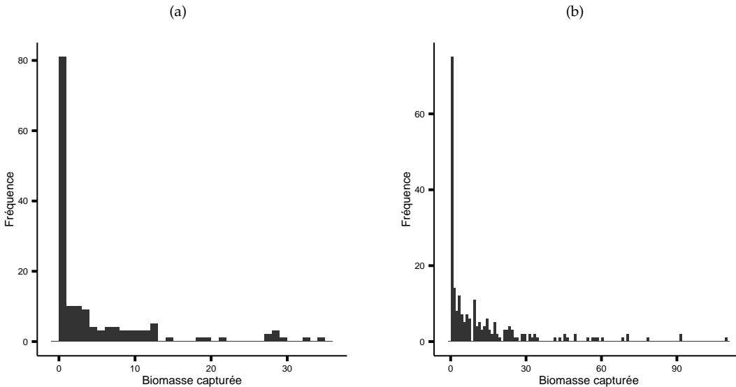
FIGURE 1.3 : Histogrammes des captures (en kg ) effectuées par le MPO en 2005. (a) Captures d’oursins effectuées dans le sGSL. (b) Captures de sole ( Microstomus pacificus ) effectuées dans le bassin de la Reine-Charlotte.
