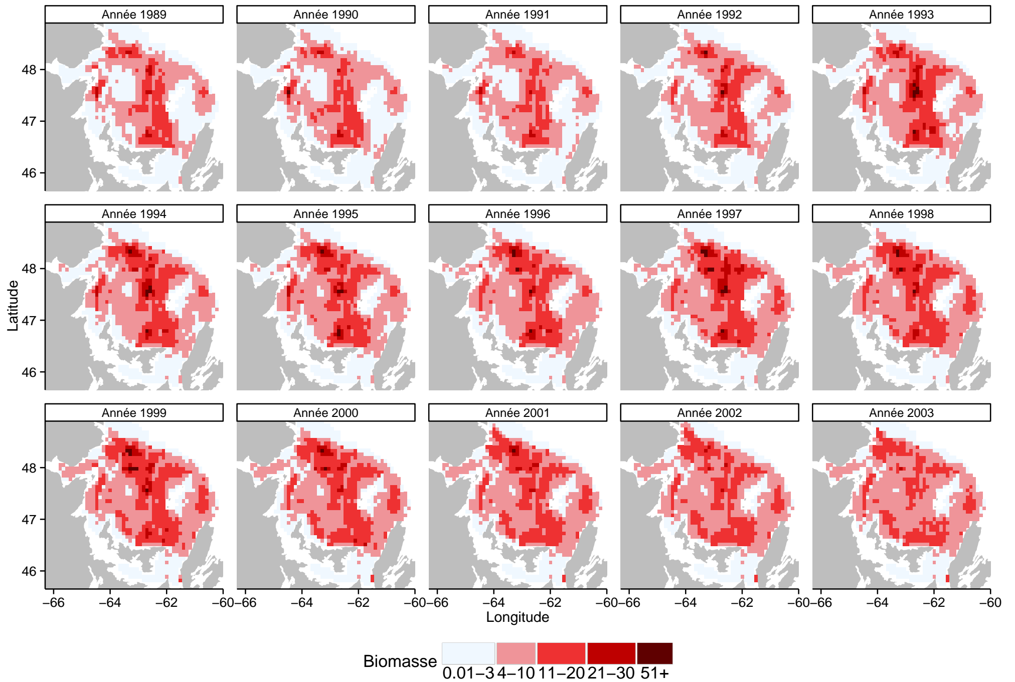
FIGURE 5.11 : Biomasse d'oursins prédite sur l'ensemble su sGSL pour les années 1989 à 2003 (grille régulière, \phi = 18 et G = 41 ).
