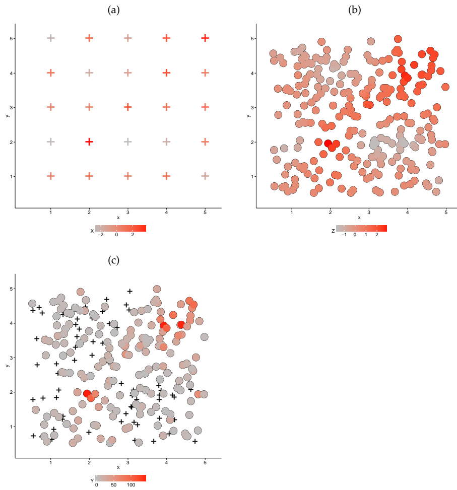
FIGURE 5.1 : Données simulées ( S = 250 et G = 25 ) avec les paramètres ( a = 1, b = 0.2, \mu = 0.1, \sigma_x^2 = 2, \phi = 0.5 ). (a) Première étape simuler sur une grille , (b) deuxième étape simuler le champ latent , (c) enfin simuler les observations (les croix représentent des valeurs nulles).
