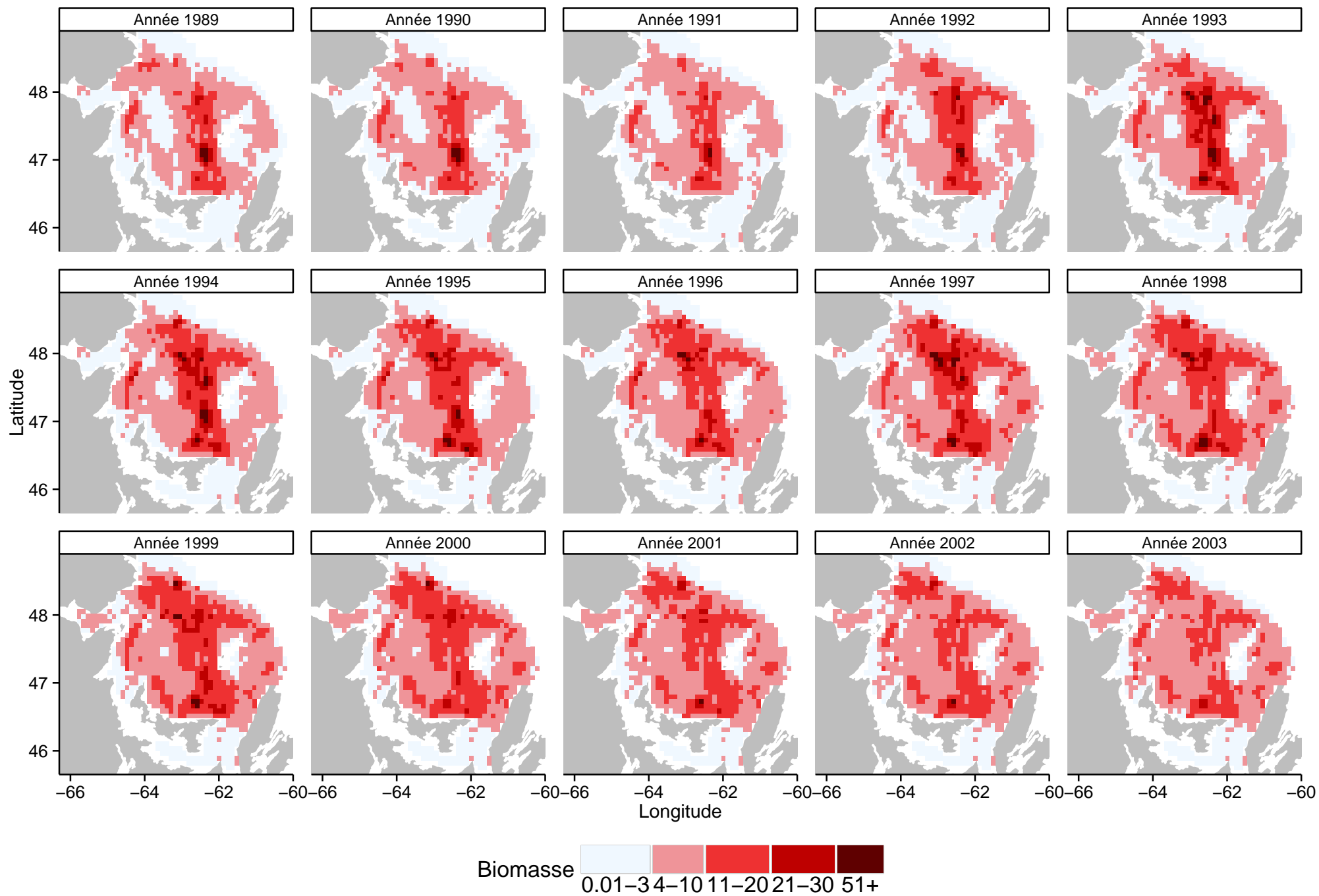
FIGURE 5.13 : Biomasse d'oursins attendue sur l'ensemble su sGSL pour les années 1989 à 2003 (grille irrégulière, \phi = 18 et G = 41 ).
