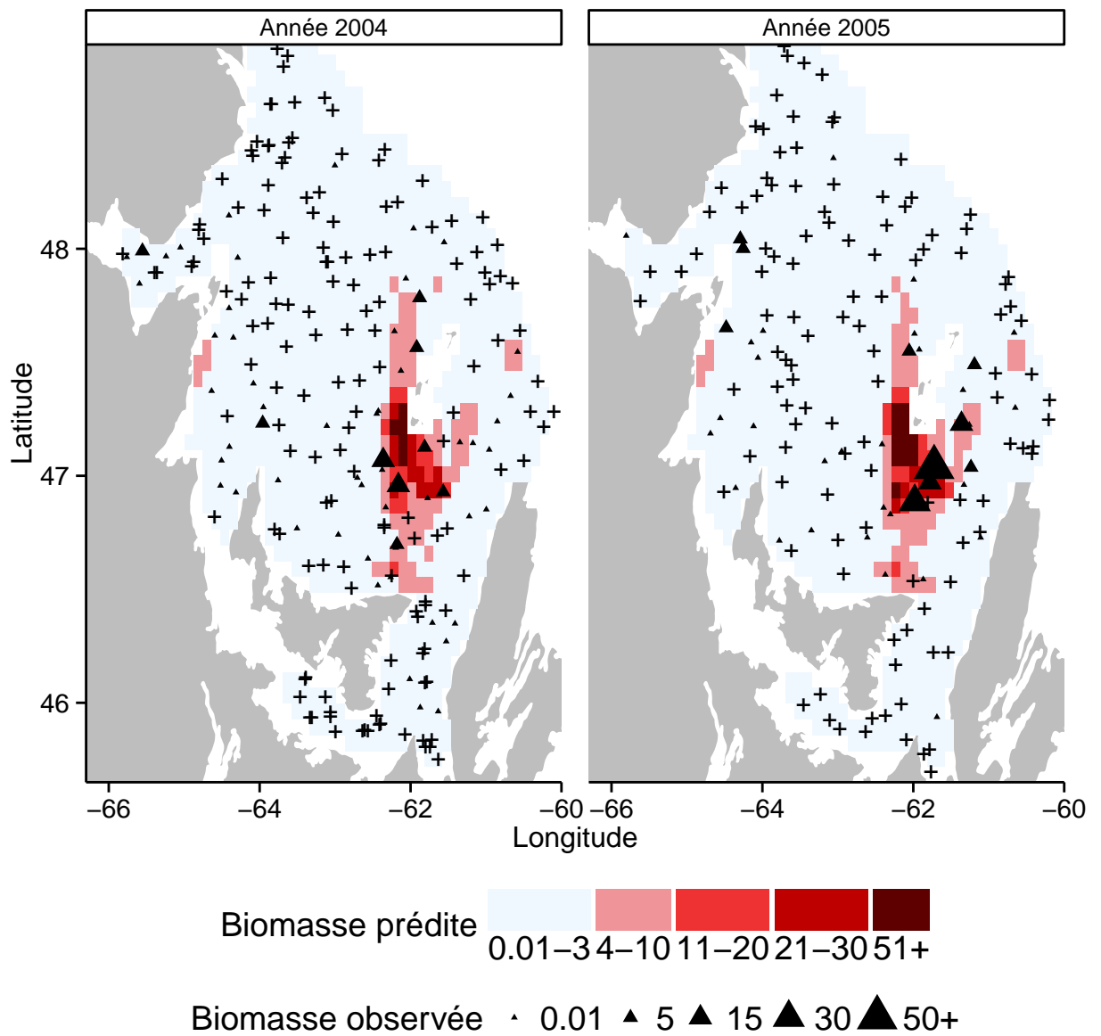
FIGURE 5.17 : Prédications et observations des quantités de biomasses de concombre de mer sur l'ensemble du sGSL pour les années 2004 et 2005 (les croix représentent les quantités de biomasses observées nulles).
