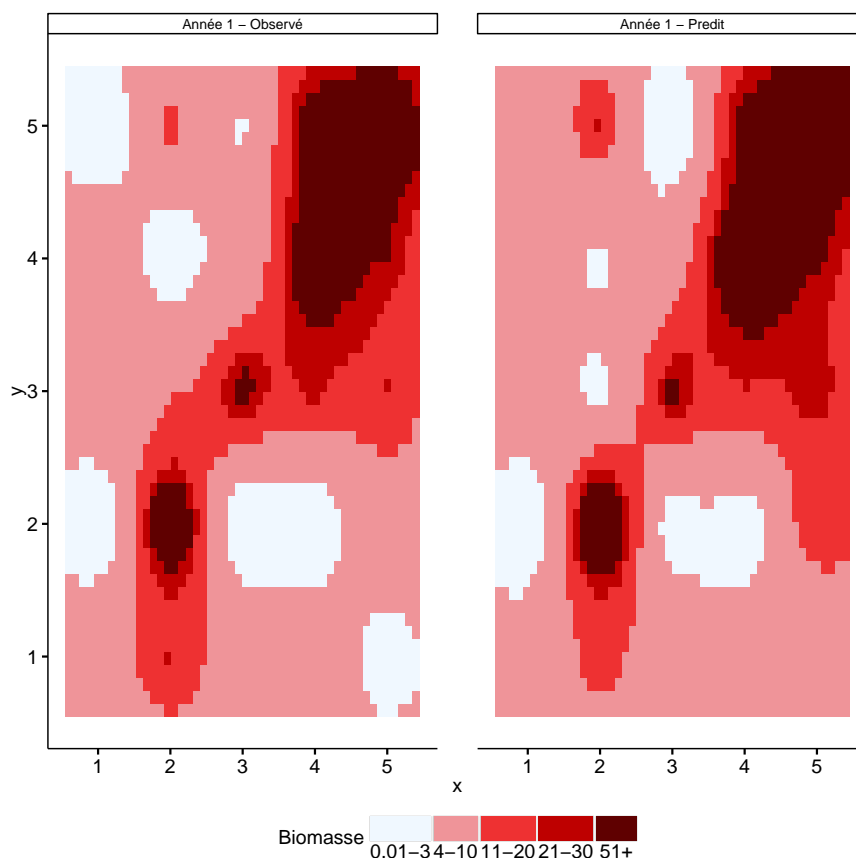
FIGURE 5.2 : Champ latent simulé et champ latent estimé sur l'ensemble de la zone d'étude.
