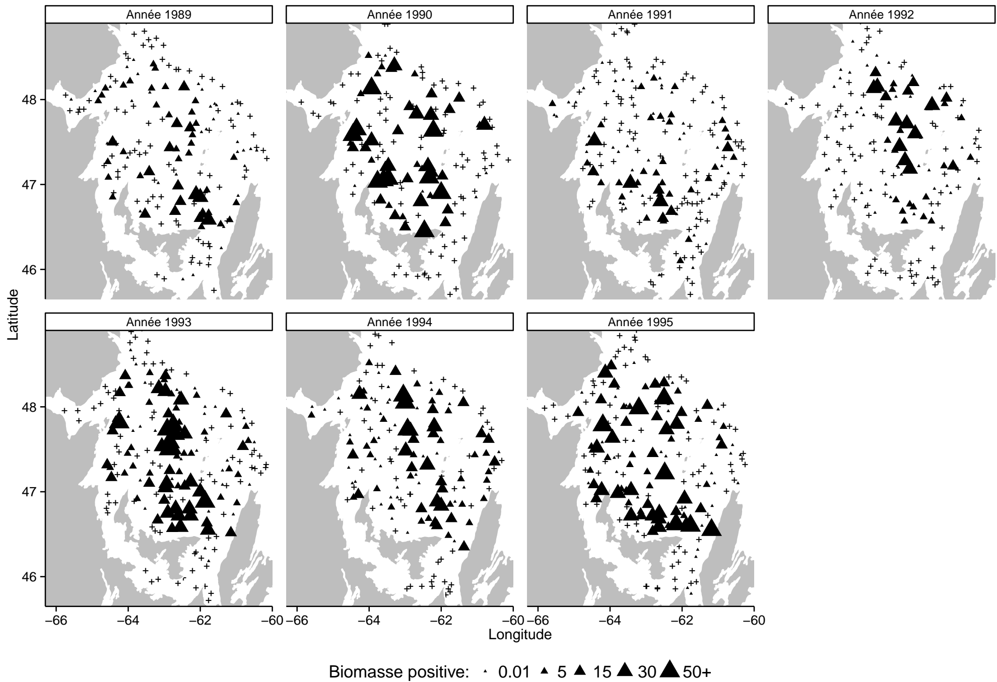
FIGURE 5.9 : Quantité de biomasses d'oursins récoltées sur l'ensemble su sGSL pour les années 1989 à 1995. Les triangles représentent les quantités de biomasses non nulles, les croix représentent l'absence de l'espèce.
