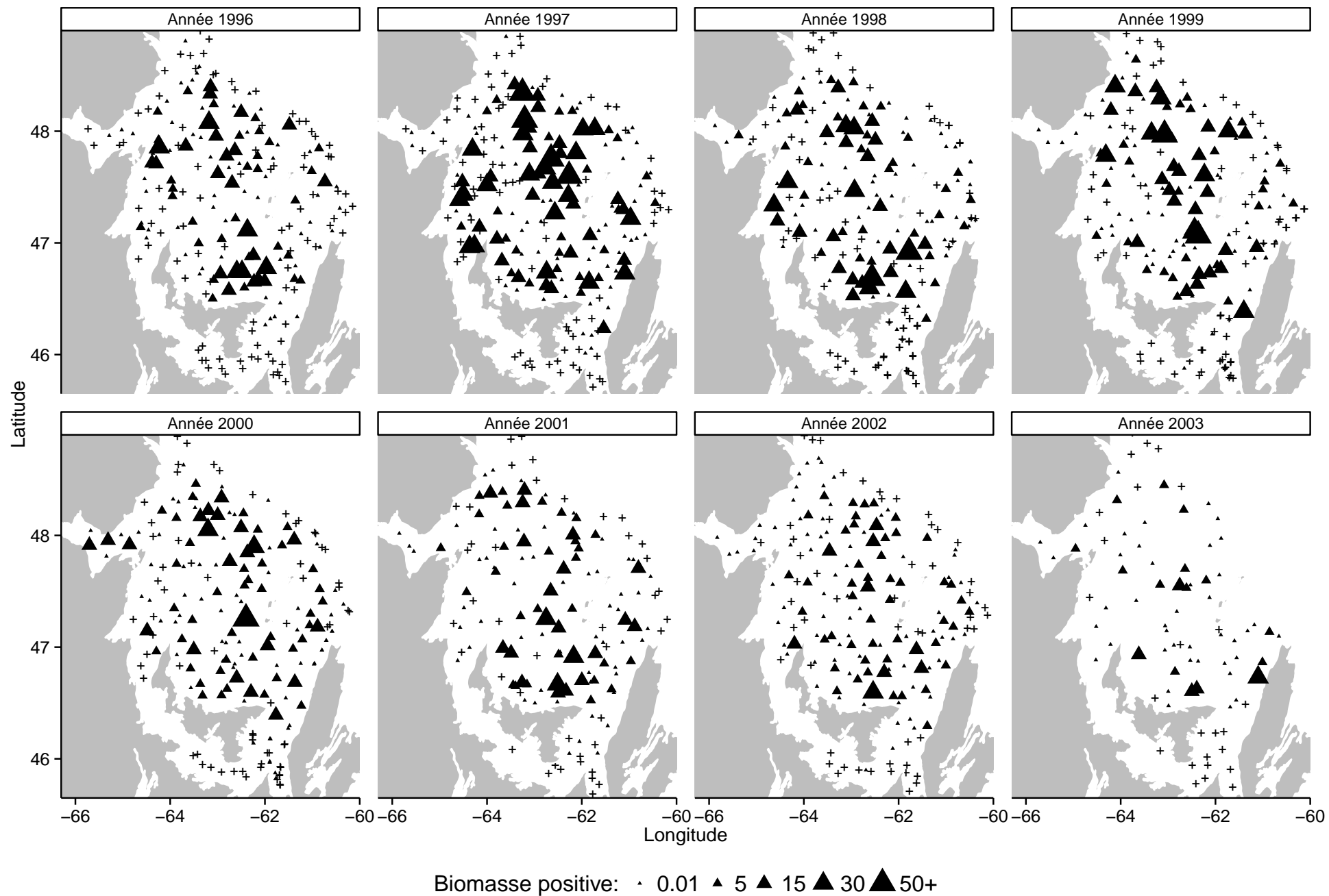
FIGURE 5.10 : Quantité de biomasses d'oursins récoltées sur l'ensemble su sGSL pour les années 1996 à 2003. Les triangles représentent les quantités de biomasses non nulles, les croix représentent l'absence de l'espèce.
