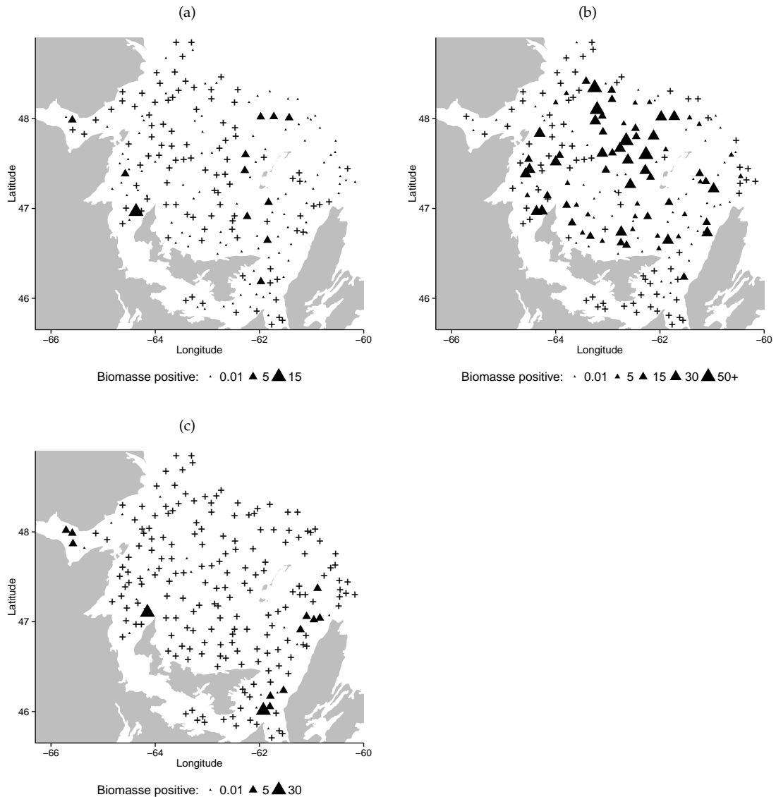
FIGURE 6.1 : Quantités de biomasses récoltées en 1997 dans le golfe du Saint-Laurent : (a) étoile de mer , (b) oursin, (c) ophiure.
