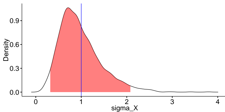
FIGURE B.3 : Distribution a posteriori du paramètre \sigma_x^2 , variance des points de grille. La zone rouge représente l'intervalle à 95% a posteriori . La valeur simulée du paramètre \sigma_x^2 est représentée par la ligne bleue.
