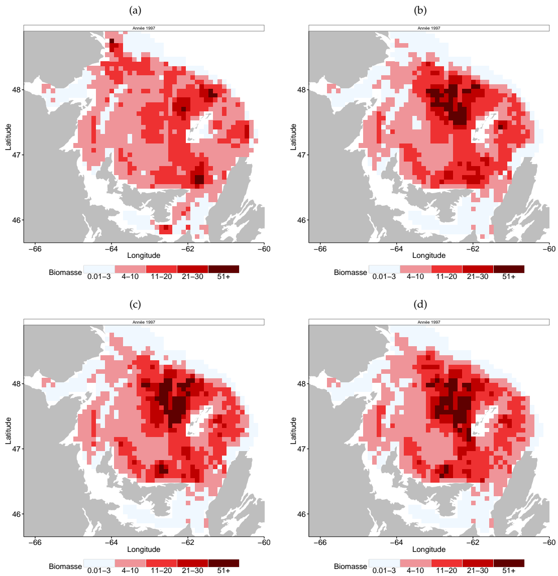
FIGURE 5.8 : Biomasse d'oursins attendue sur l'ensemble du sGSL pour l'année 1997. (a) Grille irrégulière de 32 points. (b) Grille irrégulière de 4. (c) Grille irrégulière de 50 points. (d) Grille irrégulière de 63 points.
