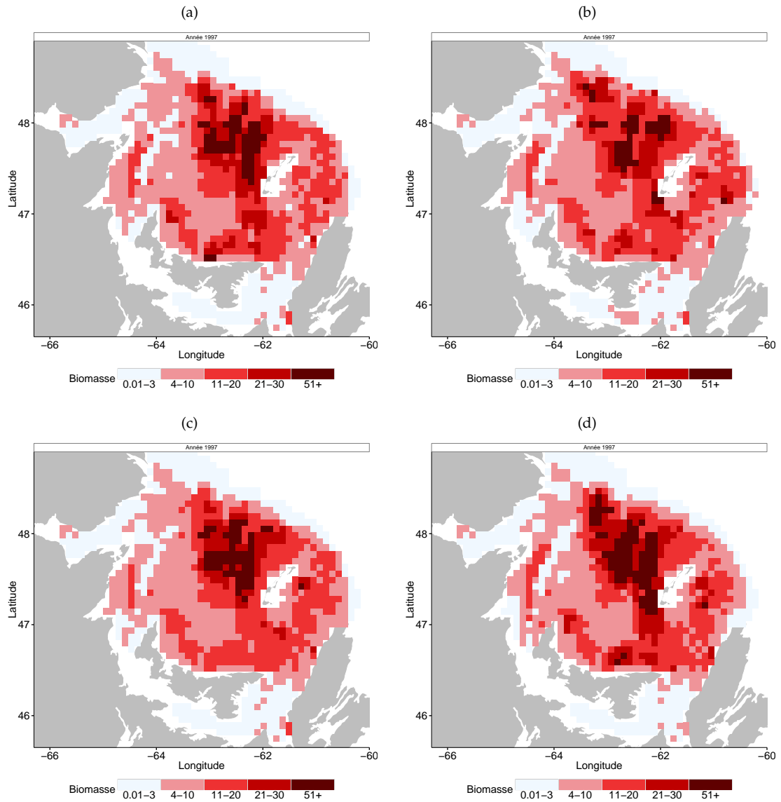
FIGURE 5.7 : Biomasse d'oursins attendue sur l'ensemble du sGSL pour l'année 1997. (a) Grille régulière de 32 points. (b) Grille régulière de 41. (c) Grille régulière de 50 points. (d) Grille régulière de 63 points.
