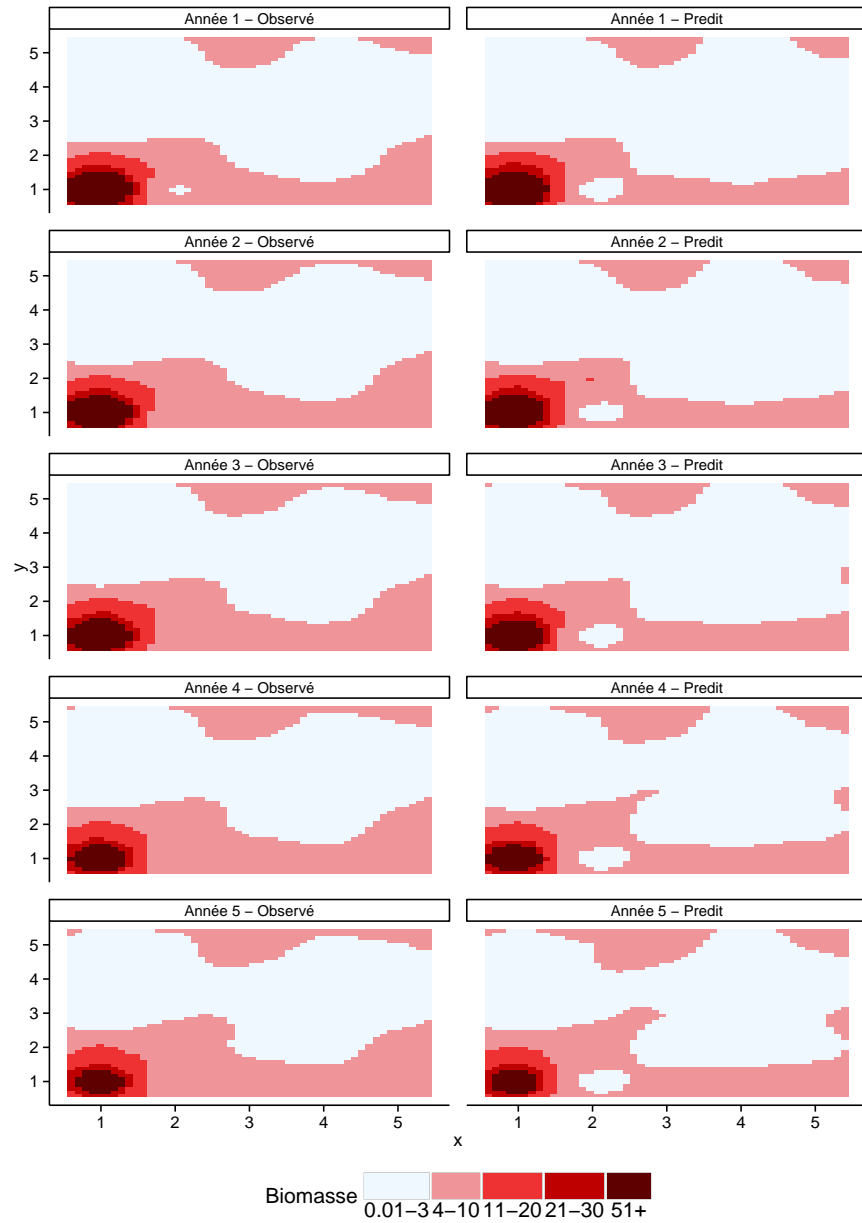
FIGURE 5.4 : Champ latent simulé et champ latent estimé sur l'ensemble de la zone d'étude pour les 5 années ( a = 1 , b = 0.2 , \mu = 0.1 , \sigma_x = 2 , \phi = 0.5 , \sigma_V = 0.1 , et \delta = 0.9 ).
