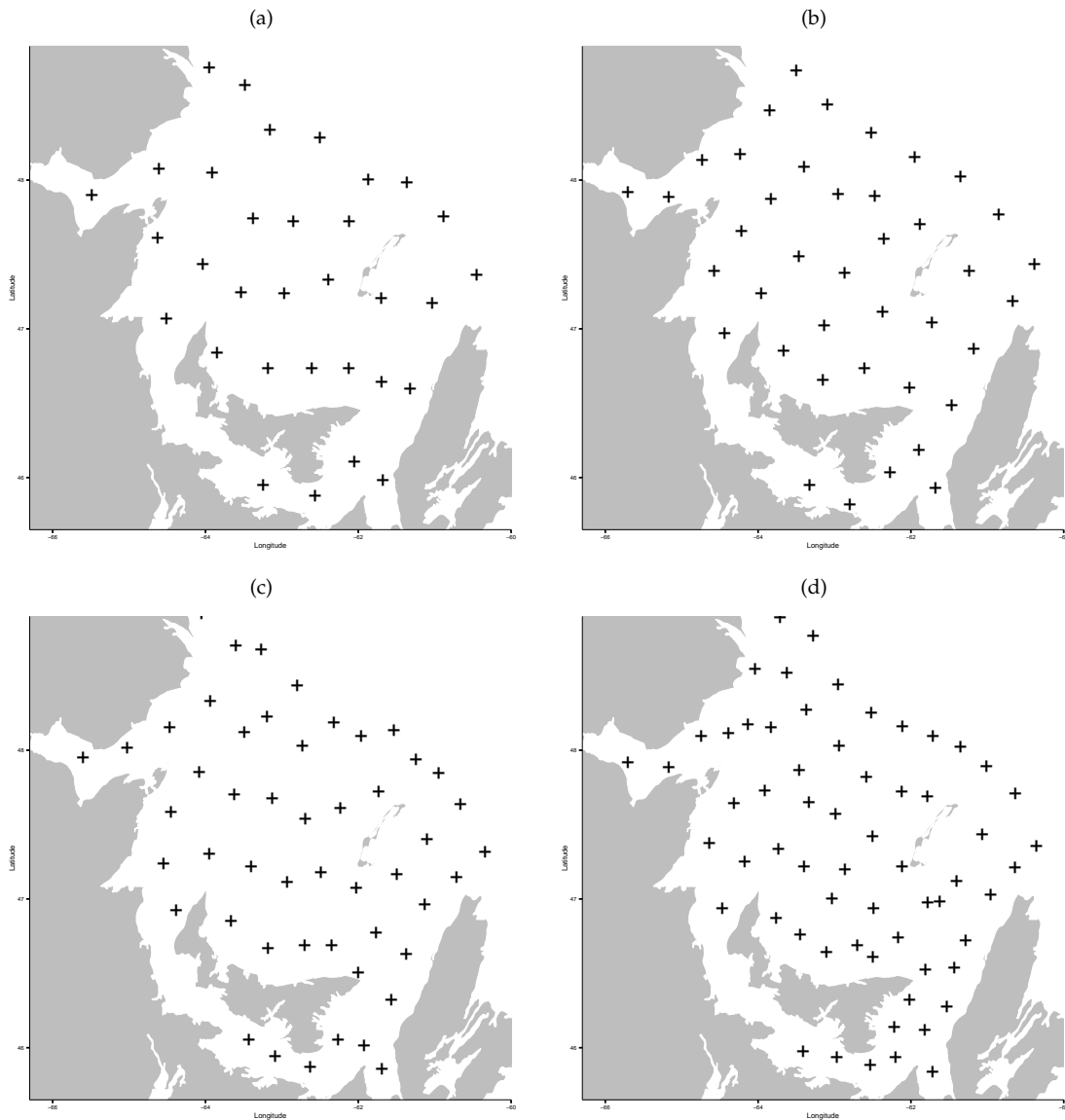
FIGURE 5.6 : Grilles irrégulières construites sur l'ensemble du sud du golfe du Saint-Laurent. (a) Grille de 32 points séparés en moyenne de 43 km . (b) Grille régulière de 41 points séparés en moyenne de 41 km . (c) Grille régulière de 50 points séparés en moyenne de 34 km . (d) Grille régulière de 63 points séparés en moyenne de 29 km .
