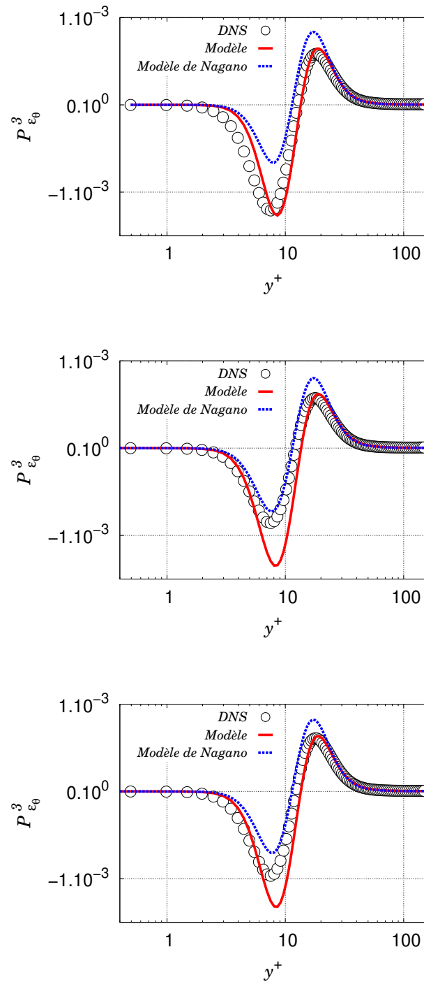
FIGURE 4.4. – Évaluation a priori du terme de production par gradient de température moyenne P_{\varepsilon_0}^1 pour un cas à température fixée (haut), à flux de chaleur imposé (milieu) et de transfert thermique conjugué (bas). Données DNS d'un cas de canal plan en convection forcée de Flageul et al. (2015, 2017).
