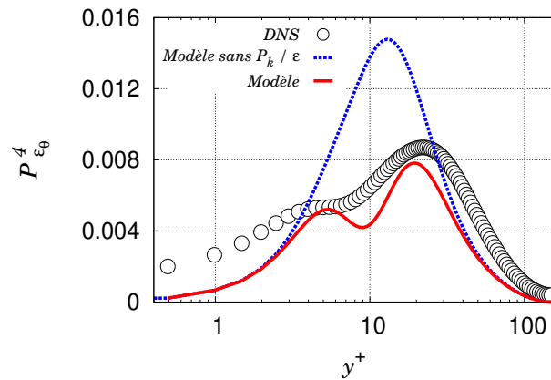
FIGURE 4.8. – Évaluation a priori du terme de production turbulente P_{\varepsilon_\theta}^A pour un cas de transfert thermique conjugué . La courbe rouge désigne le modèle complet P_{\varepsilon_\theta}^A = (1 - \alpha_\theta) P_{\varepsilon_\theta}^w + \alpha_\theta P_{\varepsilon_\theta}^h . La courbe bleue représente le même modèle sans le terme \left[ 1 - c_{\varepsilon_\theta}^{w2} (1 - \alpha_\theta) \frac{P_k}{\varepsilon} \right] dans l'expression de P_{\varepsilon_\theta}^w .
