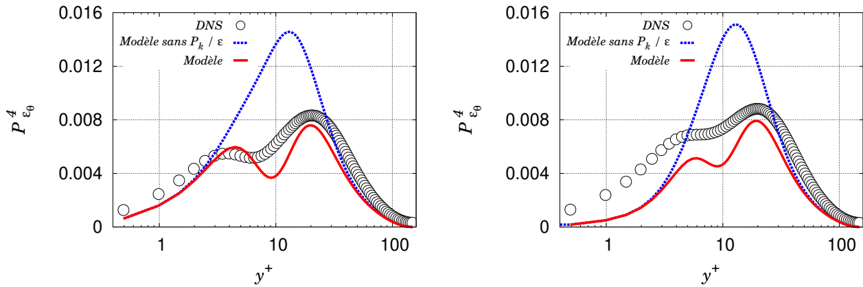
FIGURE 4.7. – Évaluation a priori du terme de production turbulente P_{\varepsilon_\theta}^A pour une température imposée à la paroi (gauche) et pour un flux de chaleur imposé (droite). La courbe rouge désigne le modèle complet P_{\varepsilon_\theta}^A = (1 - \alpha_\theta) P_{\varepsilon_\theta}^w + \alpha_\theta P_{\varepsilon_\theta}^h . La courbe bleue représente le même modèle sans le terme \left[ 1 - c_{\varepsilon_\theta}^{w2} (1 - \alpha_\theta) \frac{P_k}{\varepsilon} \right] dans l'expression de P_{\varepsilon_\theta}^w .
