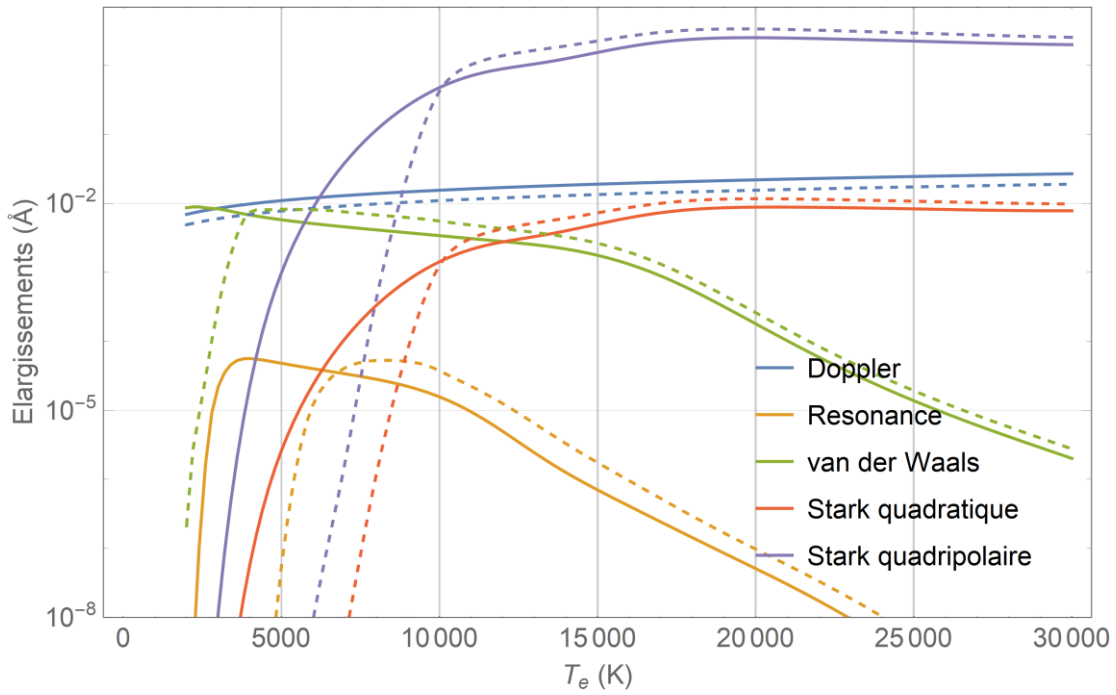
Figure 6.7 - Elargissements en fonction de la température pour la raie à 122,4 nm du soufre pour un plasma de SF 6 à 1 bar. L'ETL est en lignes pleines et \theta = 2.0 (cas 2) est en tirets.
