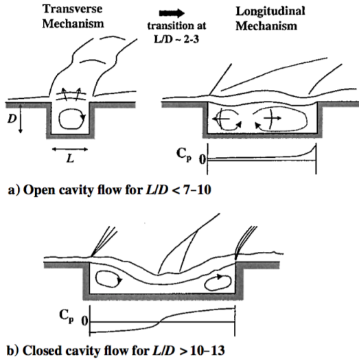
Figure 5: Schéma des cavités avec de différents rapports L/D dans un écoulement supersonique [5].
