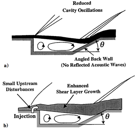
Figure 6: Techniques de stabilisation des oscillations dans la cavité : a) cavité inclinée sur la paroi arrière, b) perturbation à l'amont de la cavité [5].
