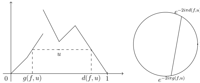
FIGURE 1.8: Une fonction càdlàg f , un point u := (s, t) de son épigraphe \mathcal{EG}(f) et la corde correspondante dans le disque \overline{\mathbb{D}} .
