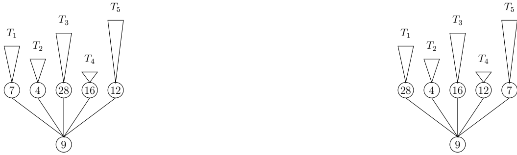
(a) Mélange d'un arbre plan étiqueté pour K = 3 : On effectue l'opération 1.
