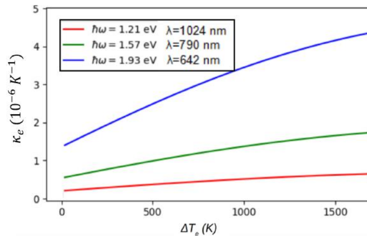
FIGURE II.15 – Coefficient de thermorélectance pour plusieurs écarts de température électronique par rapport à la température ambiante T_e = 300 K, calculée à partir des transitions intra-bande induites par collisions électron-photon-électron Umklapp. Ces résultats ont été obtenus pour une température des phonons maintenue à la température ambiante.
