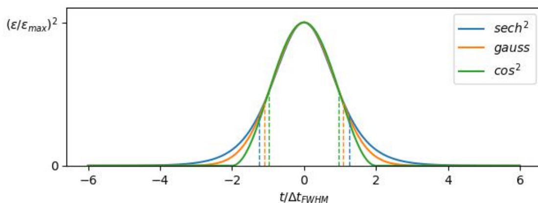
FIGURE E.1 – Différents types d'enveloppes temporelles normalisées pour le carré du champ électrique. On présente une enveloppe en \text{sech}^2(t) , une enveloppe gaussienne \exp(-\frac{1}{2}(\frac{t}{\Delta t_{FWHM}}\sqrt{2\ln(2)})^2) et une enveloppe en \cos^2 : \frac{1+\cos(\pi t/\Delta t_{FWHM})}{2}\Pi(2t/\Delta t_{FWHM}) . Les segments délimitent la zone centrale de l'enveloppe qui contient 80% de sa surface.
