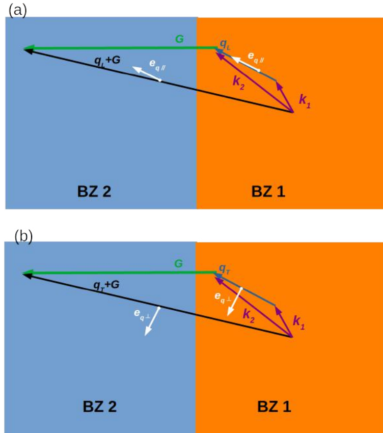
FIGURE II.4 – Collision électron-phonon Umklapp. On représente ici dans l'espace des phases les états initial \mathbf{k}_1 et final \mathbf{k}_2 (flèches violettes) d'un électron qui effectue une collision avec un phonon de vecteur d'onde \mathbf{q} (flèche bleue). On représente aussi en bleu le vecteur polarisation \mathbf{e}_q du phonon qui donne la direction dans laquelle oscillent les ions. (a) présente deux voies de diffusion par un phonon longitudinal qui permettent une transition de l'état \mathbf{k}_1 vers \mathbf{k}_2 . Dans les deux voies (directe ou Umklapp), le vecteur d'onde échangé ( \mathbf{q} ou \mathbf{q} + \mathbf{G} ) a une composante non nulle dans la direction portant la polarisation. (b) présente aussi deux voies de diffusion par un phonon transverse, mais on voit ici qu'il n'y a pas de composante du vecteur d'onde dans la direction de polarisation pour la transition directe. En revanche, dans la diffusion Umklapp, le moment cristallin échangé vaut \mathbf{G} + \mathbf{q}_T , il peut alors y avoir une composante longitudinale avec le vecteur polarisation : (\mathbf{G} + \mathbf{q}_T) \cdot \mathbf{e}_q = \mathbf{G} \cdot \mathbf{e}_q
