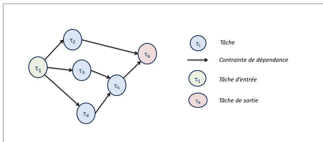
FIGURE 2.2 – Exemple d'un DAG.
