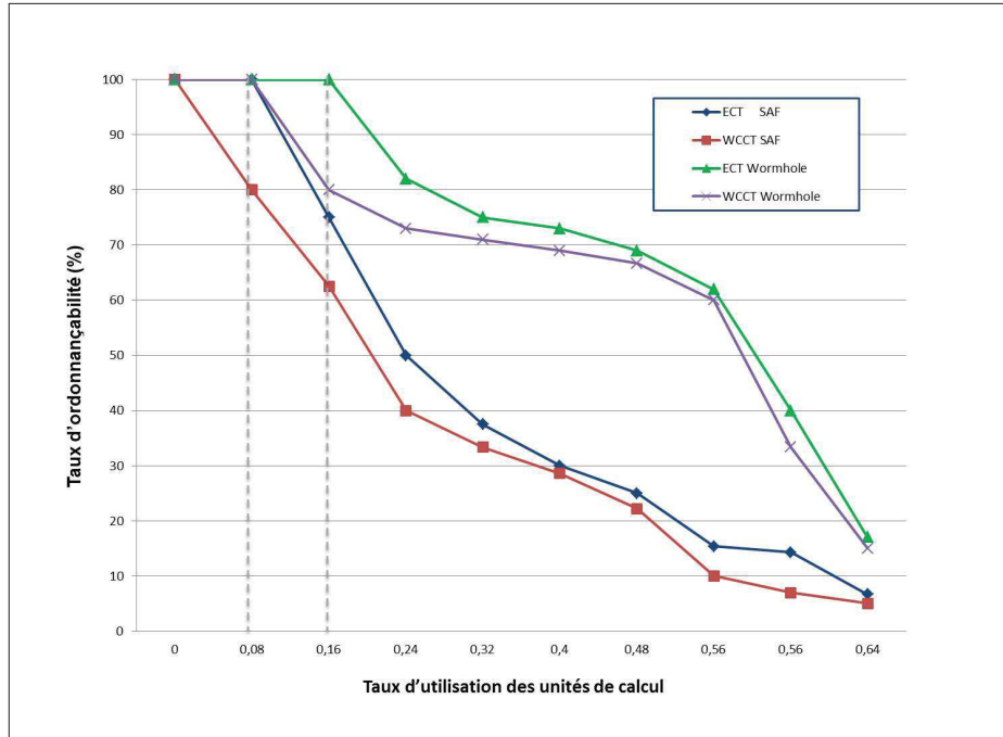
FIGURE 7.13 – Taux d'ordonnançabilité pour le modèle One-To-One
