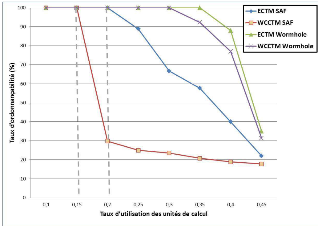
FIGURE 7.12 – Taux d'ordonnancement pour le modèle All-To-One
