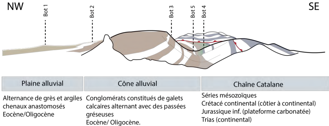
Figure 80 Carte d'après la carte de Terra Alta au 1/50000 (disponible sur le site : icgc.cat), log magnéto-stratigraphique d'après Jones et al., (2004) et panorama de la chaîne côtière catalane.
