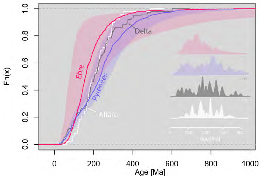
Figure 105 CC (Courbe cumulative) et KDE (kernel density plot) des âges ZFT obtenus dans les sédiments pyrénéens (Vacherat et al., 2017; Whitchurch et al., 2011) et les sédiments du bassin de l'Èbre (cette étude) comparés aux distributions cumulatives obtenues dans les sédiments actuels en amont et en aval du fleuve de l'Èbre. Les erreurs sur les âges ZFT sont représentées par des
