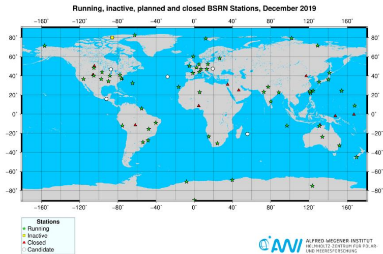
Figure 19: stations de mesure du réseau BSRN
