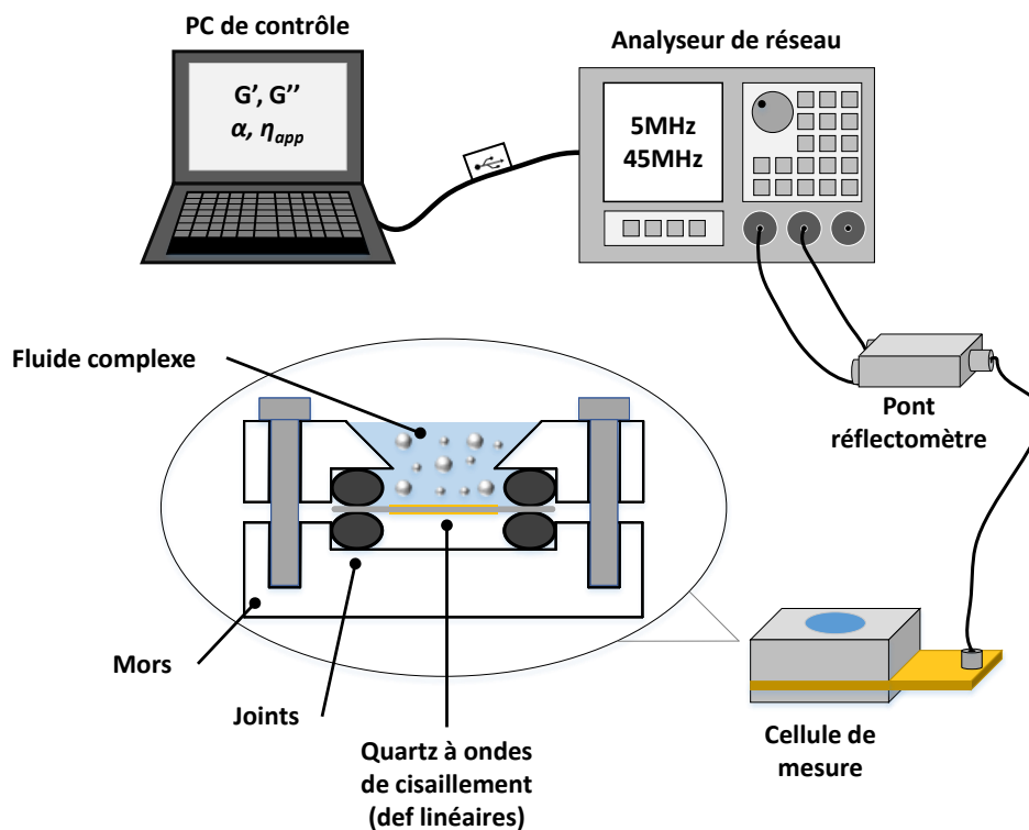
Figure LXXXIII Chaîne de mesure microrhéologique pour fluides complexes
