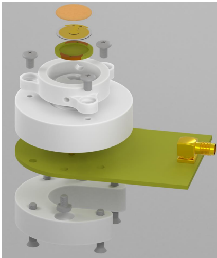
Figure LXIV Vue éclatée du modèle numérique de la cellule de mesure ex vivo
