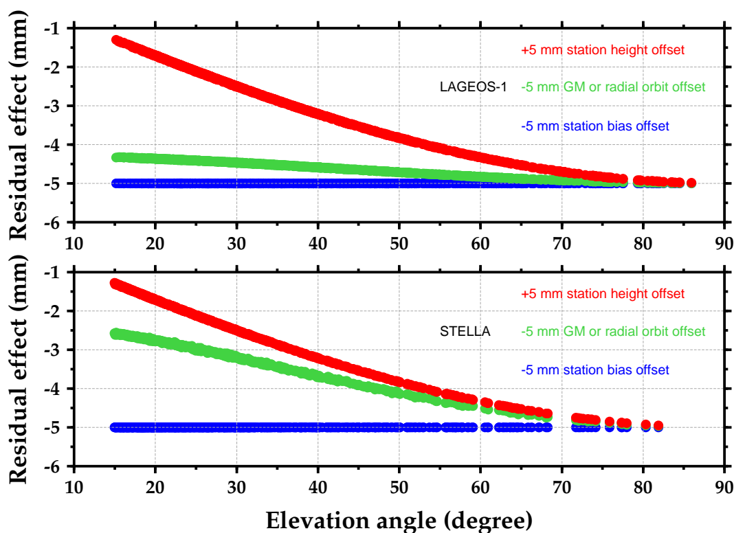
FIGURE 2.3: Impact sur les résidus laser d'un offset de biais de +5 mm (bleu), d'un offset de hauteur de -5 mm (rouge), et d'un offset de GM équivalent à un offset d'orbite radial de -5 mm (vert), pour les satellites LAGEOS-1 (haut) et Stella (bas). Les résidus ont été calculés pour la station laser de Yarragadee (7090), en Australie, sur le mois de juin 2007, mais ces résultats sont indépendants de la station et de la période analysée.
