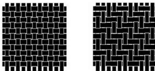
Fig. 119 : Les armures de toile 1/1 (à gauche) et de sergé 2/2 (à droite)
