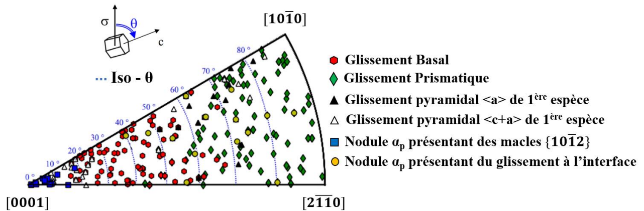
Figure IV-26 : Modes de déformation des nodules \alpha_p du Ti-6Al-4V en fonction de l'orientation cristallographique représentée sur une figure de pôles inverse codée selon la direction de sollicitation pour un chargement en dwell-fatigue 120s à \sigma_{\max} = 0,94 \times R_p^{0,2\%} jusqu'à 2,5% de déformation plastique.
