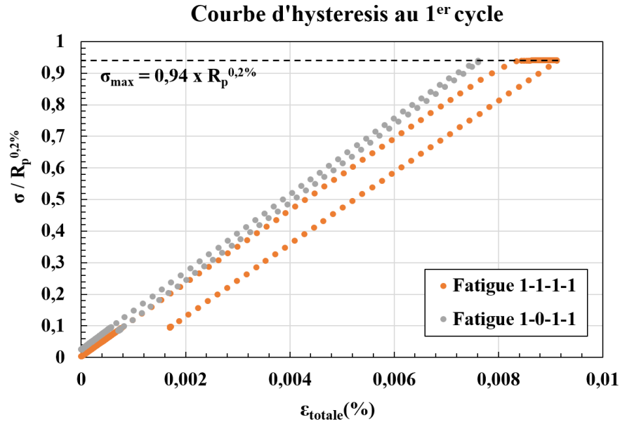
Figure III-27 : Contrainte en fonction de la déformation totale durant le premier cycle d'une sollicitation cyclique avec un temps de maintien de 1s (1-1-1-1) ou aucun temps de maintien (1-0-1-1).
