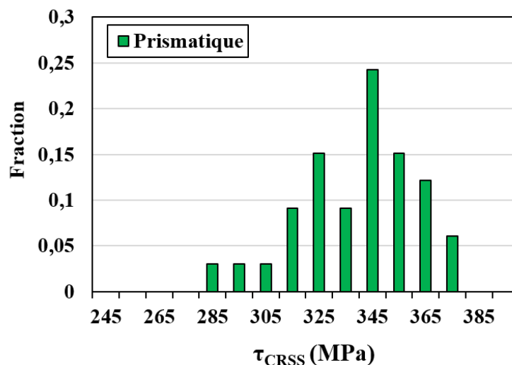
Figure III-12 : Répartition en nombre et par classe de 10 MPa des \tau_{CRSS} pour les systèmes de glissement prismatique.
