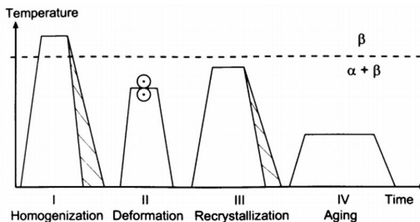
Figure I-7: Schéma de la procédure de traitement thermomécanique pour les alliages de titane \alpha + \beta . Les étapes II et III correspondent à l'obtention d'une microstructure bimodale (Lütjering and Williams, 2007)
