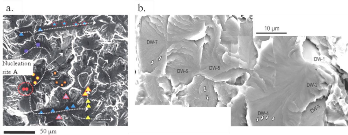
Figure I-39 : Détermination de la nature des facettes internes (amorçage ou propagation) selon les études de a. (Uta et al., 2009) et b. (Pilchak and Williams, 2011). b. DW-1 correspond à la facette d'amorçage
