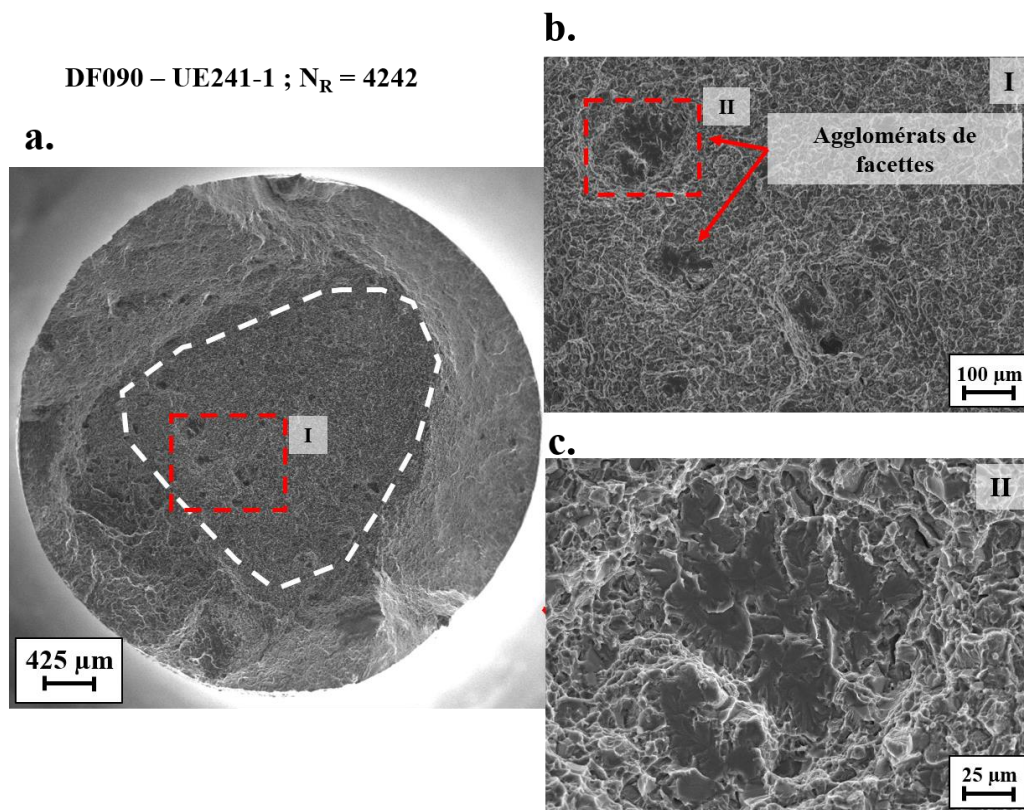
Figure III-25 : Micrographies MEB à différents grossissements du faciès de rupture de l'éprouvette UE241-1 obtenue par dwell-fatigue à \sigma_{\max} = 0,90 \times R_p^{0,2\%} .
