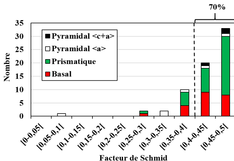
Figure III-7 : Histogramme de répartition en nombre des systèmes de glissement prismatique, basal, pyramidal \langle a \rangle et \langle c+a \rangle en fonction du facteur de Schmid
