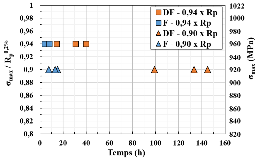
Figure III-20 : Temps à rupture en fonction du niveau de contrainte maximale appliqué pour les essais de fatigue (F) et de dwell-fatigue 120s (DF).
