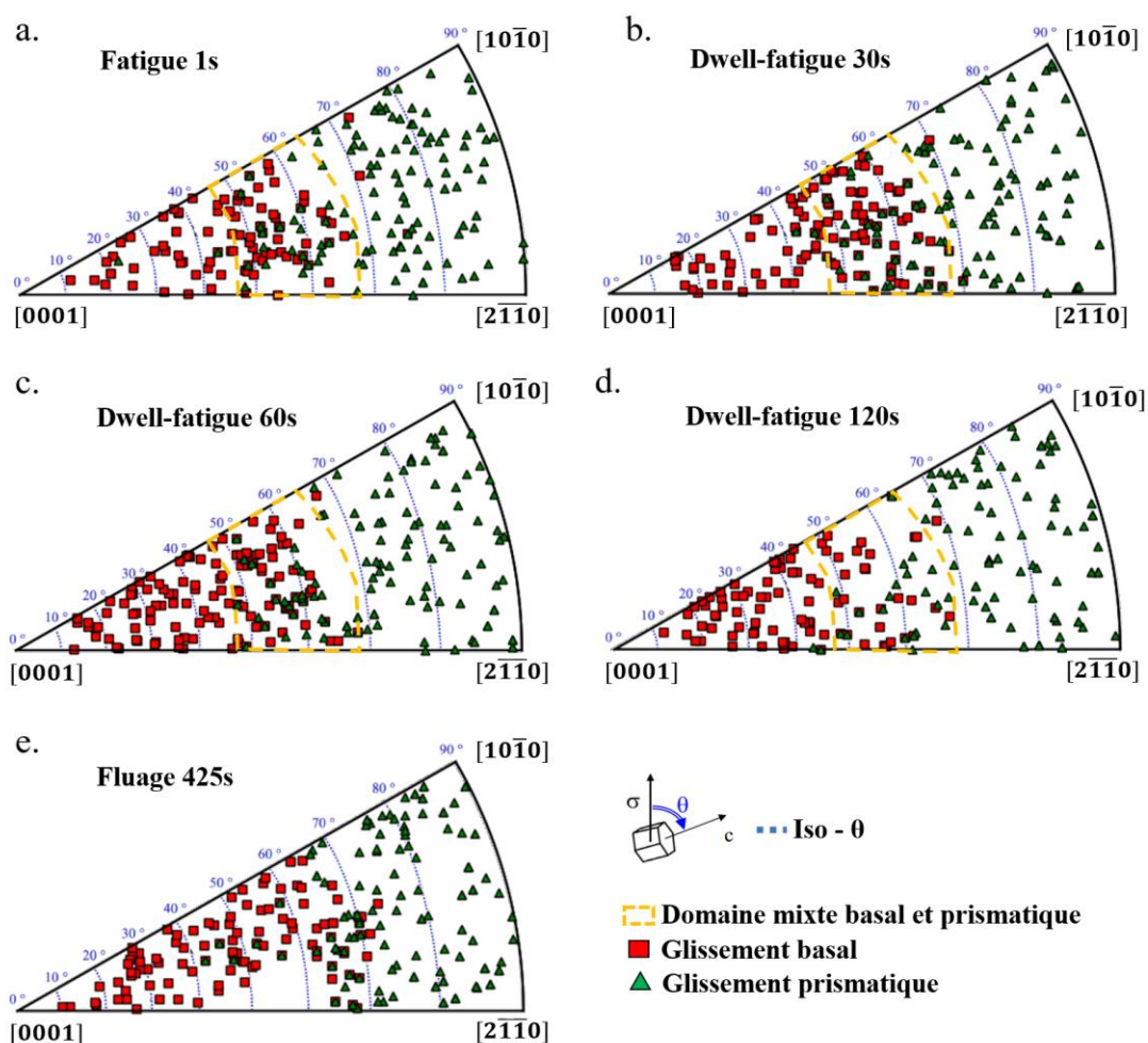
Figure A-1 : Orientations cristallographiques des nœuds \alpha_p présentant des traces de glissement basal et prismatique représentées sur une figure de pôles inverse codée selon la direction de sollicitation après une déformation plastique de 2,5% en a. fatigue, dwell-fatigue b. 30s, c. 60s, d. 120s et e. fluage à \sigma_{\max} = 0,94 \times R_p^{0,2\%} .
