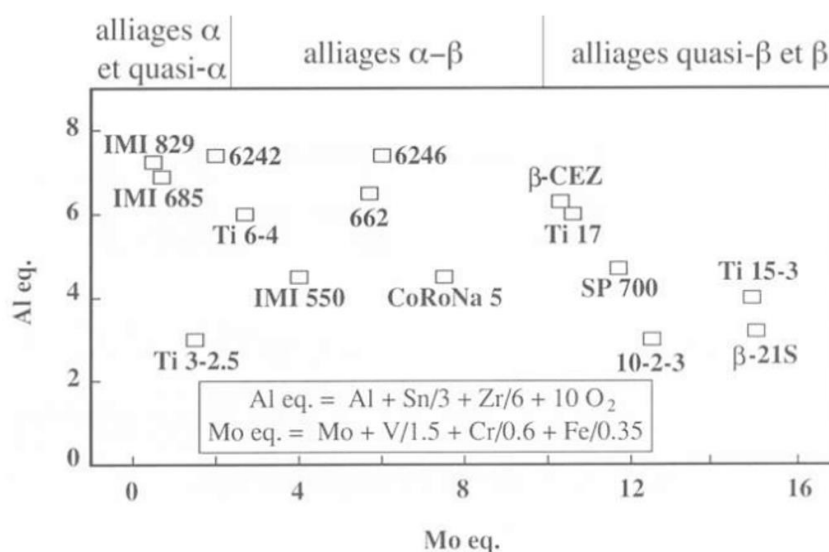
Figure I-6 : Classification d'alliages de titane usuels en fonction du pourcentage équivalent en poids d'aluminium et de molybdène (Jousset, 2008)
