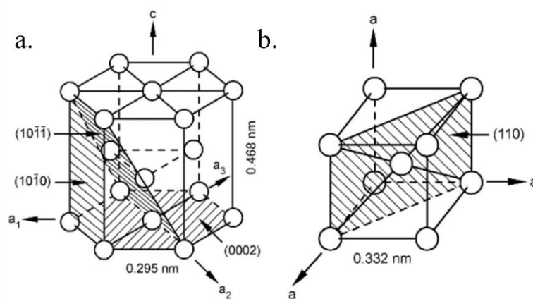
Figure I-1 : Structure cristallographique : a. hexagonale compacte de la phase \alpha et b. cubique centrée de la phase \beta (Lunt, 2014).
