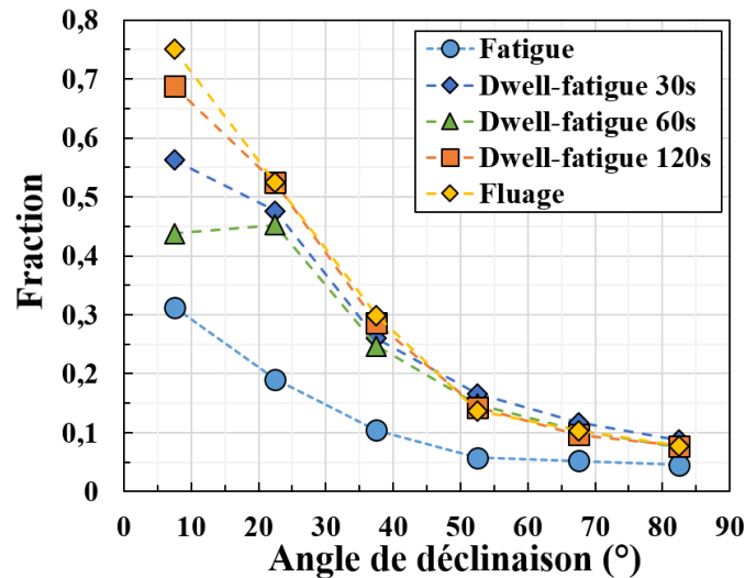
Figure IV-14 : Fractions des systèmes pyramidal \langle c+a \rangle actifs après 2,5% de déformation plastique en fatigue, dwell-fatigue 30s, 60s, 120s et fluage à \sigma_{\max} = 0,94 \times R_p^{0,2\%} en fonction de l'angle de déclinaison des nodules au sein desquels ils ont été identifiés par intervalle de 15^\circ .
