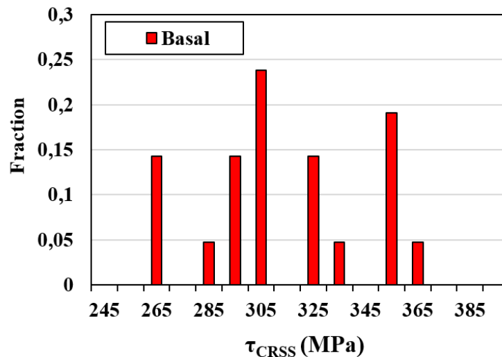
Figure III-11 : Répartition en nombre et par classe de 10 MPa des \tau_{CRSS} pour les systèmes de glissement basal.
