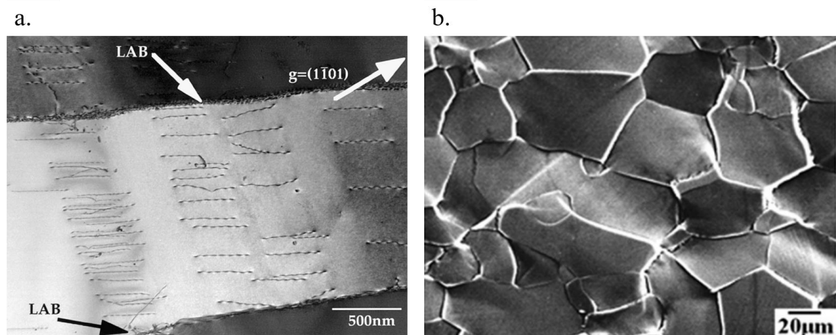
Figure I-30 : Micrographies a. MET du glissement intra-lamellaire planaire en fluage à température ambiante (Neeraj et al., 2000) pour un alliage Ti-6Al et b. MEB du glissement aux joints de grain en fluage à chaud pour un alliage Ti-6Al-4V avec une microstructure équiaxe (Li et al., 2012).
