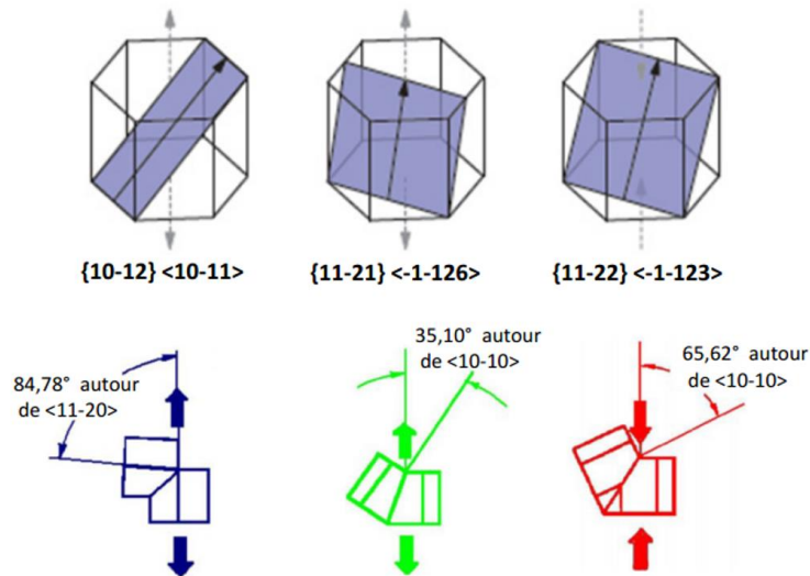
Figure I-13: Modes de maillage de la phase \alpha du titane (Barkia, 2014)
