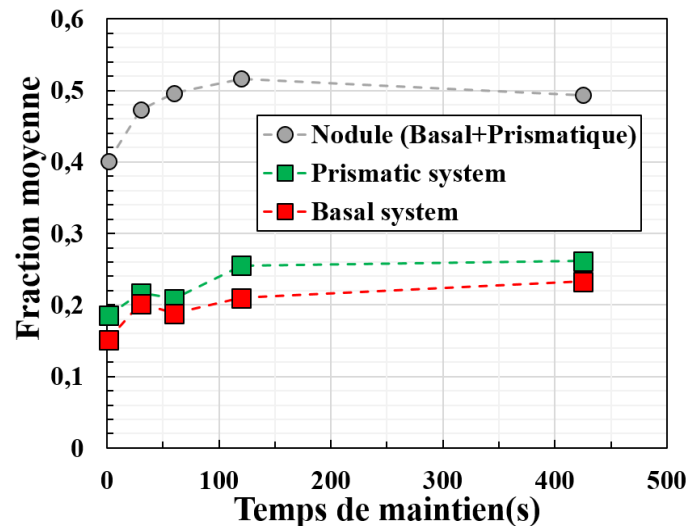
Figure IV-10 : Fractions moyenne des systèmes de glissement basal et prismatique actifs après 2,5% de déformation plastique à \sigma_{\max} = 0,94 \times R_p^{0,2\%} en fonction du temps de maintien à charge maximale appliqué en cours de cycle. (Plusieurs systèmes sont possiblement détectés dans un même nodule, c'est pourquoi les sommes des fractions sont supérieures à 1)
