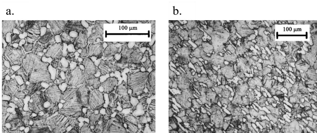
Figure I-26 : Microstructures bimodales d'un alliage IMI 834 a. « bar » et b. « disc » des travaux de Bache et al. (Bache et al., 1997a). La Figure I-24 présente les durées de vie de chacune des microstructures en fatigue et dwell-fatigue.
