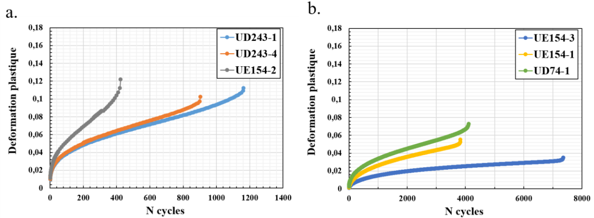
Figure III-17 : Evolution de la déformation plastique en fonction du nombre de cycles pour les essais de a. dwell-fatigue et b. fatigue réalisés à \sigma_{\max} = 0,94 \times R_p^{0,2\%}
