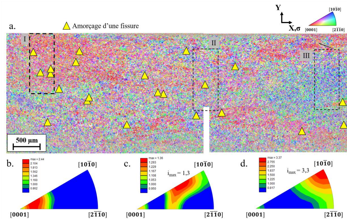
Figure V-18 : a. Cartographie des orientations cristallographiques codées selon la direction de sollicitation montrant la position des sites d'amorçage de fissure en lien avec la texture cristallographique locale pour l'éprouvette sollicitée en fatigue à 0,90 \times R_p^{0,2\%} jusqu'à 1% de déformation plastique. Textures cristallographiques des régions (b) I, (c) II et (d) III représentée sur une figure de pôle inverses.
