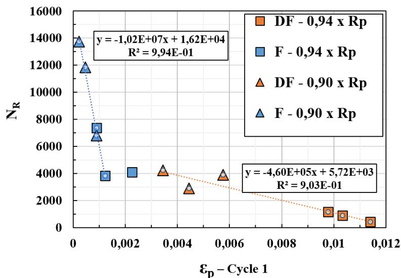
Figure III-22 : Nombre de cycles à rupture N_R en fonction de la déformation plastique après 1 cycle de chargement pour les essais de fatigue (F) et de dwell-fatigue 120s (DF).
