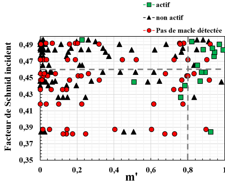
Figure IV-22 : Facteur de Schmid incident en fonction du paramètre m' associé en considérant les 6 systèmes de maclage \{10\bar{1}2\} pour chaque interaction d'une bande de glissement avec l'interface d'un nodule étudié. Les distributions et le code de couleurs associé sont équivalents à ce qui est décrit pour le graphique de la Figure IV-21.
