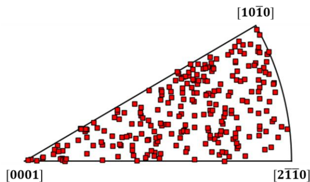
Figure III-2 : Orientations cristallographiques des nodules de phase alpha primaire contenus dans les zones d'étude sur une figure de pôle inverse codée selon la direction de sollicitation
