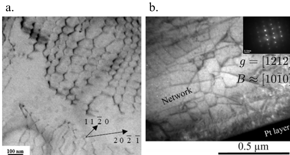
Figure V-23 : Micrographies MET montrant des réseaux de dislocations à proximité des sites d'amorçage de fissures en dwell-fatigue dans les études de a. Wang et al. et b. Tynpel et al. (Tynpel et al., 2016; Wang et al., 2007)
