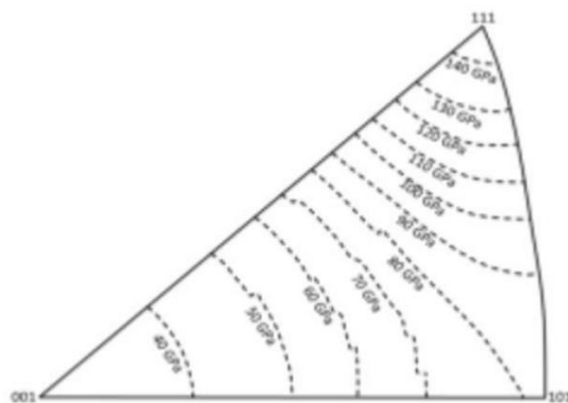
Figure I-3 : Figure de pôles inverse codée selon la direction de sollicitation avec les iso-contours du module d'Young de la phase \beta (Duval, 2014).
