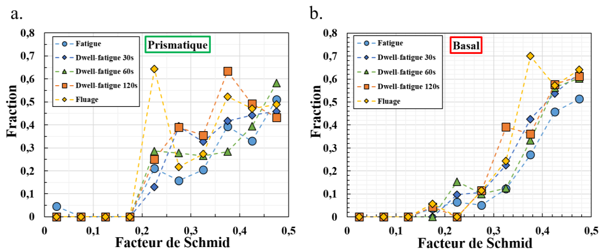
Figure IV-9 : Distribution des fractions des systèmes de glissement a. prismatiques et b. basals actifs après 2,5% de déformation plastique en fatigue, dwell-fatigue 30s, 60s, 120s et fluage à 0,94 \times R_p^{0,2\%} par intervalle de facteur de Schmid de 0,05.
