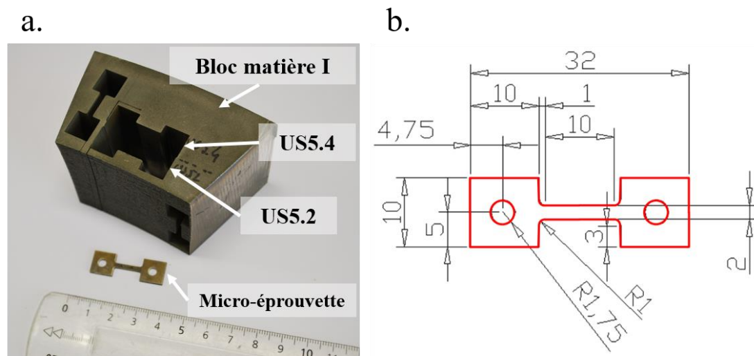
Figure II-2 : a. Bloc de matière I avec les directions de prélèvement des micro-éprouvettes et b. plan de conception d'une micro-éprouvette (dimensions en mm).
