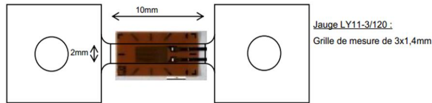
Figure II-10 : Schéma d'une micro-éprouvette avec le positionnement d'une jauge de déformation (Freiherr von Thügen, 2016).
