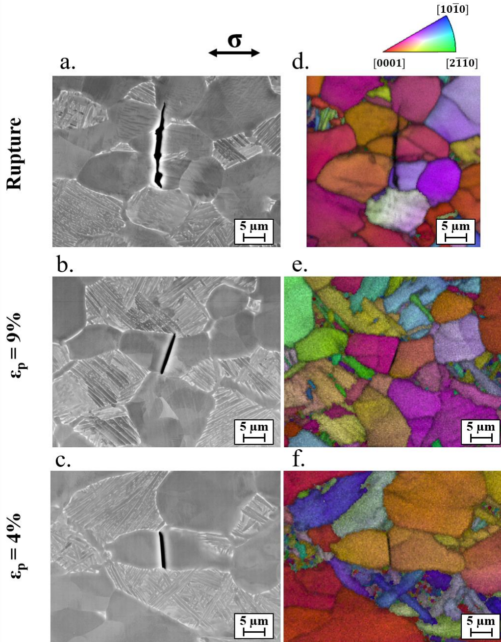
Figure V-9 : Micrographies MEB de fissures subsurfaciques détectées a. pour un chargement en dwell-fatigue 120s a. à \sigma_{\max} = 0,94 \times R_p^{0,2\%} à rupture, b. à \sigma_{\max} = 0,94 \times R_p^{0,2\%} et 9% de déformation plastique et c. \sigma_{\max} = 0,90 \times R_p^{0,2\%} et 4% de déformation plastique. Les cartographies d'orientations cristallographiques respectives sont codées selon la direction de sollicitation (d,e et f).
