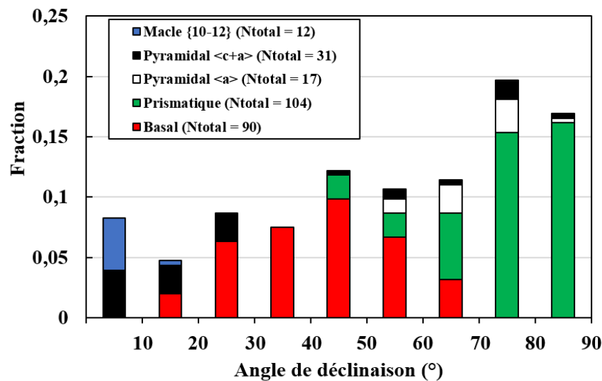
Figure IV-27 : Distribution en nombre des modes de déformation des nodules \alpha_p du Ti-6Al-4V en fonction de l'angle de déclinaison pour chargement en dwell-fatigue 120s à \sigma_{\max} = 0,94 \times R_p^{0,2\%} jusqu'à 2,5% de déformation plastique
