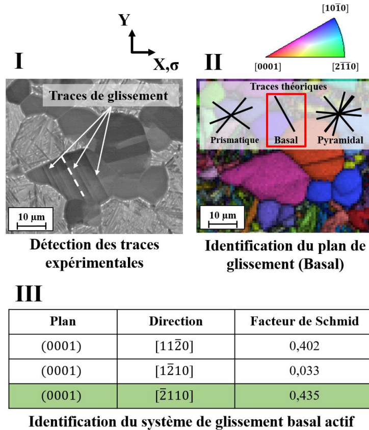
Figure II-15 : Principe de l'analyse des traces de glissement. I. Détection des traces de glissement expérimentales sur les micrographies MEB. II. Calcul des traces théoriques des plans de glissement du titane et identification du plan de glissement actif (basal ici). III. Identification du système de glissement basal actif sur la base du Facteur de Schmid maximum.
