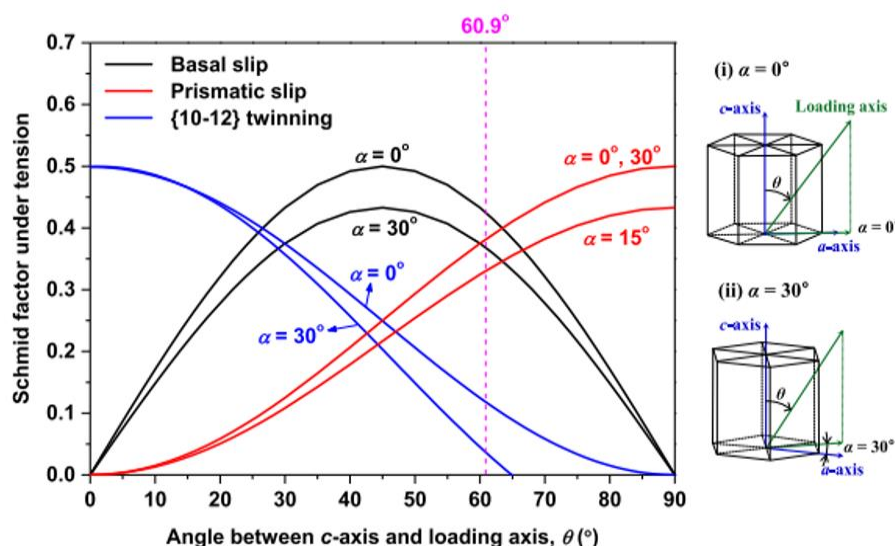
Figure I-16 : Evolution du facteur de Schmid pour le mode de maillage \{10\bar{1}2\} en fonction de l'angle de déclinaison pour l'alliage Mg-1Gd (Lee et al., 2019).
