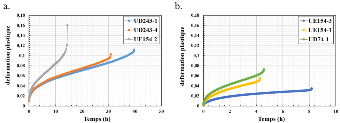
Figure III-18 : Evolution de la déformation plastique en fonction du temps pour les essais de a. dwell-fatigue et b. fatigue réalisés à \sigma_{\max} = 0,94 \times R_p^{0,2\%}
