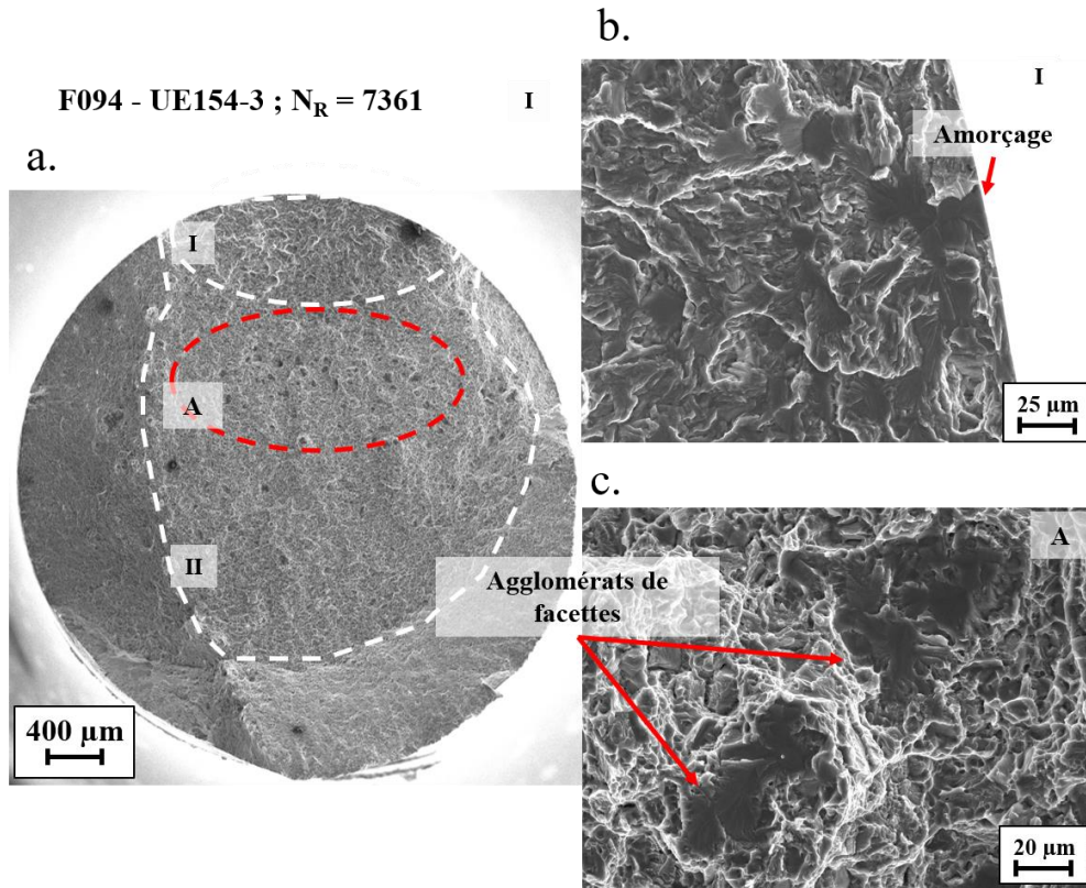
Figure III-24 : Micrographies MEB à différents grossissements du faciès de rupture de l'éprouvette UE154-3 sollicitée en fatigue à \sigma_{\max} = 0,94 \times R_p^{0,2\%} .
