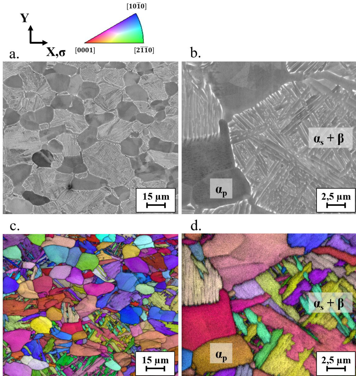
Figure II-1 : Micrographies MEB à différents grossissements et cartographies d'orientations cristallologiques (c, d) selon la direction de sollicitation (X) de la microstructure bimodale du lot de matière I.
