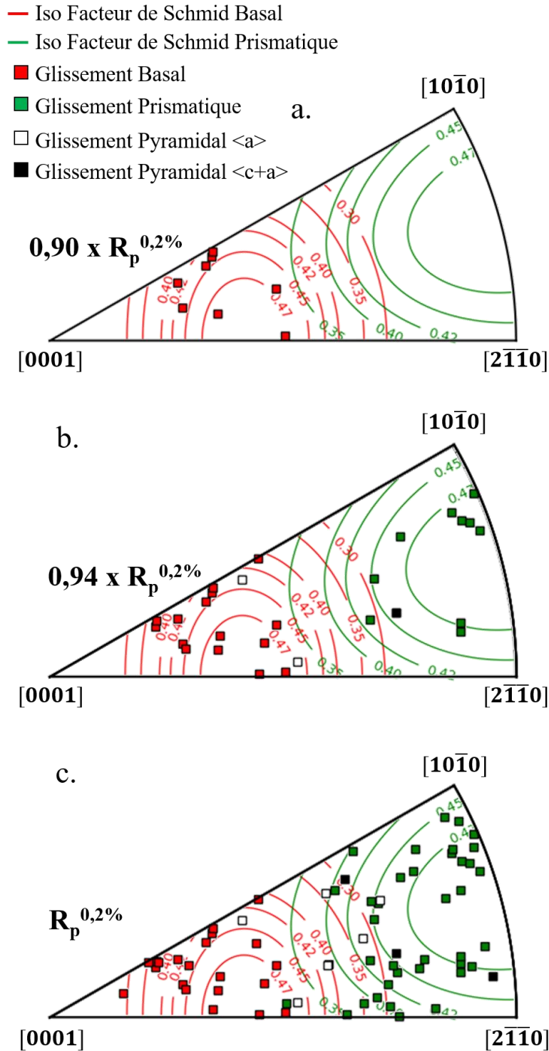
Figure III-13 : Orientations cristallographiques des nodules présentant des lignes de glissement basal, prismatique, pyramidal \langle a \rangle et \langle c+a \rangle aux niveaux de contraintes a. \sigma = 0,90 \times R_p^{0,2\%} , b. \sigma = 0,94 \times R_p^{0,2\%} et c. \sigma = R_p^{0,2\%} . Les figures de pôles inverses sont codées selon la direction de sollicitation.
