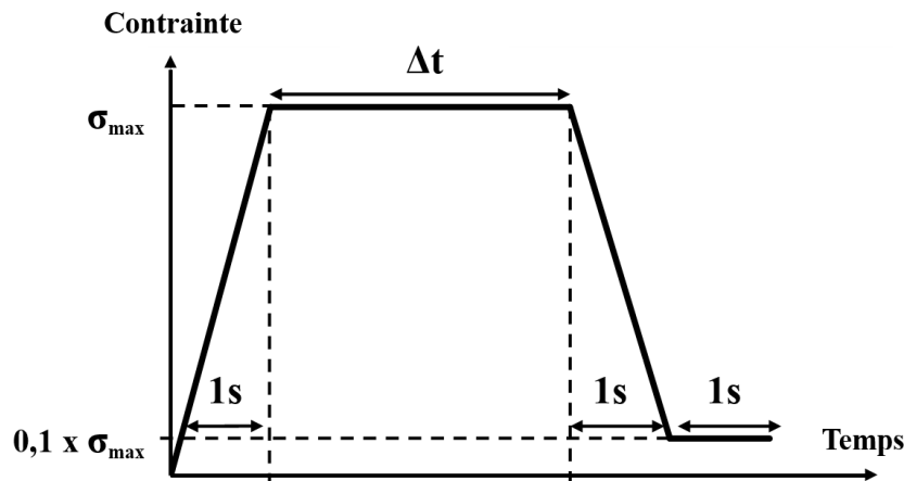
Figure II-12 : Cycle de chargement imposé pendant 1 cycle pour les essais de fatigue et dwell-fatigue
