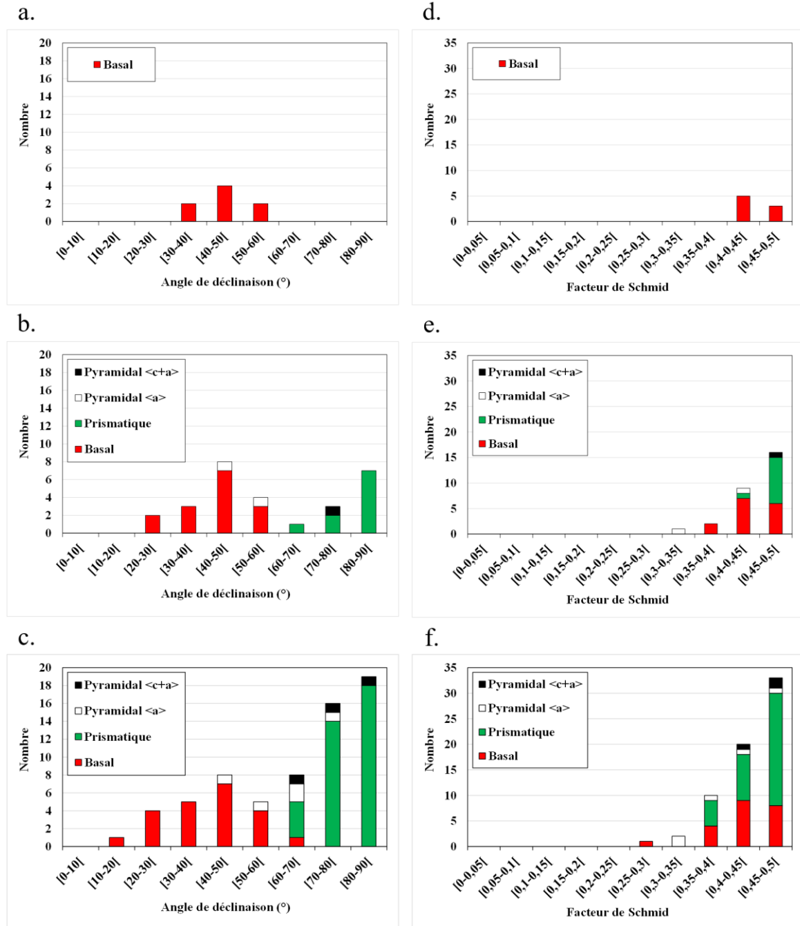
Figure III-14 : Distribution des systèmes de glissement actifs en fonction de l'angle de déclinaison à a. \sigma = 0,90 \times R_p^{0,2\%} , b. \sigma = 0,94 \times R_p^{0,2\%} et c. \sigma = R_p^{0,2\%} . Distribution des systèmes de glissement actifs en fonction du facteur de Schmid à d. \sigma = 0,90 \times R_p^{0,2\%} , e. \sigma = 0,94 \times R_p^{0,2\%} et f. \sigma = R_p^{0,2\%}
