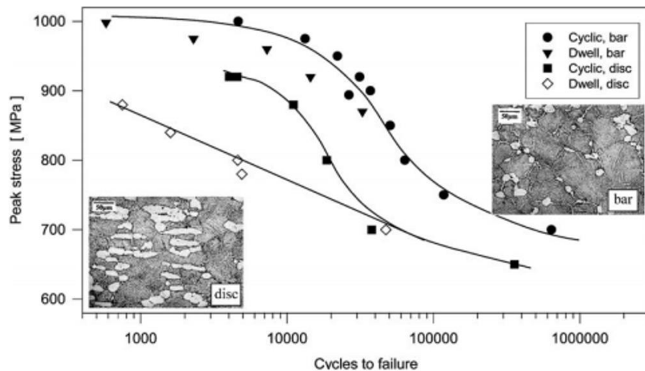
Figure I-24 : Nombre de cycles à rupture en fonction du niveau de contrainte maximale appliqué en fatigue et dwell-fatigue pour deux microstructures bimodales d'un alliage Timetal 834 (Bache et al., 1997a)
