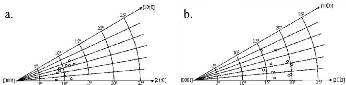
Figure I-38 : Orientations cristallographiques des facettes subsurface de dwell-fatigue pour un alliage Ti-6242 représentées sur une figure de pôles inverse codée selon a. la normale au plan de quasi-clivage et b. selon la direction de sollicitation (Sinha et al., 2007)
