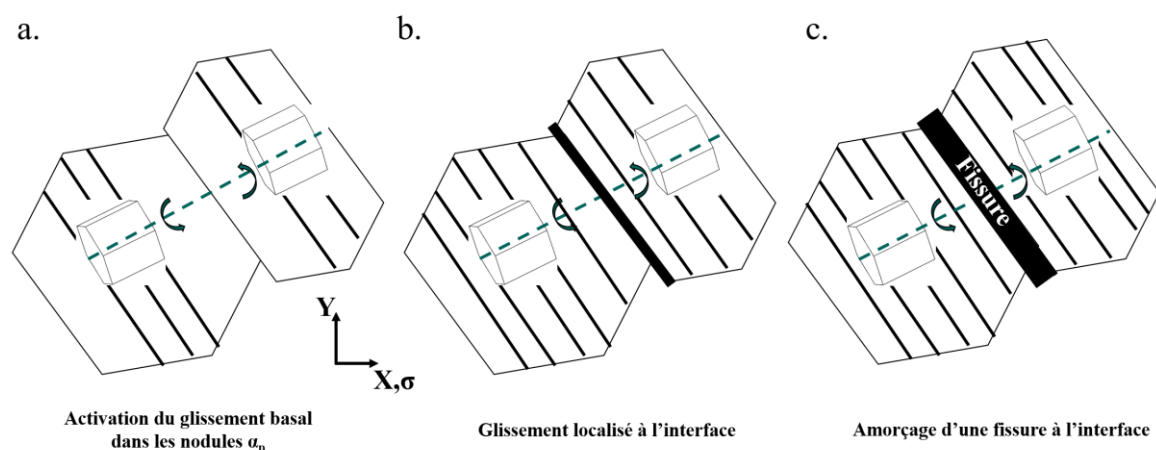
Figure V-24 : Représentation schématique des étapes conduisant à l'amorçage d'une fissure pour une sollicitation en fatigue et dwell-fatigue, en surface et dans le volume. a. Paire de nodules favorablement orientés pour le glissement basal avec un joint de twist (0001). b. Multiplication et intensification des bandes de glissement basal conduisant au glissement de l'interface. c. Amorçage d'une fissure suite à la localisation de la déformation plastique.
