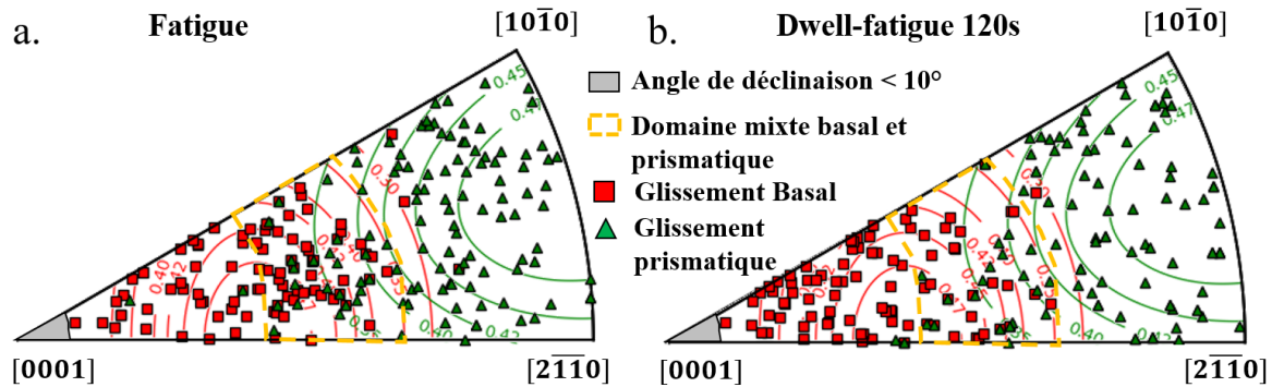
Figure IV-8 : Orientations cristallographiques des nodules \alpha_p présentant des traces de glissement basal et prismatique représentées sur une figure de pôles inverse codée selon la direction de sollicitation après une déformation plastique de 2,5% en a. fatigue et b. dwell-fatigue 120s à \sigma_{\max} = 0,94 \times R_p^{0,2\%} .
