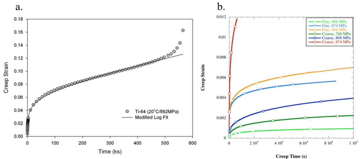
Figure I-29 : Courbes de fluage pour un alliage Ti-6Al-4V avec une microstructure a. bimodale (Harrison et al., 2013) et b. lamellaire à différents niveaux de contrainte (Brandes, 2008)
