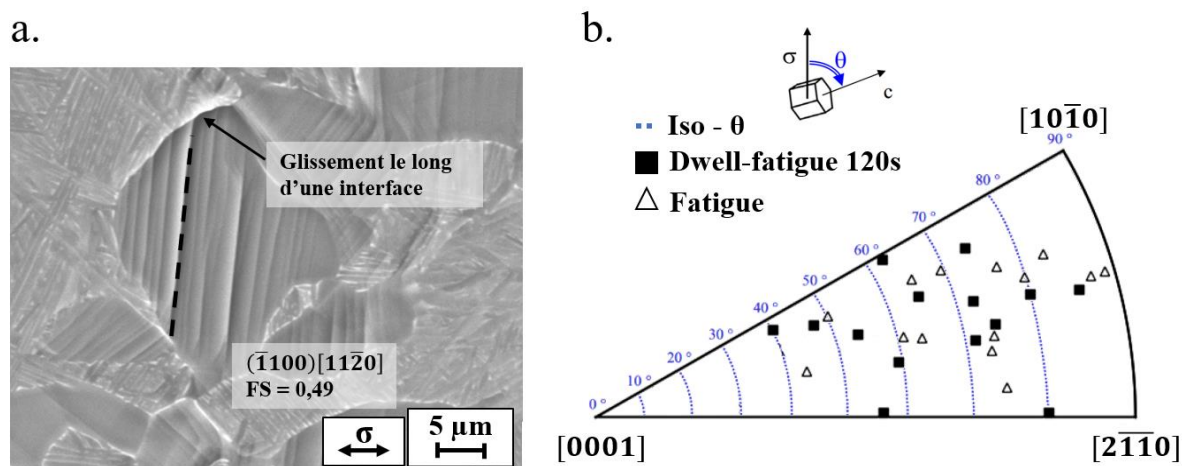
Figure IV-15 : a. Micrographie MEB montrant le glissement le long d'une interface entre un nodule \alpha_p et des colonies lamellaires stimulée par une bande de glissement présente dans le nodule \alpha_p . b. Représentations des orientations cristallographiques sur une figure de pôles inverse codée selon la direction de sollicitation des nodules \alpha_p associés à du glissement le long de l'interface en fatigue et dwell-fatigue 120s après 2,5% de déformation plastique à 0,94 \times R_p^{0,2\%} .
