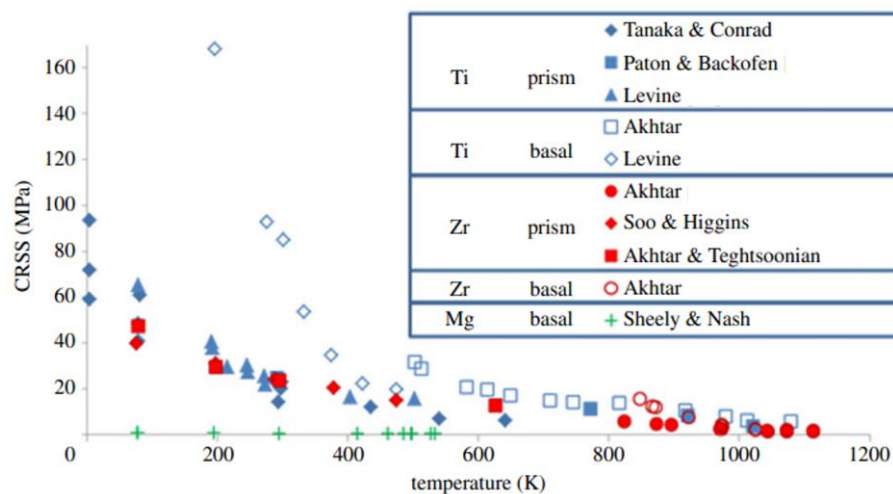
Figure I-17 : Evolution des \tau_{CRSS} du glissement basal et prismatique en fonction de la température pour des monocristaux de titane, de magnésium et de zirconium \alpha (Britton et al., 2015).
