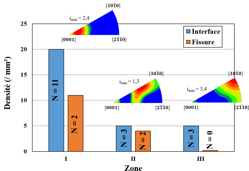
Figure V-19 : Densité de configurations microstructurales, dénommées paires de nodules \langle c \rangle , critiques pour l'amorçage et de fissures en fonction de la texture cristallographique locale.
