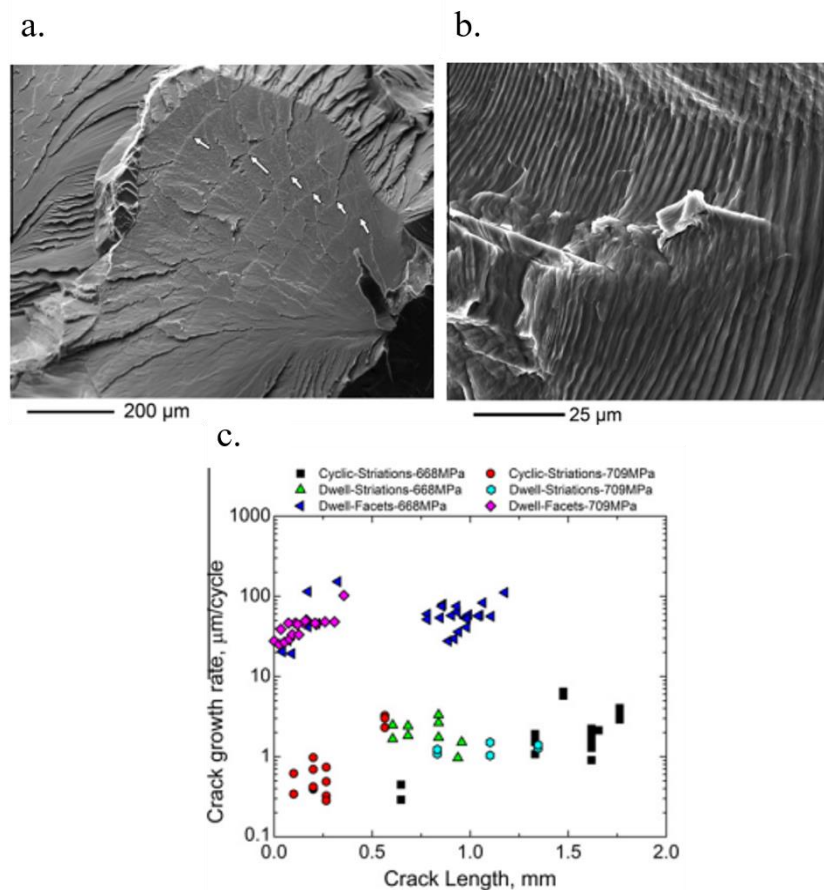
Figure I-42 : Exemples de faciès de rupture associés à une propagation de fissure conduisant à la formation a. de facettes et b. de stries de fatigue avec c. les vitesses de propagation correspondantes (Pilchak, 2013)
