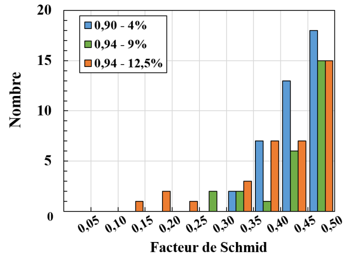
Figure V-12 : Distribution en nombre par intervalle de 0,05 des facteurs de Schmid maximum pour le glissement basal de part et d'autre des fissures subsurfaciques détectées pour des chargements en dwell-fatigue 120s à 0,90 \times R_p^{0,2\%} interrompu à 4% de déformation plastique ainsi qu'à 0,94 \times R_p^{0,2\%} interrompus à 9% et 12,5% de déformation plastique.
