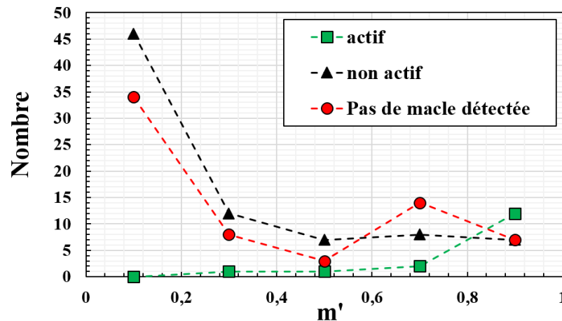
Figure IV-21 : Distribution en nombre des valeurs de m' pour les 6 systèmes de maclages \{10\bar{1}2\} en fonction pour chaque interaction d'une bande de glissement à l'interface d'un nodule avec un angle de déclinaison inférieur à 30^\circ .
