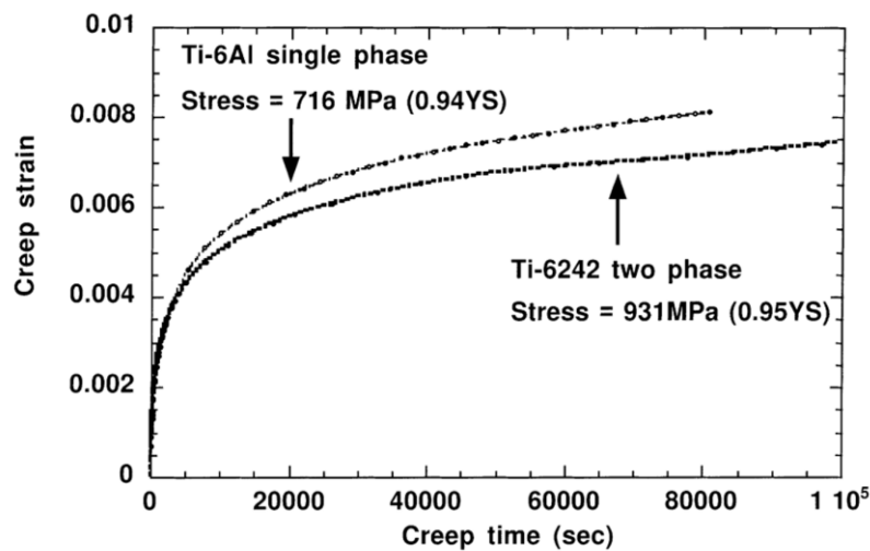
Figure I-31 : Courbes de fluage pour un alliage Ti-6Al polycristallin à un niveau de contrainte de 716 MPa et d'un alliage Ti-6242 à une contrainte de 931 MPa (Neeraj et al., 2000)
