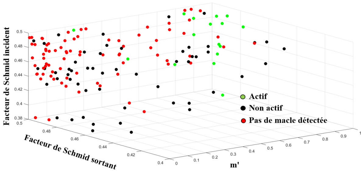
Figure IV-24 : Cartographie en trois dimensions des systèmes de maillage en fonction du facteur de Schmid incident, du facteur de Schmid sortant et du paramètre m' associé pour chaque interaction d'une bande de glissement à l'interface d'un nodule investigué. Le graphique regroupe les données présentées avec les Figure IV-22 et Figure IV-23. Les distributions et le code de couleurs associé sont équivalents à ce qui est décrit pour le graphique de la Figure IV-21.
