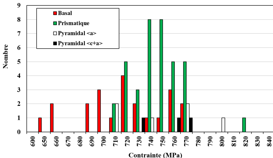
Figure III-9 : Répartition en nombre des systèmes de glissement actifs en fonction du niveau de contrainte appliqué
