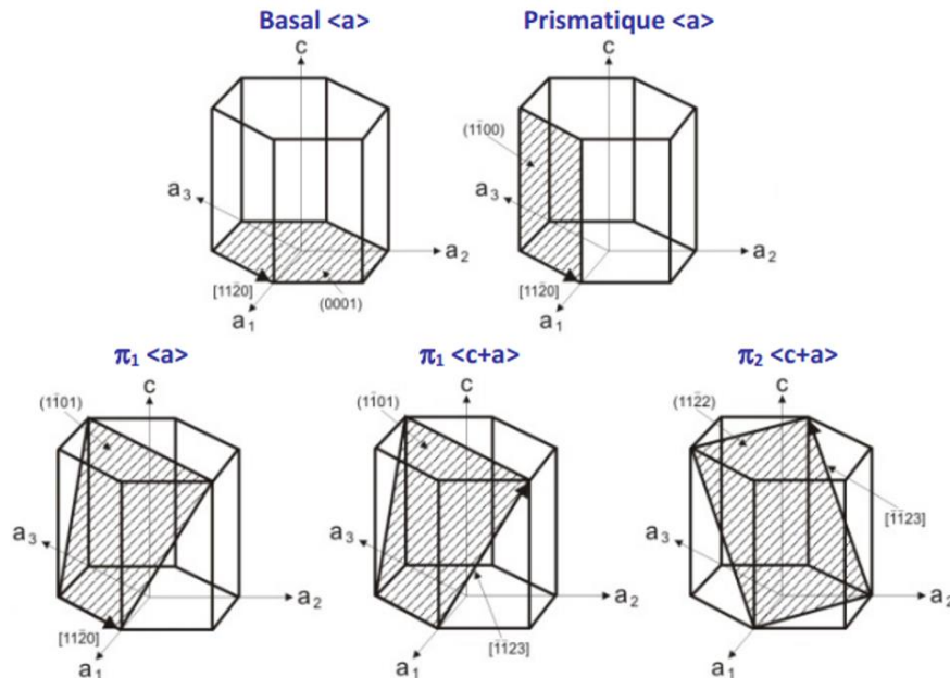
Figure I-12 : Modes de glissement de la phase \alpha du titane (Barkia, 2014)
