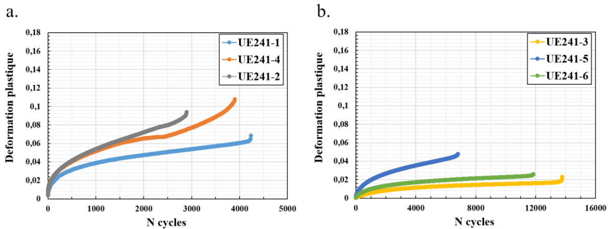
Figure III-15 : Evolution de la déformation plastique en fonction du nombre de cycles pour les essais de a. dwell-fatigue et b. fatigue réalisés à \sigma_{\max} = 0,90 \times R_p^{0,2\%}
