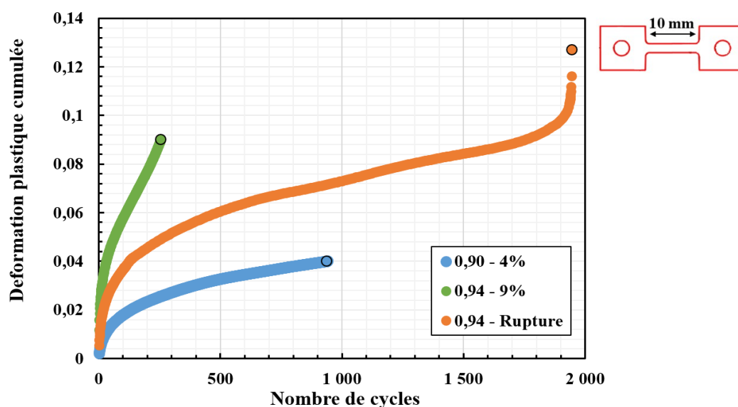
Figure V-8 : Déformation plastique en fonction du nombre de cycles pour les essais de dwell-fatigue 120s sur micro-éprouvette pour l'étude de l'amorçage des fissures subsurfaciques.
