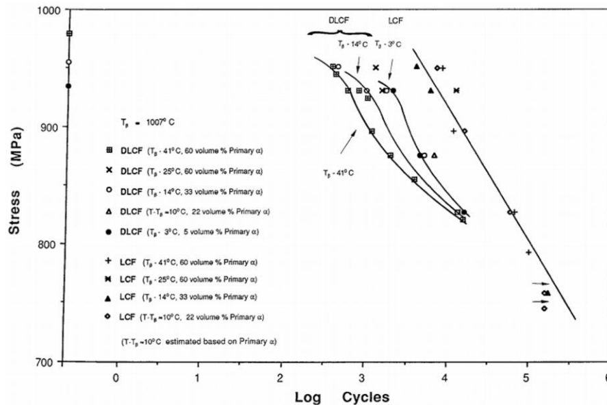
Figure I-25 : Durée de vie en fatigue et dwell fatigue de l'alliage Ti-6242 avec une microstructure bimodale et différents taux de phase \alpha_p (Kassner et al., 1999)
