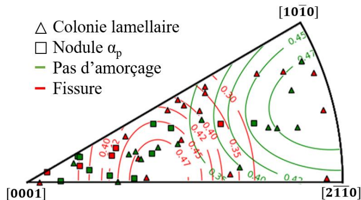
Figure V-21 : Représentation des orientations cristallographiques des éléments microstructuraux voisins des interfaces favorables à l'amorçage d'une fissure sur une figure de pôles inverse codée selon la direction de sollicitation.
