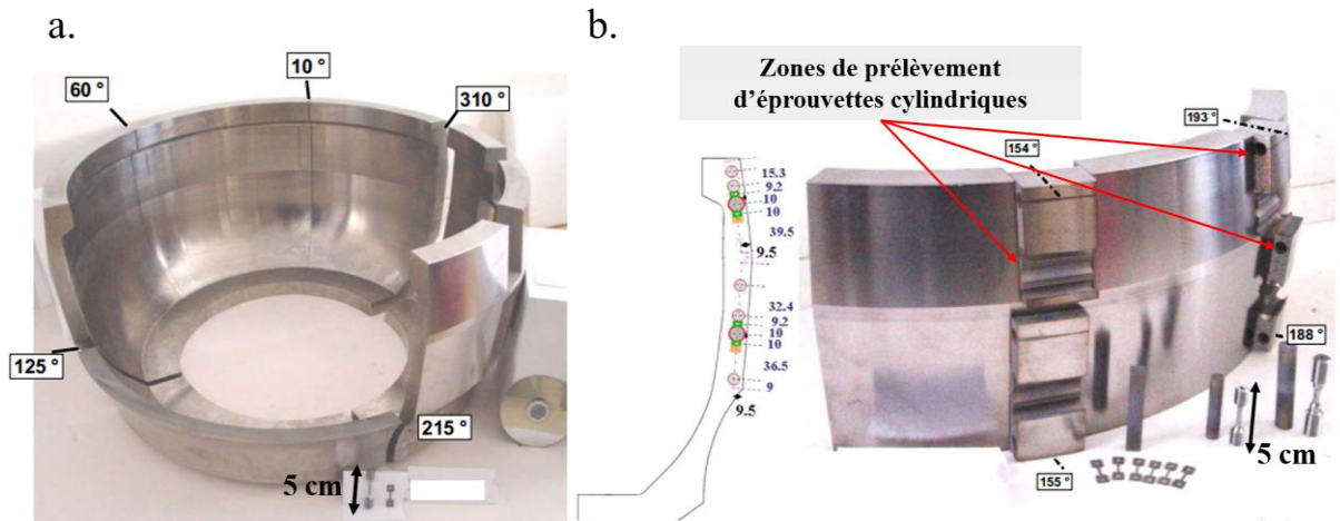
Figure II-5 : a. Vue d'ensemble du bloc de matière II et b. Prélèvement des éprouvettes cylindriques dans le haut de tambour.
