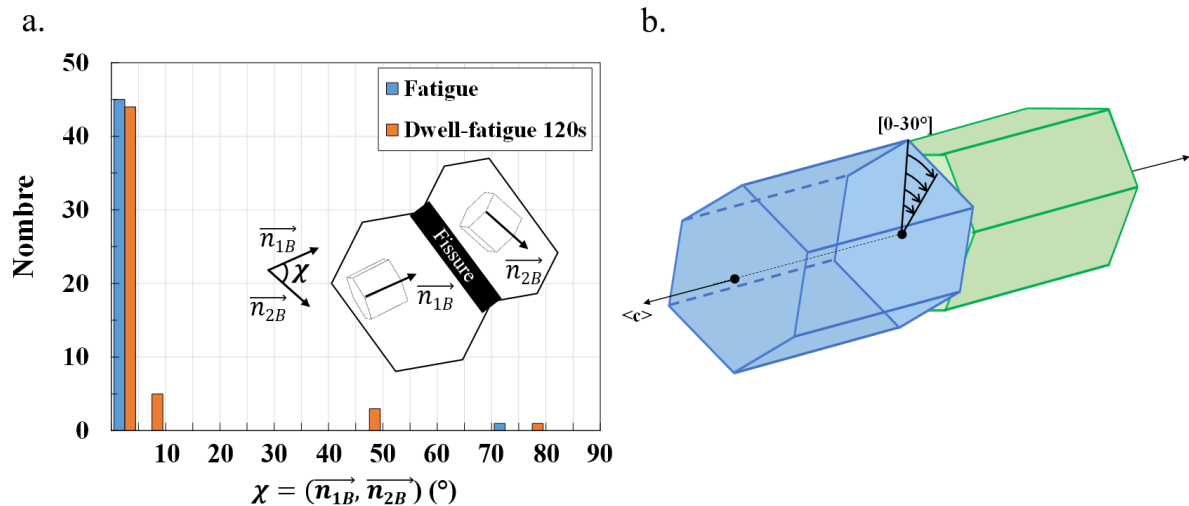
Figure V-7 : a. Distribution en nombre par intervalle de 5^\circ des valeurs des angles \chi entre par les normales au plan basal de chaque côté des fissures surfaciques pour un chargement en fatigue et dwell-fatigue 120s à 0,90 \times R_p^{0,2\%} . b. Représentation schématique de la relation d'orientation particulière entre les mailles hexagonales de part et d'autre des fissures d'après l'analyse statistique de l'angle \chi .
