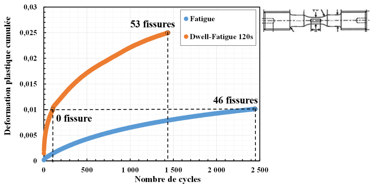
Figure V-1 : Déformation plastique cumulée en fonction du nombre de cycles pour les essais de fatigue et dwell-fatigue 120s effectué à 0,90 \times R_p^{0,2\%} sur les éprouvettes cylindriques contenant des méplats et usinées à partir du lot de matière II. Les interruptions de chaque essai et le nombre de fissures correspondant en surface sont indiqués.
