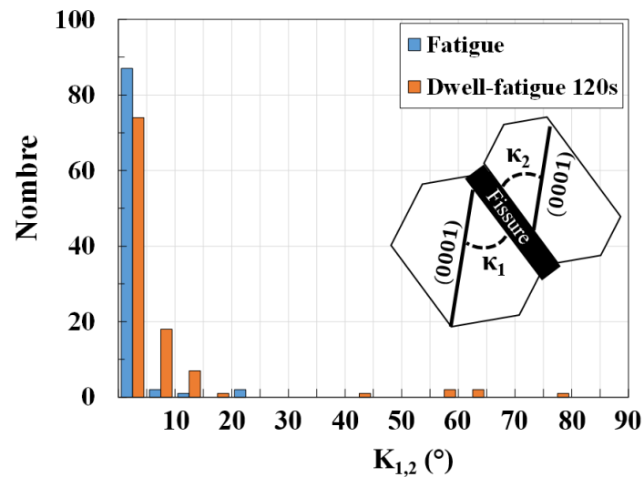
Figure V-4 : Distribution en nombre par intervalle de 5^\circ des valeurs d'angle K mesurées entre les traces des plans basaux et des fissures en surface pour un chargement en fatigue et dwell-fatigue 120s à 0,90 \times R_p^{0,2\%} .
