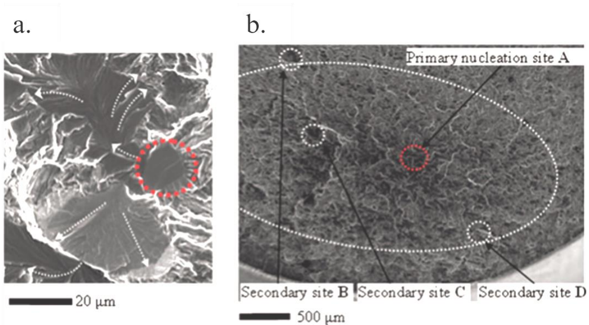
Figure I-36 : Micrographies MEB d'un faciès de rupture obtenu par un chargement en dwell-fatigue : a. site principal d'amorçage avec observation d'une facette de quasi-clivage entourée et b. position des différentes facettes d'amorçage sur le faciès de rupture (Uta et al., 2009).
