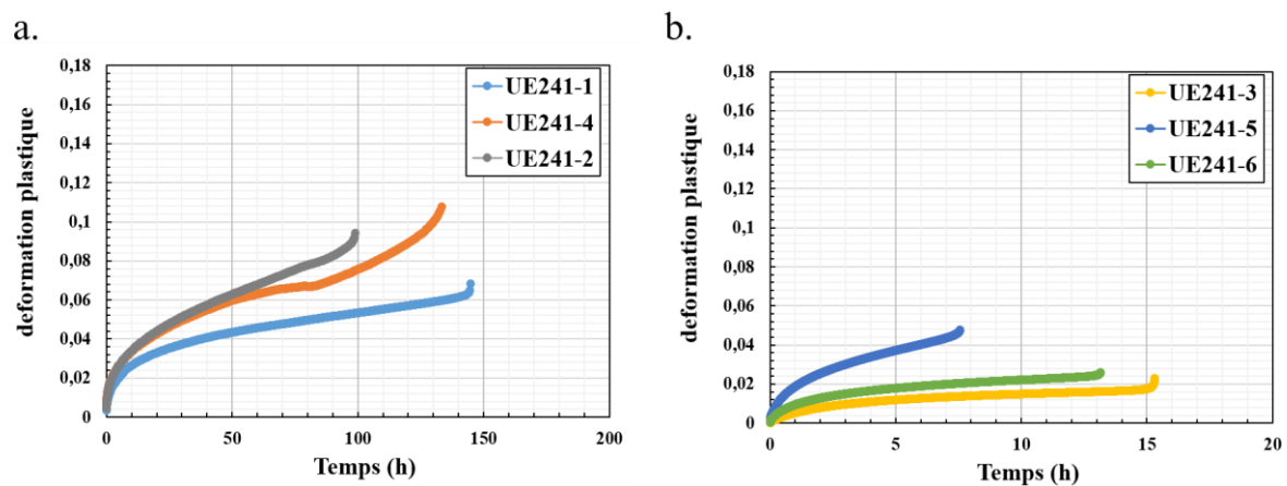
Figure III-16 : Evolution de la déformation plastique en fonction du temps pour les essais de a. dwell-fatigue et b. fatigue réalisés à \sigma_{\max} = 0,90 \times R_p^{0,2\%}
