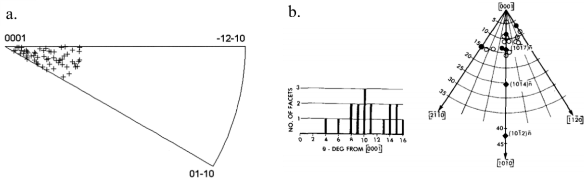
Figure I-37: Orientations cristallographiques des facettes subsurface de dwell-fatigue représentées sur une figure de pôles inverse codée selon a. la direction de sollicitation pour un alliage IMI 834 (Bache et al., 1997a) et b. selon la normale au plan de quasi-clivage pour un alliage IMI 685 (Davidson and Eylon, 1980).
