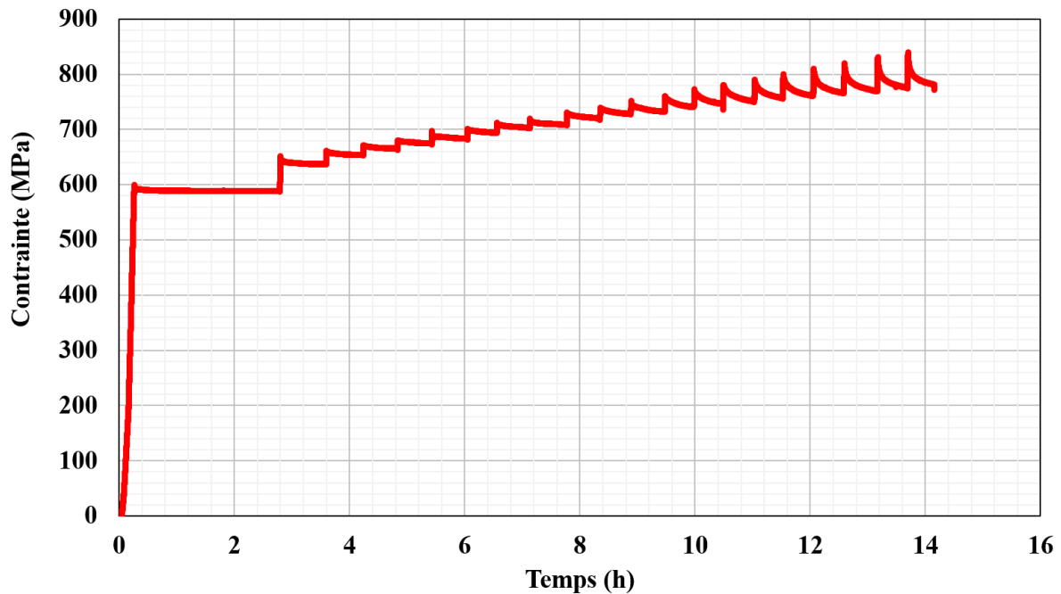
Figure III-3 : Evolution de la contrainte en fonction du temps d'essai en heures durant l'essai de traction in situ sous MEB
