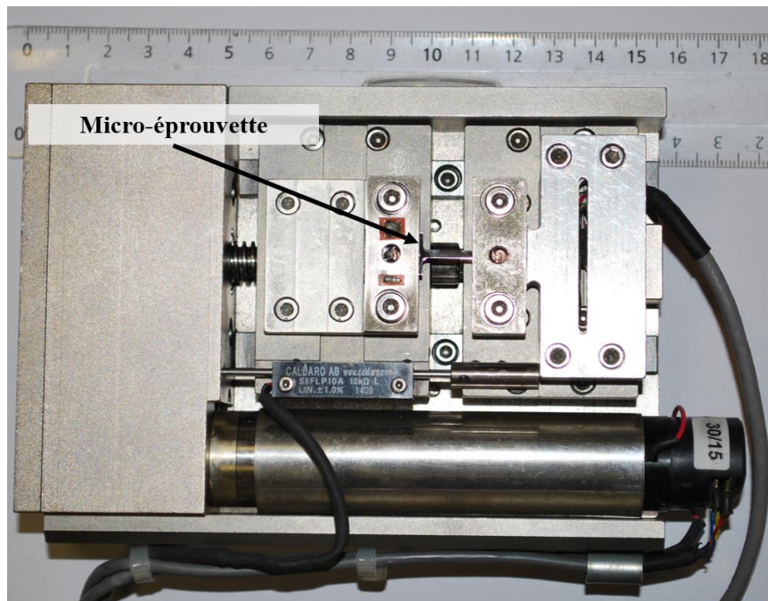
Figure II-9 : Micromachine pour essai de traction in situ sous MEB
