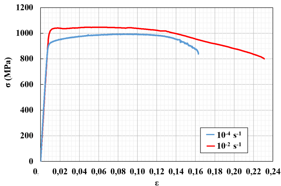
Figure II-8 : Courbes de traction réalisées sur le lot de matière II à vitesse de déplacement imposée.
