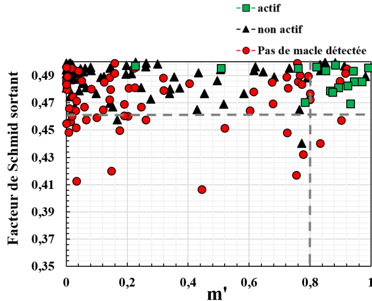
Figure IV-23 : Facteur de Schmid sortant en fonction du paramètre m' associé des 6 systèmes de maillage \{10\bar{1}2\} pour chaque interaction d'une bande de glissement avec l'interface d'un nodule étudié. Les distributions et le code de couleurs associé sont équivalents à ce qui est décrit pour le graphique de la Figure IV-21.
