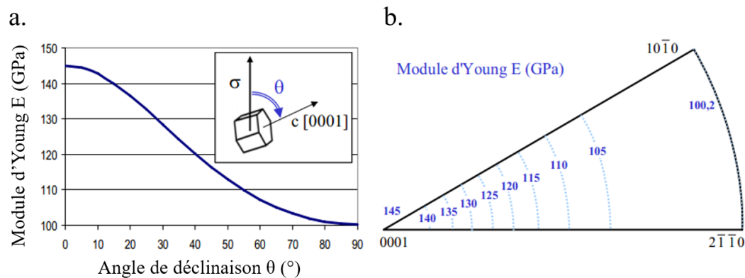
Figure I-2 : a. Evolution du module d'Young de la phase \alpha en fonction de l'angle de déclinaison \theta . b. figure de pôles inverse codée selon la direction de sollicitation avec les iso-contours du module d'Young de la phase \alpha (Bridier, 2006)
