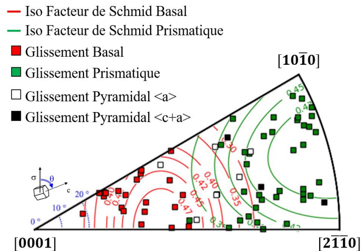
Figure III-6 : Représentation de l'orientation cristallographique des nodules présentant des traces de glissement prismatique, basal, pyramidal \langle a \rangle et \langle c+a \rangle sur une figure de pôles inverse codée selon la direction de sollicitation. Les iso-contours des facteurs de Schmid pour les modes de glissement basal et prismatique sont également représentés.
