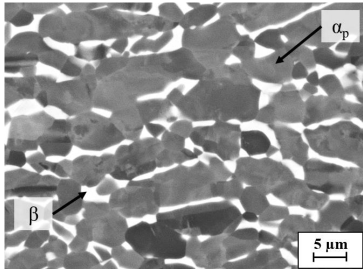
Figure I-9: Microstructure équiaxe d'un alliage Ti-6Al-4V
