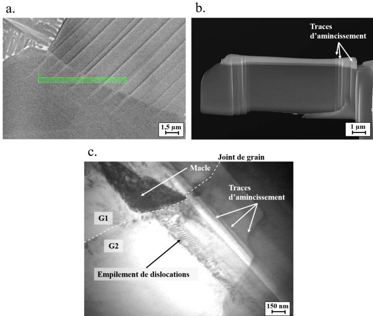
Figure IV-18 : Micrographies MEB a. du positionnement de prélèvement de la lame mince et b. de la lame mince pour le cas d'étude de la Figure IV-16. c. Micrographie MET selon le vecteur \vec{g} = [\bar{1}013] du cas d'étude de la Figure IV-16. La micrographie montre que la macle observée dans le nodule G1 est localisée en tête d'un empilement de dislocations contenue dans un plan prismatique du nodule G2.
