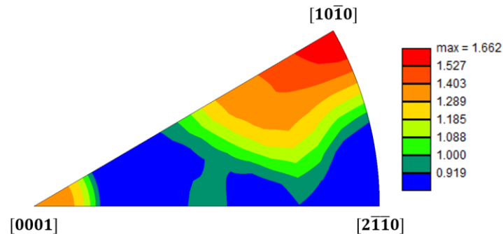
Figure III-1 : Distribution des orientations cristallographiques contenues dans les zones d'études sur une figure de pôle inverses codée selon la direction de sollicitation.
