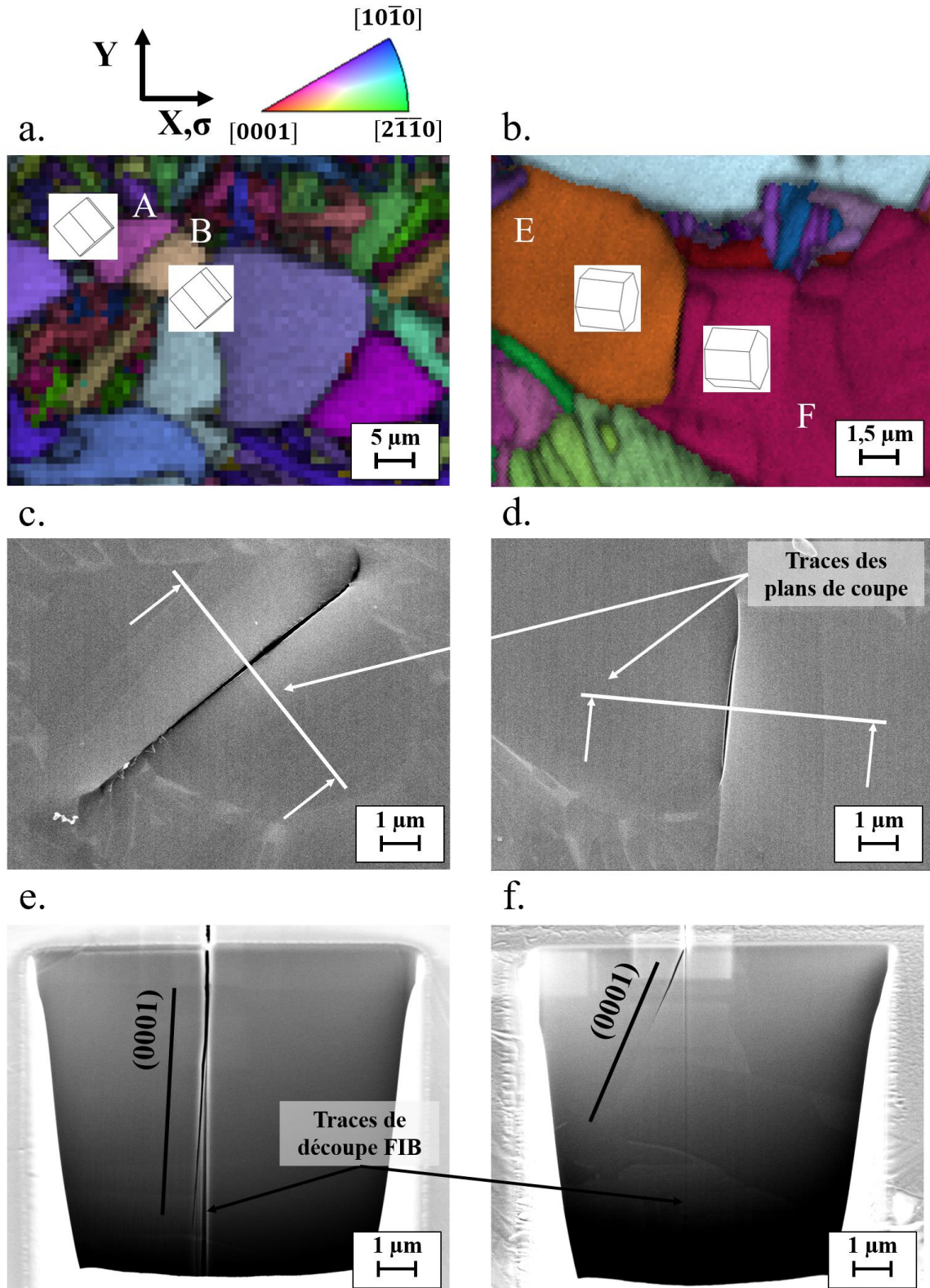
Figure V-16 : Etude de l'amorçage de deux fissures surfaciques pour un chargement en dwell-fatigue à 0,90 \times R_p^{0,2\%} au moyen de coupes transverses réalisées avec un MEB-FIB. Cartographie d'orientations cristallographiques codées selon la direction de sollicitation dévoilant les interfaces d'intérêt entre les nœuds A,B (a) et E,F (b). Micrographies MEB (c,d) des sites microstructuraux après 1438 cycles et 2,5% de déformation plastique. Micrographies MEB (e,f) des coupes transverses.
