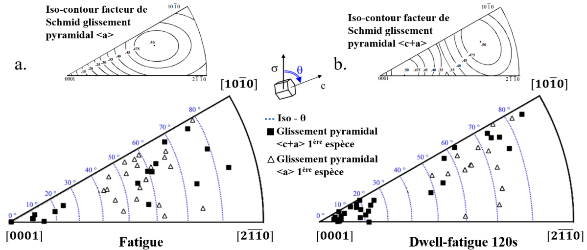
Figure IV-12 : Représentation sur une figure de pôles inverse codée selon la direction de sollicitation des orientations cristallographiques des nœuds où des traces de glissement pyramidal \langle a \rangle et \langle c+a \rangle de 1 ère espèce ont été identifiées à 2,5% de déformation plastique en a. fatigue et b. dwell-fatigue 120s à \sigma_{\max} = 0,94 \times R_p^{0,2\%} . Les iso-contours de l'angle de déclinaison \theta sont superposées.
