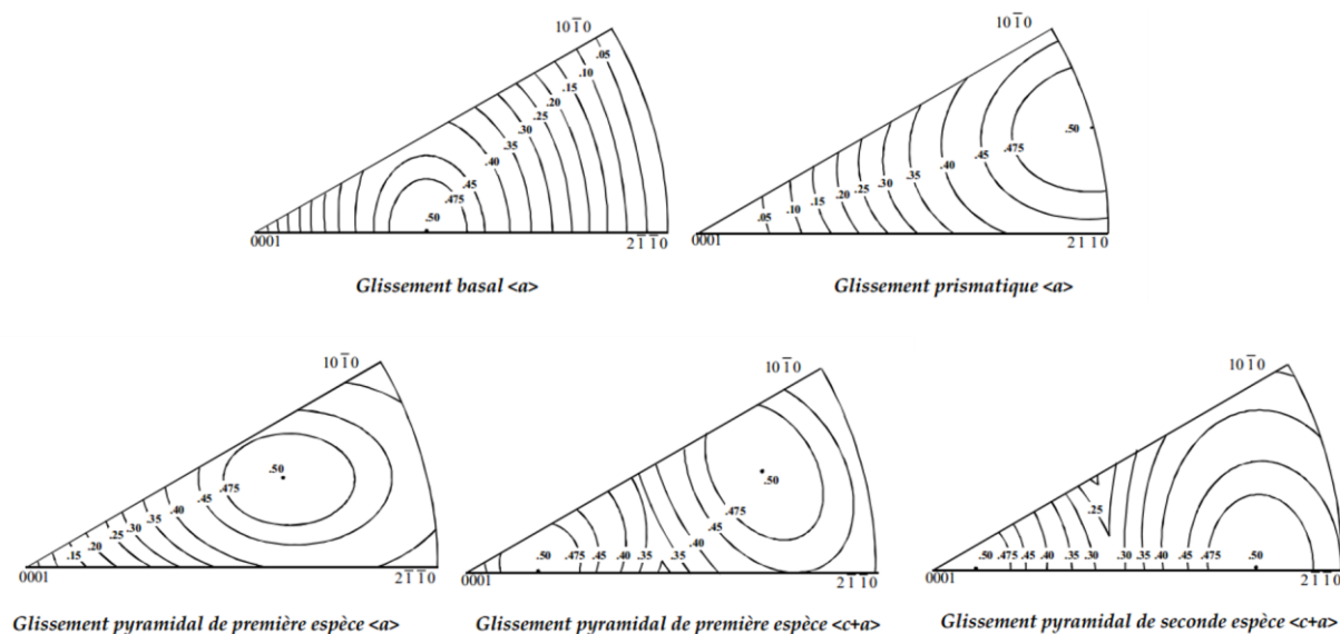
Figure I-15: Figures de pôles inverses codées selon la direction de sollicitation avec les iso-contours des facteurs de Schmid pour les différents modes de glissement du titane \alpha (Bridier, 2006)
