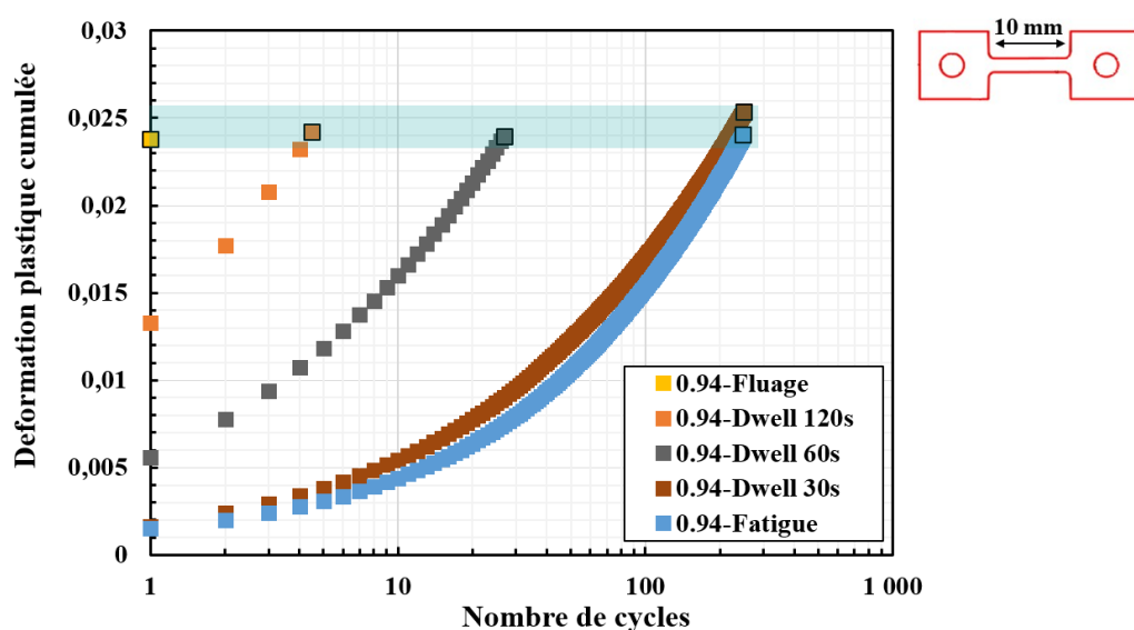
Figure IV-2 : Déformation plastique en fonction du nombre de cycles pour les essais cycliques interrompus à \sigma_{\max} = 0,94 \times R_p^{0,2\%}
