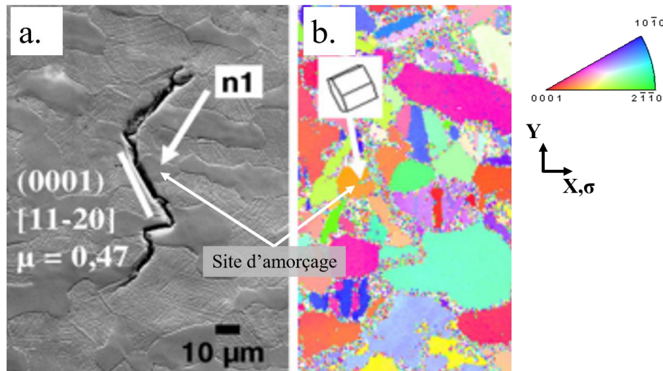
Figure I-35: a. Micrographie MEB d'une fissure de fatigue secondaire et b. cartographie des orientations associées projetées selon la direction de sollicitation (Bridier et al., 2008)
