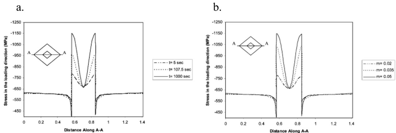
Figure I-32 : Niveau de contrainte selon la direction de sollicitation dans une configuration microstructurale grain dur/ grain mou a. en fonction du temps de maintien à charge maximale et b. en fonction de la sensibilité à la vitesse de déformation pour un chargement de fluage à un niveau de contrainte de -606 MPa d'un alliage Ti-6Al (Hasija et al., 2003)
