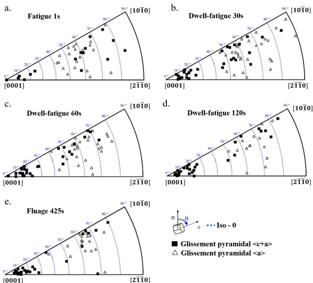
Figure B-1 : Orientations cristallographiques des nodules \alpha_p présentant des traces de glissement pyramidal \langle a \rangle et \langle c+a \rangle représentées sur une figure de pôles inverse codée selon la direction de sollicitation après une déformation plastique de 2,5% en a. fatigue, dwell-fatigue b. 30s, c. 60s, d. 120s et e. fluage à \sigma_{\max} = 0,94 \times R_p^{0,2\%} .
