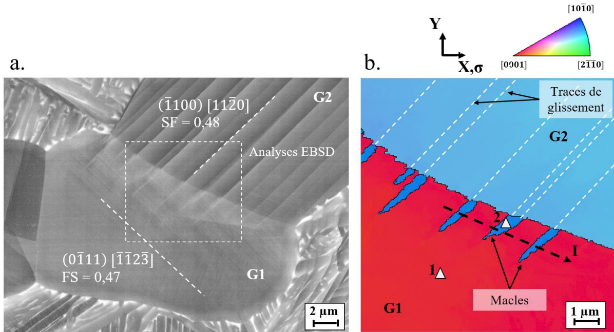
Figure IV-16 : a. Micrographie MEB d'une paire de nodules \alpha_p dur (G1) et mou (G2). b. Cartographie des orientations cristallographiques codées selon la direction de sollicitation et centrée sur l'interface entre le nodule mou et le nodule dur. La cartographie révèle la présence de macles au sein du nodule dur en face des traces de glissement prismatique du nodule mou.
