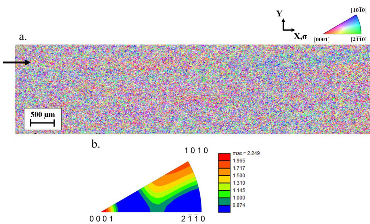
Figure II-3 : a. Cartographie des orientations cristallographiques en surface de la zone utile d'une micro-éprouvette représentative des directions US5.2 et US5.4 et b. Distribution des orientations cristallographiques représentée sur une figure de pôles inverse codée selon la direction de sollicitation (X)
