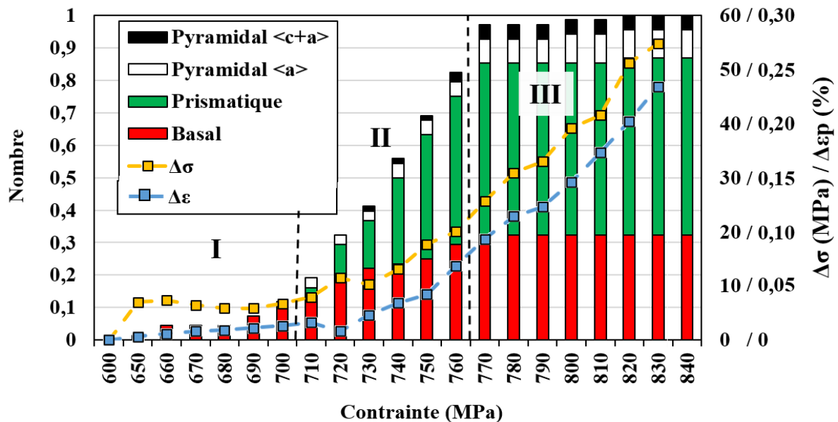
Figure III-10 : Evolution de la fraction de systèmes de glissement actif et des variations de contrainte et de déformation de la contrainte relaxée en fonction du niveau de contrainte appliqué
