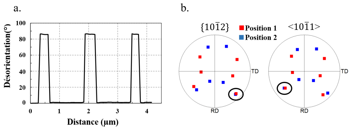
Figure IV-17 : a. Profil de désorientation cristallographique depuis le point d'origine du chemin I défini en Figure IV-16 et b. représentation des orientations des plans \{10\bar{1}2\} et des directions \langle 10\bar{1}1 \rangle dans le repère échantillon aux points 1 et 2 définis en Figure IV-16b.
