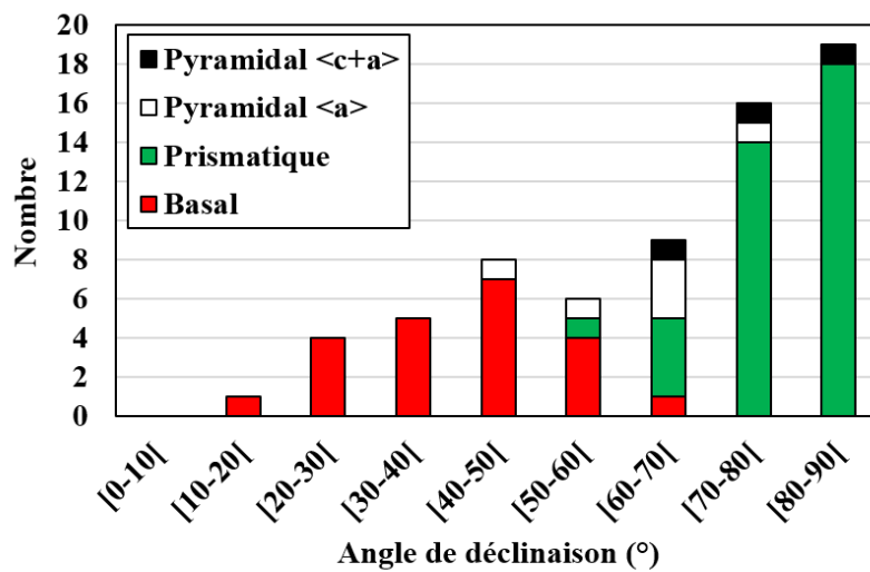
Figure III-8 : Histogramme de répartition en nombre des systèmes de glissement prismatique, basal, pyramidal \langle a \rangle et \langle c+a \rangle en fonction de l'angle de déclinaison du nodule au sein duquel ils ont été identifiés
