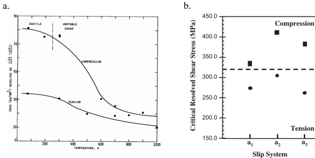
Figure I-19 : a. Cission critique résolue pour le glissement pyramidal \langle c+a \rangle en fonction de la température pour une sollicitation en traction et en compression de monocristaux d'alliage Ti-5Al (Williams et al., 2002), et b., cissions critiques résolues pour le glissement basal en traction et en compression pour une sollicitation uniaxiale de monocolonies lamellaires dans un alliage Ti-6242 (Neeraj et al., 2005).
