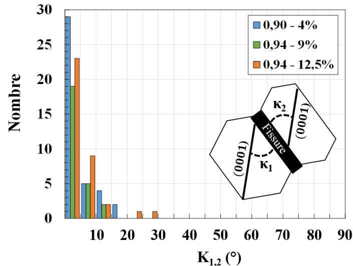
Figure V-11 : Distribution en nombre par intervalle de 5^\circ des angles K mesurés entre les traces de plan basal et des fissures subsurfaciques pour des chargements en dwell-fatigue 120s à 0,90 \times R_p^{0,2\%} interrompu à 4% de déformation plastique ainsi qu'à 0,94 \times R_p^{0,2\%} interrompus à 9% et 12,5% de déformation plastique.
