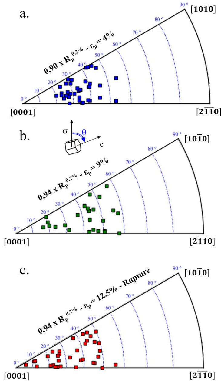
Figure V-10 : Orientations cristallographiques des nœuds \alpha_p présents aux sites d'amorçage des fissures subsurfaciques pour un chargement en dwell-fatigue 120s à a. 0,90 \times R_p^{0,2\%} et 4% de déformation plastique, b. 0,94 \times R_p^{0,2\%} et 9% de déformation plastique et c. 0,94 \times R_p^{0,2\%} et 12,5% de déformation plastique.
