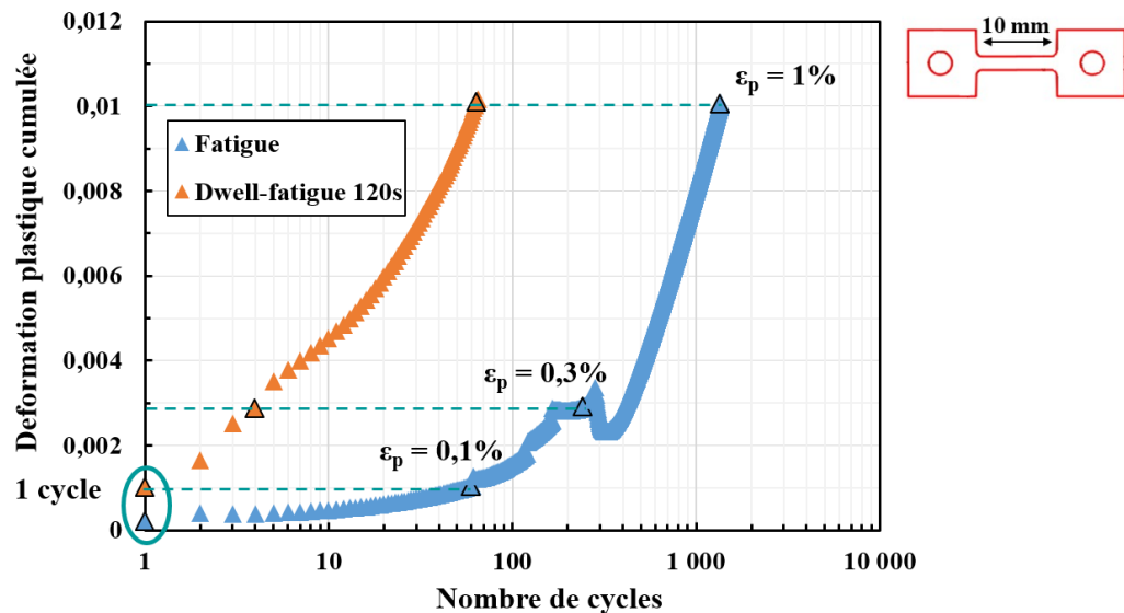
Figure IV-1 : Evolution de la déformation plastique en fonction du nombre de cycles pour les essais cycliques interrompus à \sigma_{\max} = 0,90 \times R_p^{0,2\%} .
