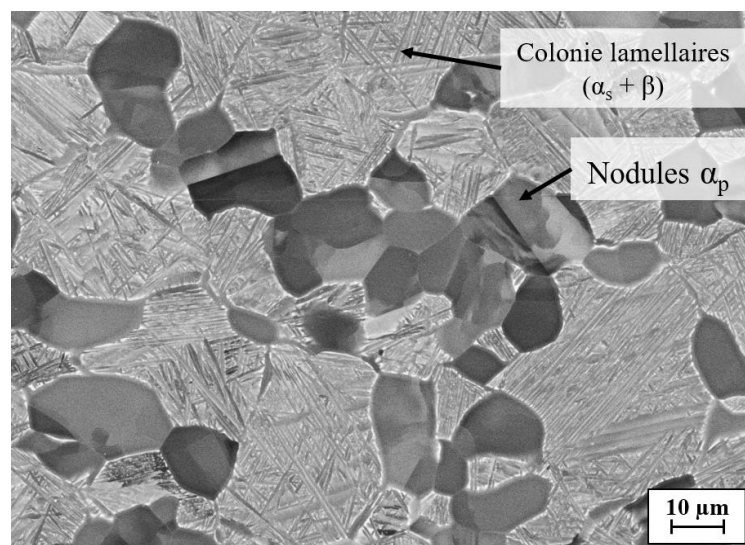
Figure I-10 : Microstructure bimodale d'un alliage Ti-6Al-4V
