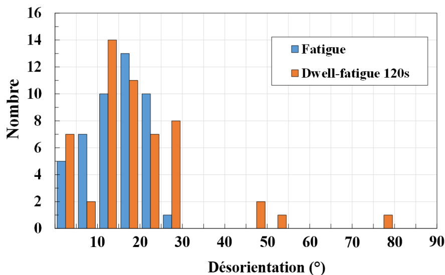
Figure V-6 : Distribution en nombre par intervalle de 5° des mesures de désorientation cristallographique de la phase \alpha_p au site d'amorçage des fissures surfaciques en fatigue et dwell-fatigue 120s à 0,90 \times R_{p0,2\%} .
