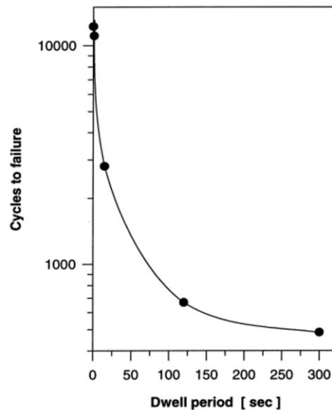
Figure I-23: Influence du temps de maintien sur la durée de vie de l'alliage IMI 834 avec une microstructure bimodale (880 MPa, R=0,1) (Bache et al., 1997a)
