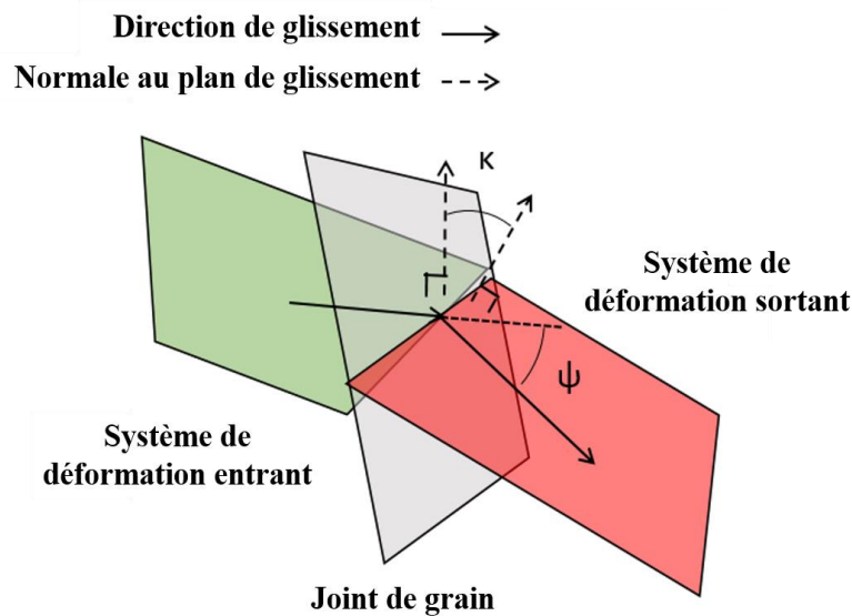
Figure II-16 : Représentation schématique de l'orientation de deux systèmes de glissement de part et d'autre d'une interface.
