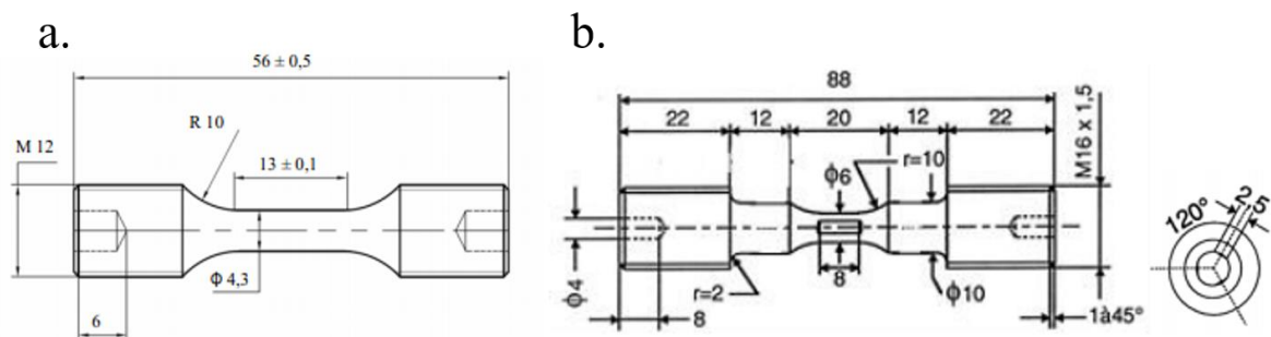
Figure II-6 : Géométrie des éprouvettes cylindriques a. pour les essais de durée de vie et b. pour l'étude des mécanismes de déformation et d'endommagement en surface
