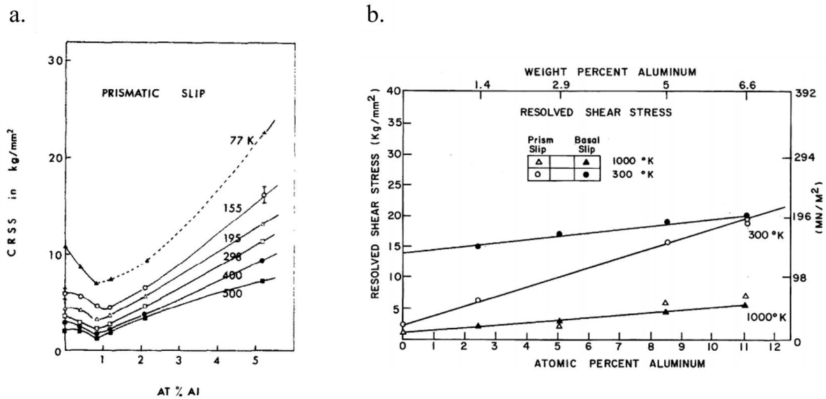
Figure I-18 : Influence de l'aluminium sur la cisssion critique du glissement prismatique et basal selon les études de a. Sakai et Fine et b. Williams et al. (Sakai and Fine, 1974; Williams et al., 2002)
