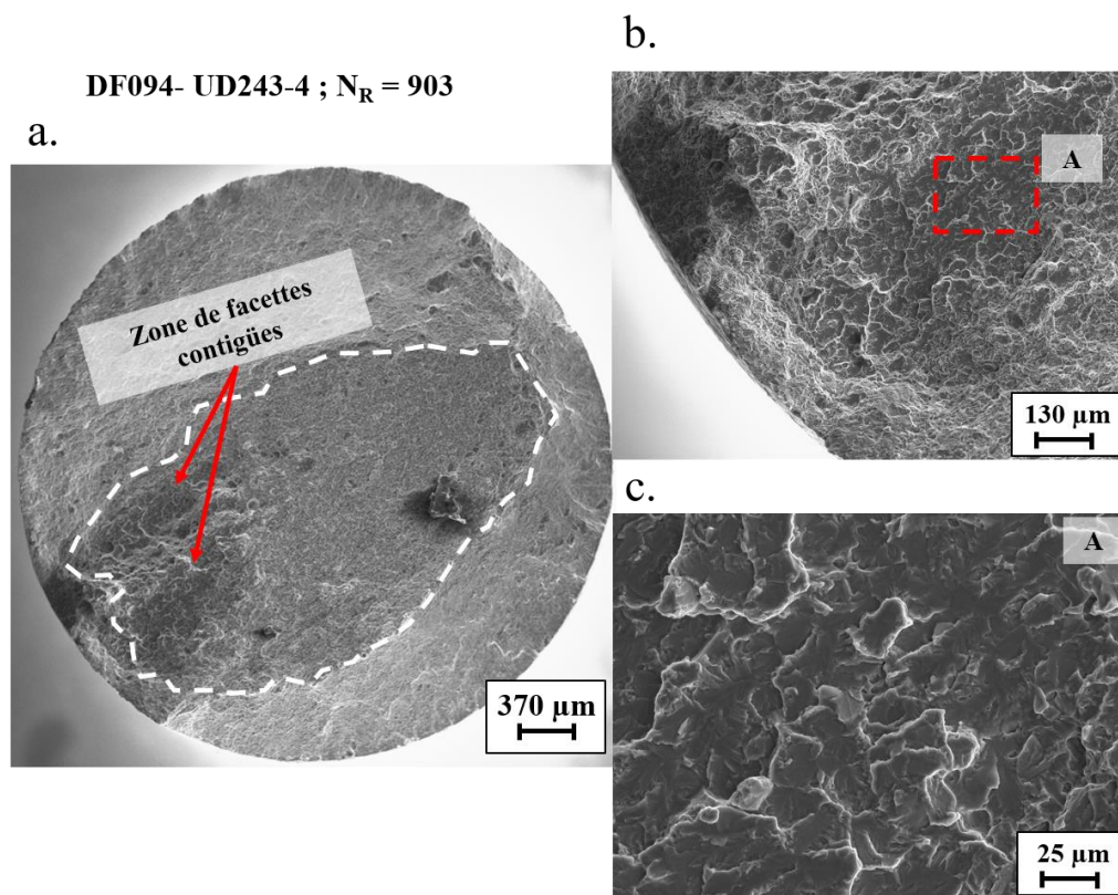
Figure III-26 : Micrographies MEB à différents grossissements du faciès de rupture de l'éprouvette UD243-4 obtenue par dwell-fatigue à \sigma_{\max} = 0,94 \times R_p^{0,2\%} .
