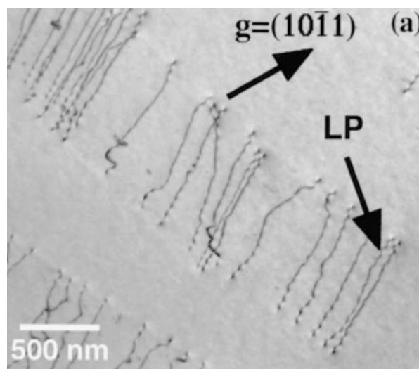
Figure I-21 : Micrographie TEM d'un empilement de dislocations dû à la présence d'ordre à courte distance (Neeraj and Mills, 2001)
