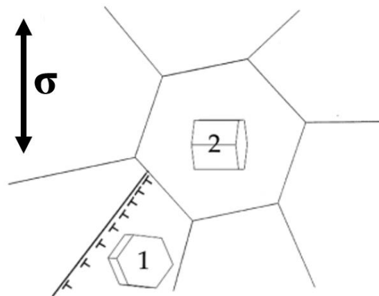
Figure I-41 : Représentation schématique de la configuration grain mou/grain mou d'amorçage de fissure subsurfacique en l'absence de grain dur (Everaerts et al., 2017).
