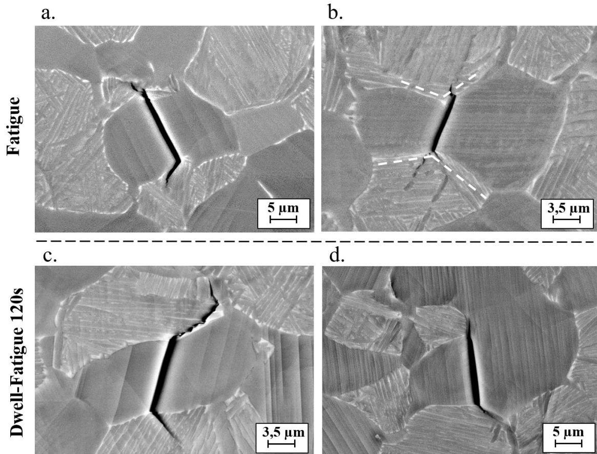
Figure V-2 : Micrographie MEB de fissures détectées en surface des éprouvettes sollicitées en fatigue (a,b) et dwell-fatigue 120s (c,d) à 0,90 \times R_p^{0,2\%} . La morphologie de la phase \alpha_p de la micrographie en (b) suggère que l'amorçage de fissure a lieu aux environs d'un joint de grain entre deux nodules \alpha_p .
