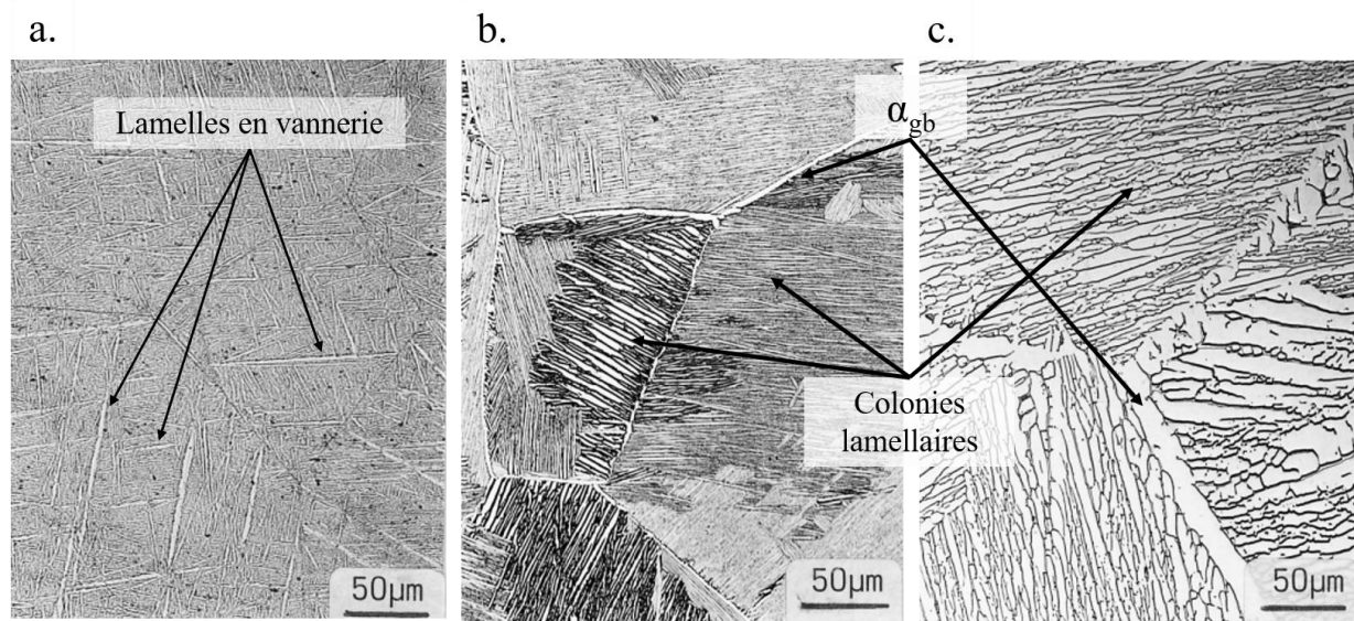
Figure I-8: Microstructures lamellaires pour un alliage de Ti-6242. La vitesse de refroidissement diminue de a. vers c. (Lütjering, 1998)
