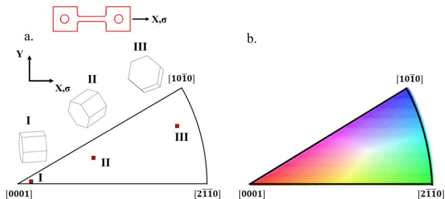
Figure II-14 : Représentation des orientations cristallographique des mailles cristalline I, II et III sur une figure de pôles inverse codée selon la direction X. b. Définition du code de couleur pour la représentation des orientations cristallographiques sur des cartographies.
