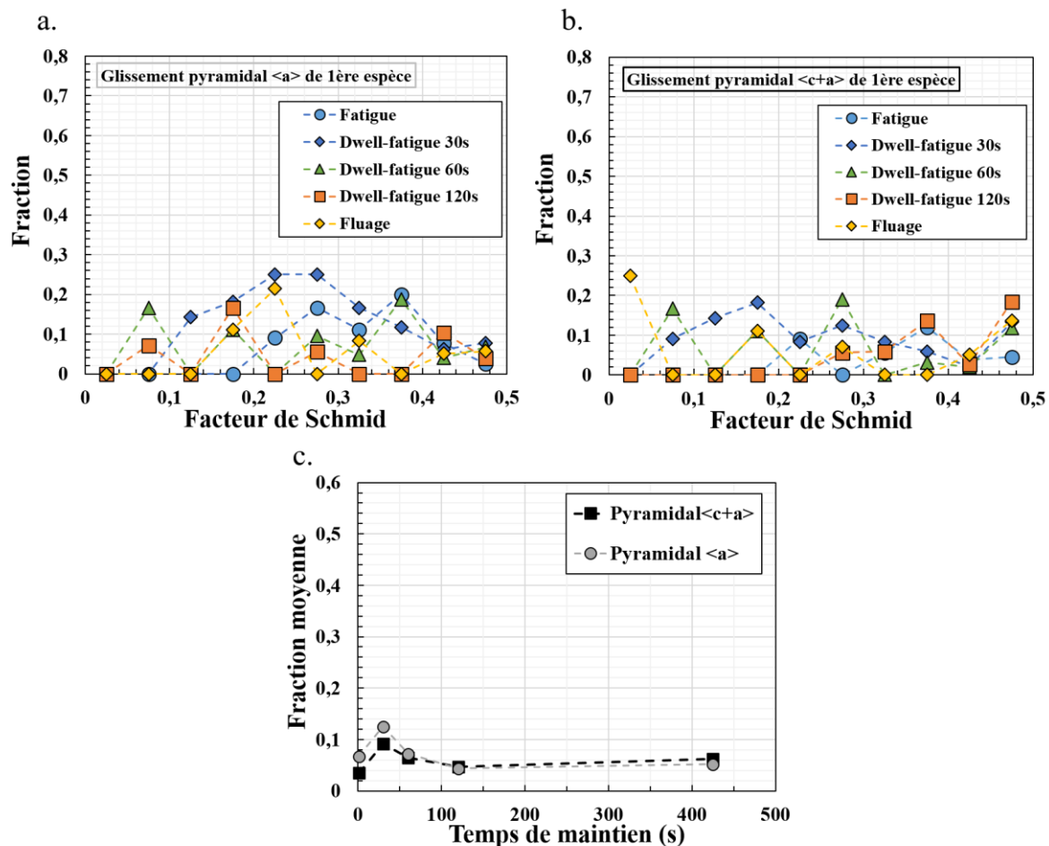
Figure IV-13 : Distribution des fractions des systèmes de glissement pyramidal de 1 ère espèce selon les directions a. \langle a \rangle et b. \langle c+a \rangle actifs après 2,5% de déformation plastique en fatigue, dwell-fatigue 30s, 60s, 120s et fluage à 0,94 \times R_p^{0,2\%} par intervalle de facteur de Schmid de 0,05. c. Moyenne des fractions des systèmes de glissement pyramidal \langle a \rangle et \langle c+a \rangle actifs en fonction du temps de maintien à charge maximale.
