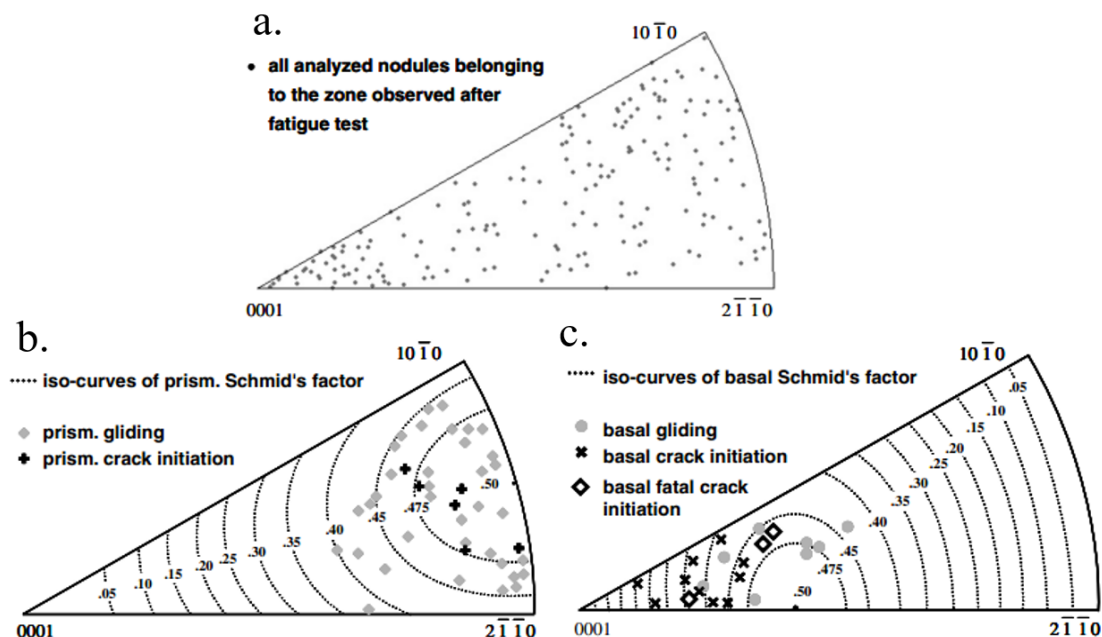
Figure I-27 : Orientations cristallographiques des nodules a. d'études et présentant des traces de glissement ou un amorçage de fissure b. prismatique et c. basal représentés sur des figures de pôles inverses codées selon la direction de sollicitation (Bridier et al., 2008)
