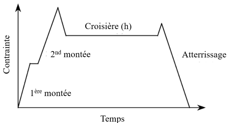
Figure 1 : Représentation schématique du chargement des disques de moteurs d'avion durant un vol (Bache, 2003).
