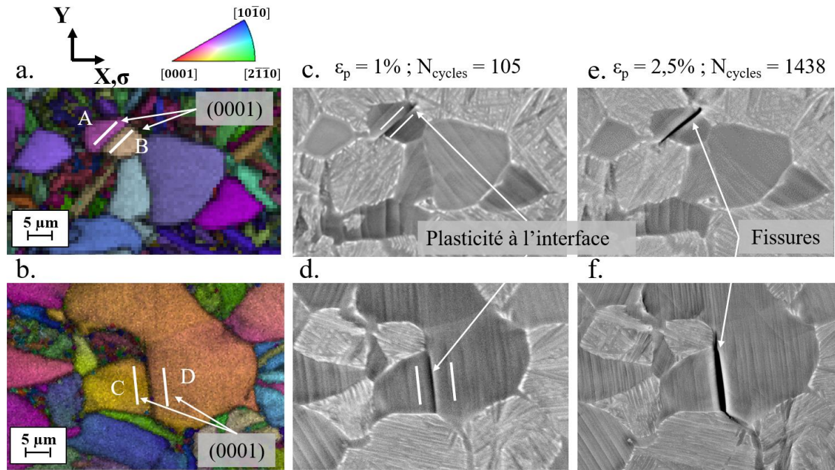
Figure V-15 : Etude ex situ de l'amorçage de deux fissures surfaciques pour un chargement en dwell-fatigue 120s à \sigma_{\max} = 0,90 \times R_p^{0,2\%} . Cartographie d'orientations cristallographiques codées selon la direction de sollicitation incluant les interfaces d'intérêt entre les nodules A,B (a) et C,D (b). Micrographie MEB (c,d) des sites d'amorçage des fissures après 105 cycles et 1% de déformation plastique montrant un glissement aux interfaces. Micrographie MEB (e,f) montrant l'amorçage de fissure aux interfaces d'intérêt après 1438 cycles et 2,5% de déformation plastique.
