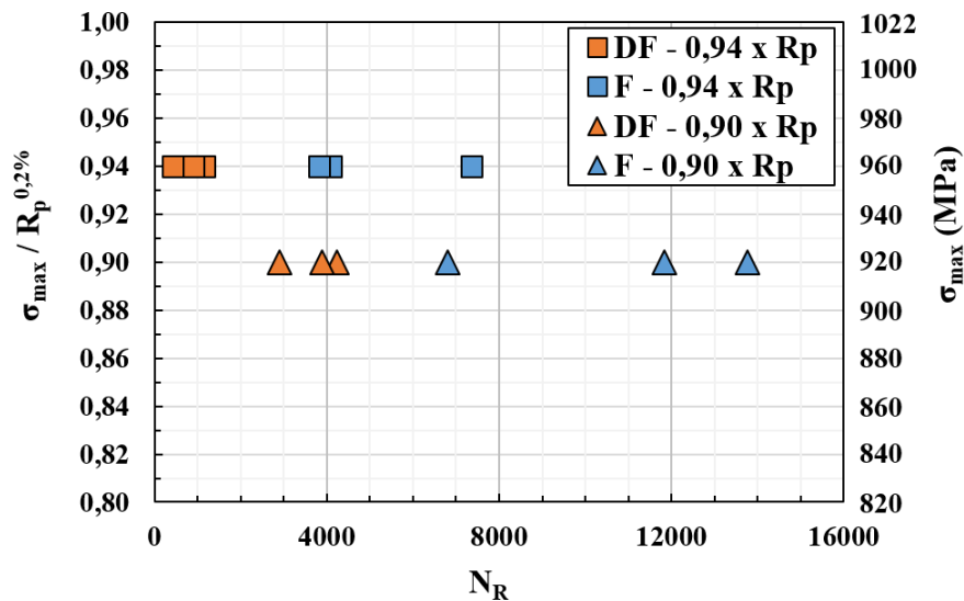
Figure III-19 : Nombre de cycles à rupture N_R en fonction du niveau de contrainte maximal appliqué en cours de cycle normalisé par la limite d'élasticité pour les essais de fatigue (F) et de dwell-fatigue 120s (DF).
