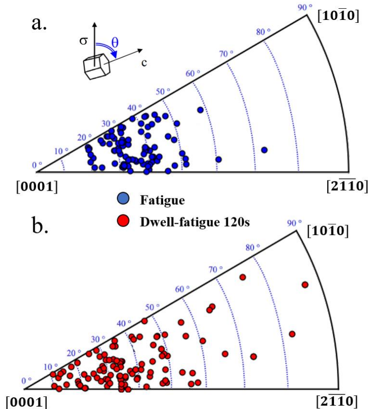
Figure V-3 : Orientations cristallographiques par rapport à la direction de chargement des nodules \alpha_p présents aux sites d'amorçage des fissures détectées en surface pour un chargement en a. fatigue et b. dwell-fatigue 120s à 0,90 \times R_p^{0,2\%} .
