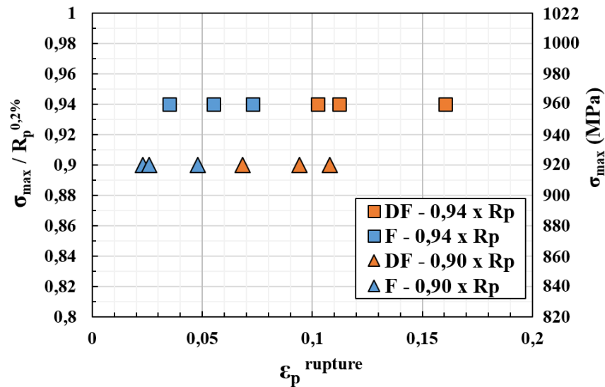
Figure III-21 : Déformation plastique à rupture en fonction du niveau de contrainte maximale appliqué pour les essais de fatigue (F) et de dwell-fatigue 120s (DF).
