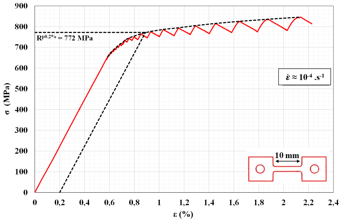
Figure III-4 : Courbe contrainte-déformation conventionnelle correspondant à l'essai in situ sous MEB
