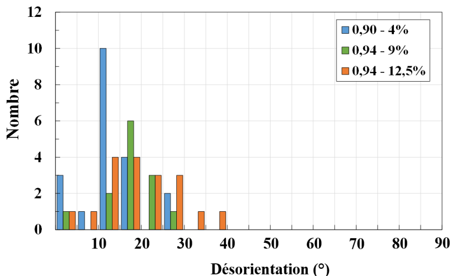
Figure V-13 : Distribution en nombre par intervalle de 5^\circ de l'angle de désorientation cristallographique de la phase \alpha_p de part et d'autre des fissures subsurfaciques en dwell-fatigue 120s à 0,90 \times R_p^{0,2\%} interrompu à 4% de déformation plastique ainsi qu'à 0,94 \times R_p^{0,2\%} interrompu à 9% et 12,5% de déformation plastique.
