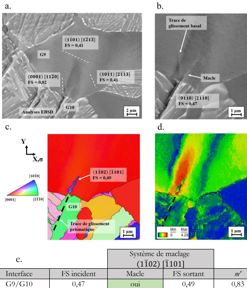
Figure IV-29 : a,b. Micrographies MEB montrant une bande de glissement prismatique contenue dans la colonie lamellaire G10 et bloquée à l'interface du nodule G9. c. Cartographie des orientations cristallographiques codées selon la direction de sollicitation montrant une macule à l'interface entre G9 et G10. d. Cartographie des désorientations cristallographiques au sein des grains (« Grain Reference Orientation Deviation map ») montrant la présence d'un gradient de désorientations dans le nodule G9 en face de la bande de glissement prismatique. e. Facteur de Schmid incident et sortant et paramètre m' pour l'analyse du maclage (1102) [1101] à l'interfaces entre G9 et G10.
