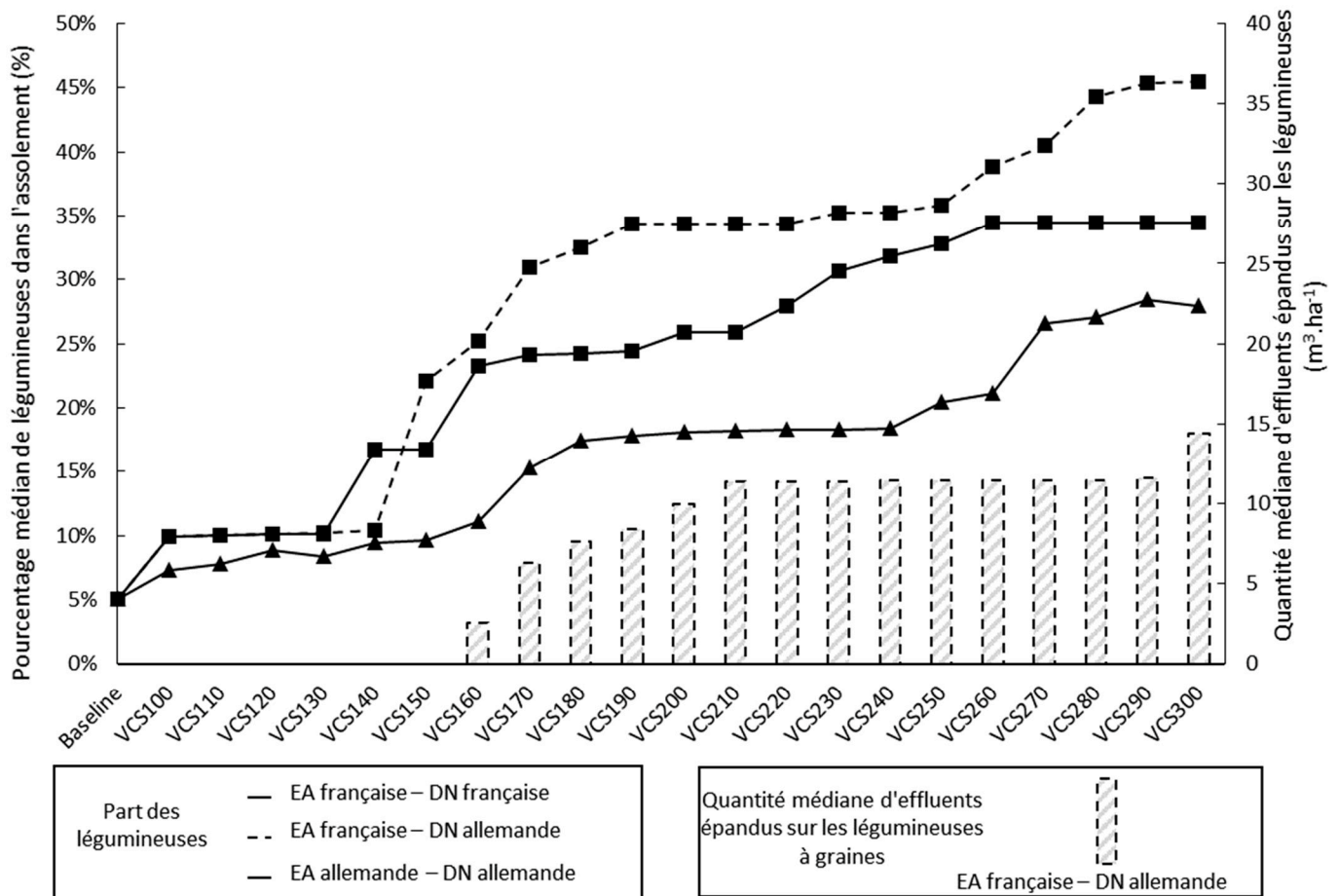
Figure S3. Pourcentage de légumineuses dans l'assolement (hors prairies) et quantité d'effluents épanchés sur les légumineuses à graines (médianes), par exploitation et application de la Directive Nitrates (DN), selon différents niveaux d'aides couplées aux légumineuses (ex : VCS100 équivaut à une aide couplée de 100€.ha -1 )
