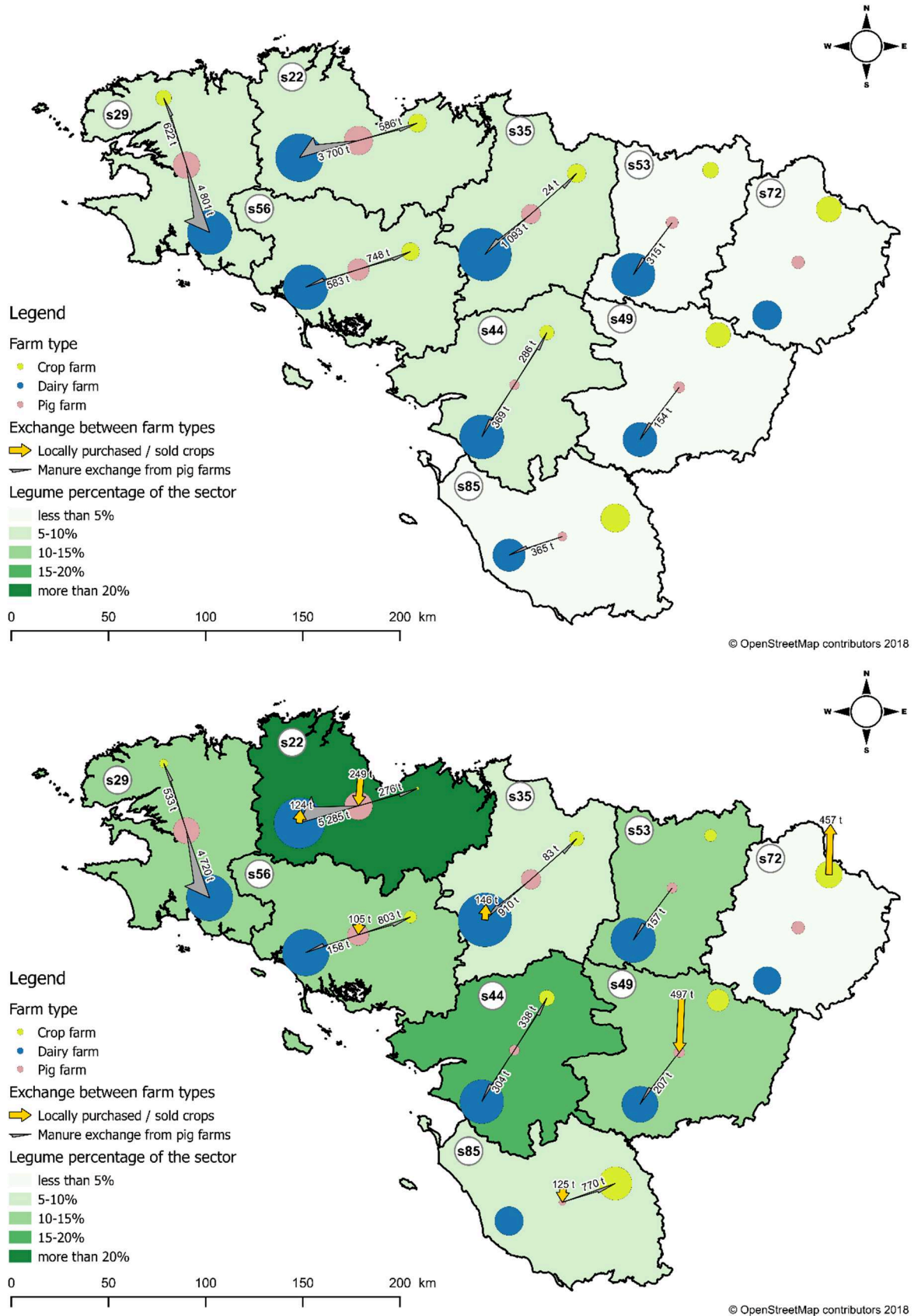
Figure S.3. Production de légumineuses et échanges entre exploitations de cultures et d'effluents dans l'ouest de la France, dans la situation initiale (a) et avec une augmentation de la demande en produits animaux sans OGM
