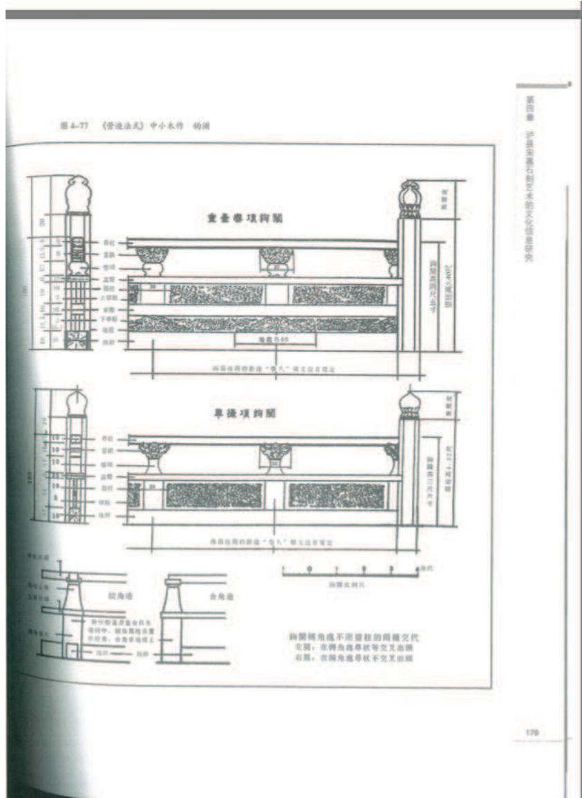
Illustration 31: Plan de détail de l'architecture d'une balustrade de Goulan de la dynastie Song (960-1279).
