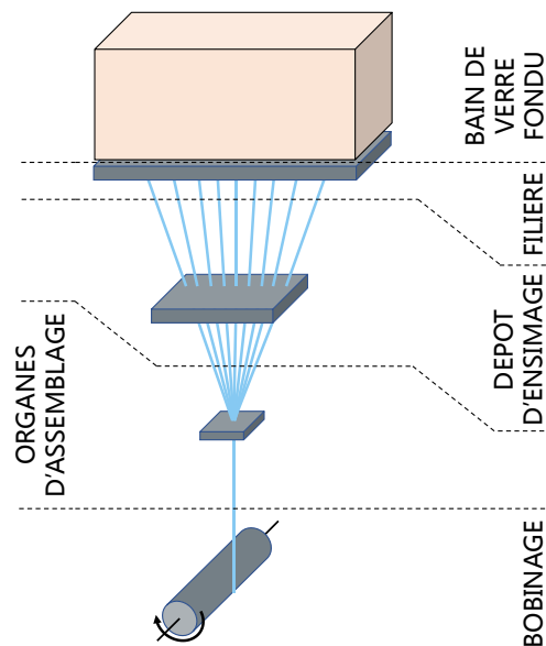
FIGURE 1.3 – Illustration du processus de fabrication des fibres de verre [BER 08]
