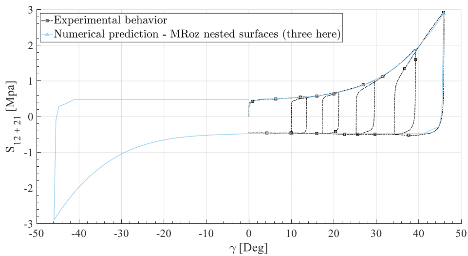
FIGURE 4.13 – Description par morceau de la boucle d’hystérésis pour des angles positifs et négatifs
