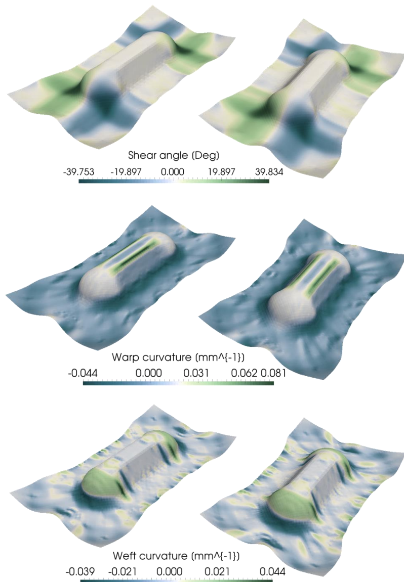
FIGURE 5.32 – Comparatif des résultats entre les approches F (à gauche) et I (à droite) pour la simulation de double dôme
