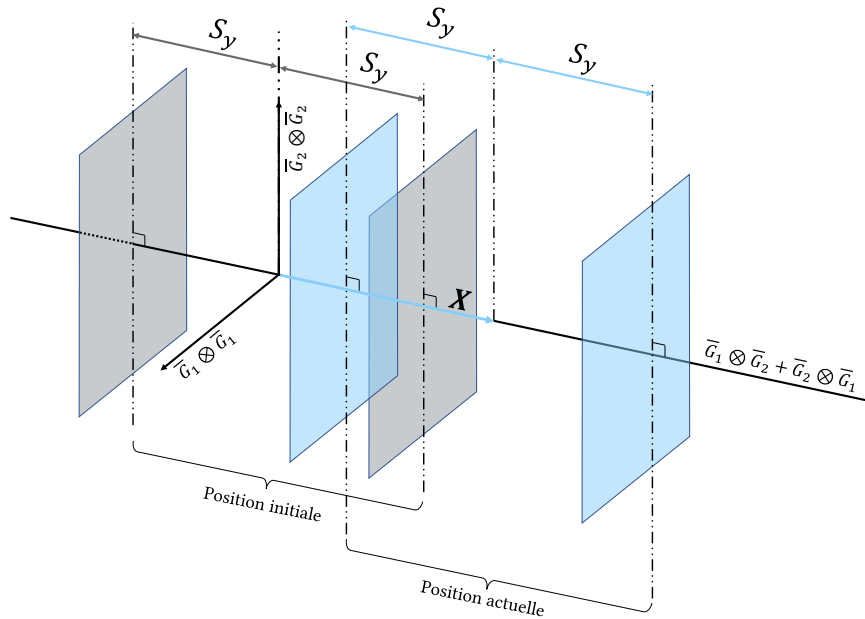
FIGURE 3.11 – Schématisation de l'érouissage cinématique en l'appliquant sur la surface de charge définie précédemment
