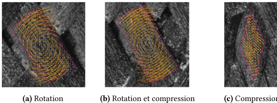
FIGURE 1.28 – Mécanisme de cisaillement du tissu Hexcel®G1151 [LUY 09b]
