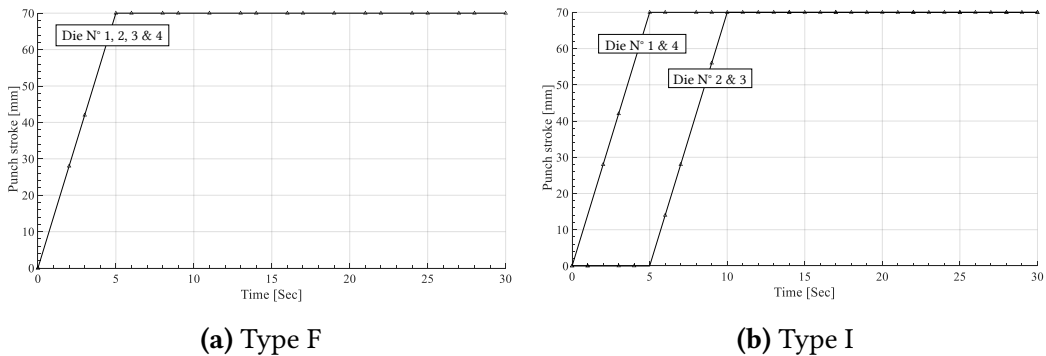
FIGURE 5.24 – Chargements étudiés pour la mise en forme en U
