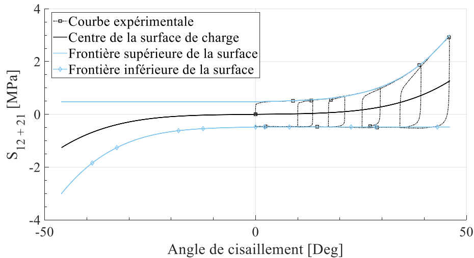
FIGURE 3.15 – Évolution de l'écroissage mixte en fonction de l'angle de cisaillement
