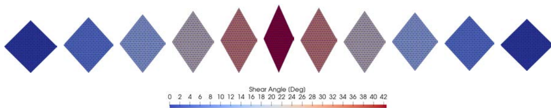
FIGURE 5.5 – Évolution de l'angle de cisaillement lors d'une simulation éléments finis d'un Picture Frame Test suivant une charge et une décharge
