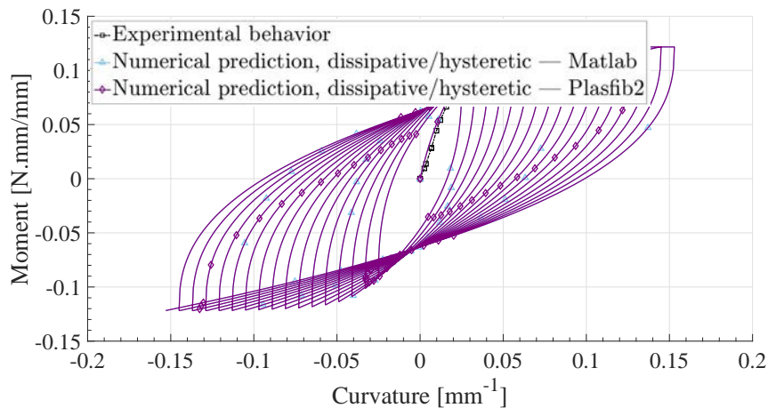
FIGURE 5.7 – Comparaison du modèle hystérétique entre l'approche expérimentale, la modélisation sur Matlab ® et la modélisation sur Plasfib2 pour un chargement non-monotone en flexion hors plan
