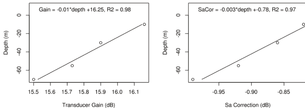
FIGURE 2.4 – Variation du gain du transducteur (en décibel) et de la correction de Sa (indice de réflexion surfacique, en m^2 \cdot m^{-2} ) du sondeur de l'EROC avec la profondeur, pour une durée d'impulsion de 128 \mu s
