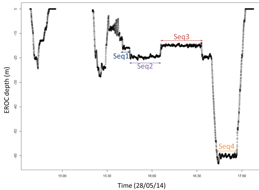
FIGURE 2.3 – Profondeur d'immersion de l'EROC en fonction du temps
