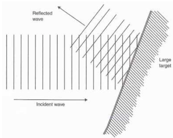
FIGURE A.5 – Retro-diffusion d'une grande cible par rapport à \lambda . L'écho correspond à la réflexion de l'onde incidente par la surface de la cible, d'après Simmonds and MacLennan (2005) .
