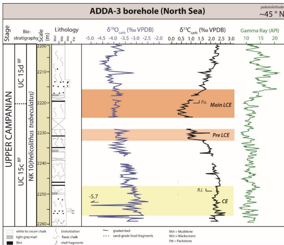
Figure 41 : Synthèse des données actuelles sur le forage Adda-3. Les données lithologiques, biostratigraphiques, de Gamma-Ray et isotopiques proviennent de Perdiou et al. (2016). La bande orange correspond au LCE et la bande jaune correspond au CE (Perdiou et al., 2016).
