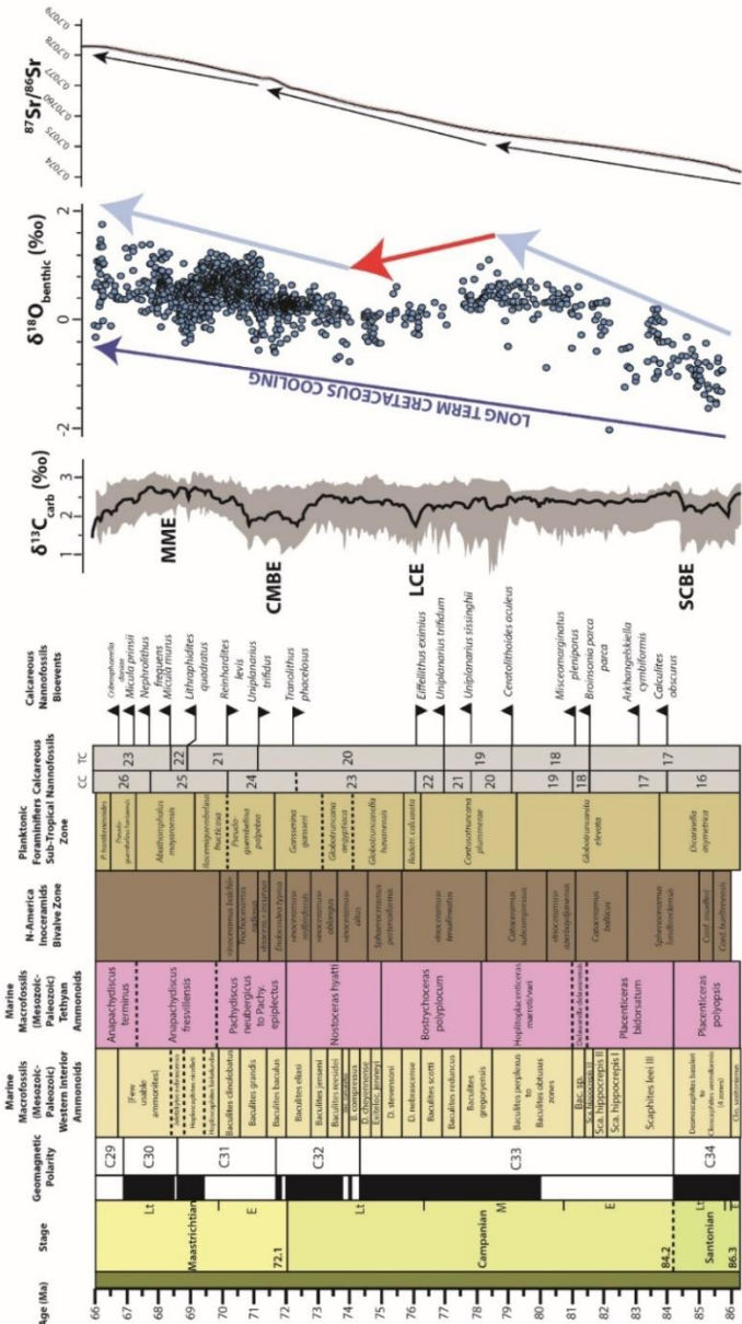
Figure 2 : Cadre stratigraphique du Santonien-Campanien-Maastrichtien, d’après la GTS 2012 et 2016 (Gradstein et al., 2012 ; Ogg et al., 2016), comparé à la compilation des données géochimiques du δ 13 C de la roche totale de Wendler (2013), du δ 18 O des foraminifères benthiques de Friedrich et al. (2012) et du 87 Sr/ 86 Sr de McArthur et al., 1993 recalculé sur le modèle d’âge
