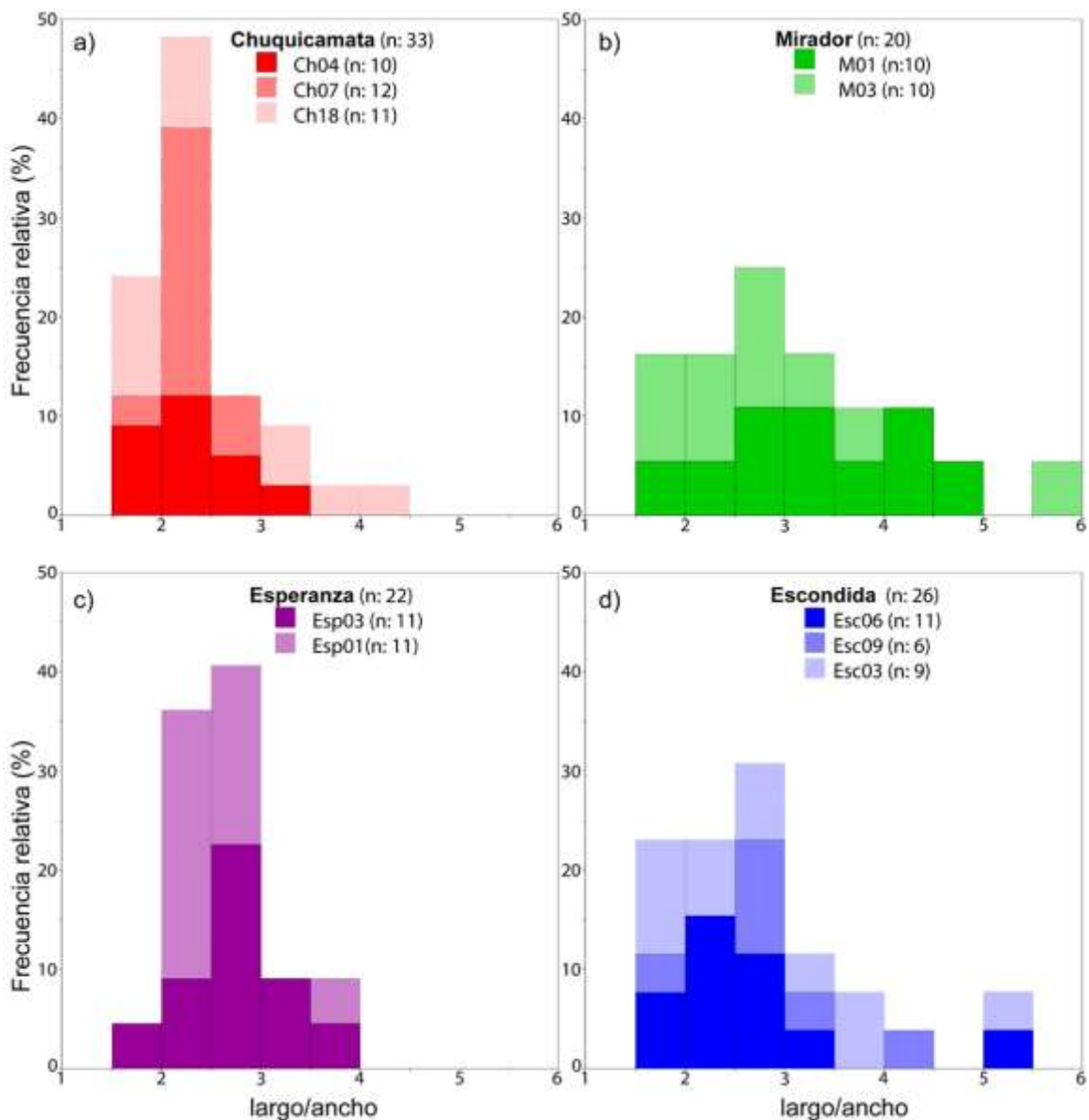
Figura 3.2 Histogramas de relación de aspecto (largo/ancho) de los circones provenientes de DPCs. a) Chuquicamata, b) Mirador; c) Esperanza; d) Escondida. n, numero de cristales medidos.
