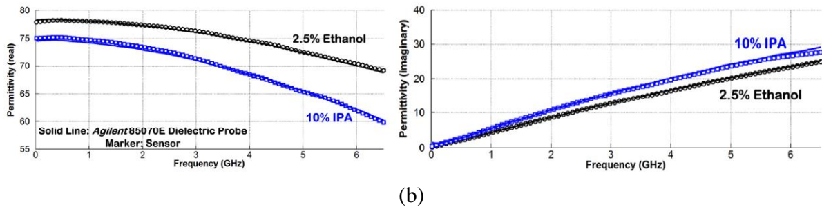
Figure I. 14. (a) Courbes d'étalonnage (b) parties réelles et imaginaires de la permittivité en fonction de la fréquence de 14 MHz à 6,5 GHz mesurées pour l'éthanol et l'alcool isopropylique [52].
