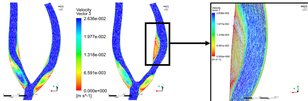
Fig. 3 : Streamlines de vitesse dans un section plane de la carotide avec et sans plaque
