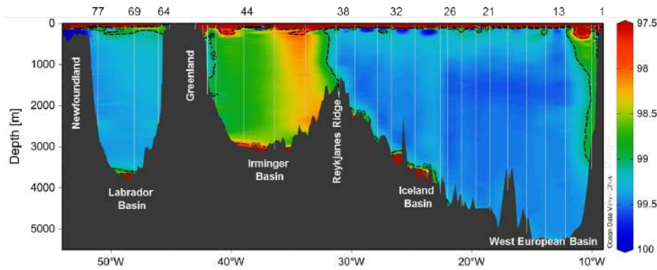
FIGURE 3.12 – Distribution de la transmissivité(en haut) le long de la section GEOVIDE. Les numéros des stations étudiées dans cette thèse se trouvent en haut de la figure. Les traits gris représentent les stations où la transmissivité a été mesurée.
