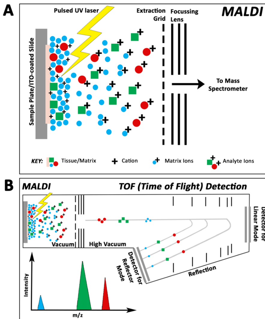
Figure 21: Principe de fonctionnement d'un appareil MALDI-TOF (Lakshini, 2016)
