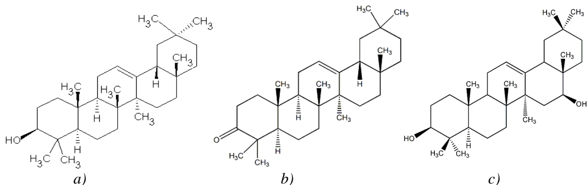
Figure 27: Structures moléculaires des triterpènes pentacycliques majoritaire d'Okoumé : a = \beta -amyrine b = \beta -amyrenone et c = maniladiol
