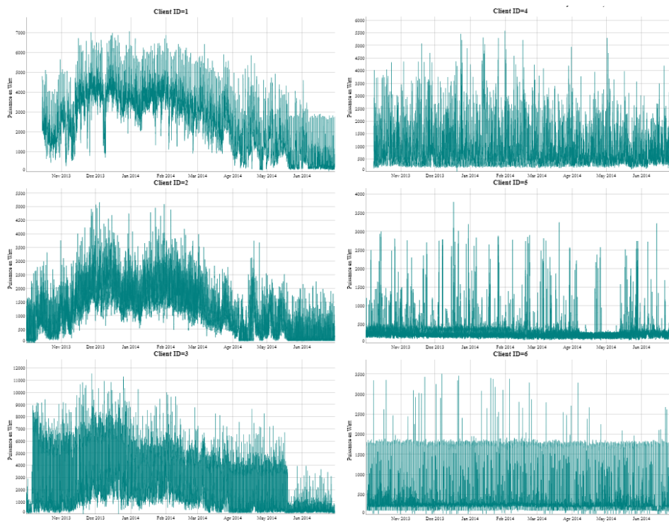
Figure 1.3 : Client thermo-sensible (à gauche) et non thermo-sensible (à droite).
