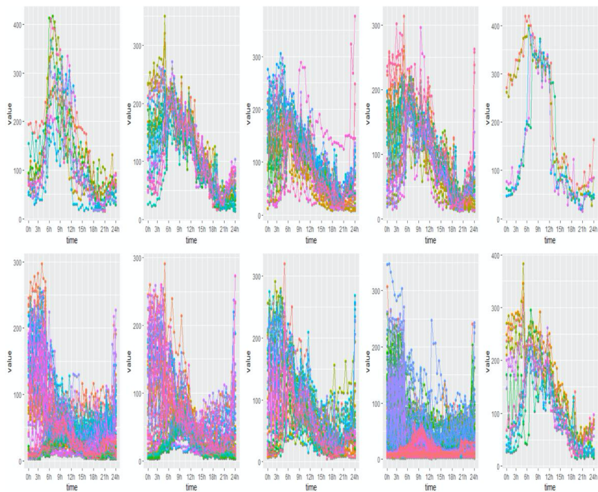
Figure 4.6 : Classification intra-journalière de la courbe de charge d'une entreprise A selon les hautes fréquences (l'échelle j = 1 ).
