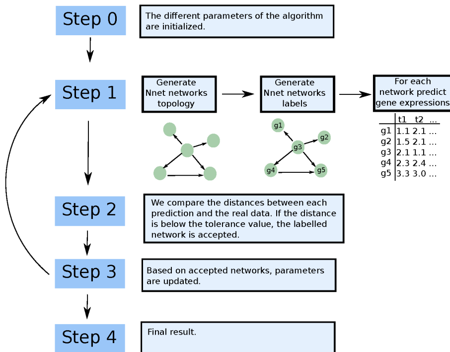
Figure 1.9 : Algorithme ABC pour l'inférence de réseau biologique.
