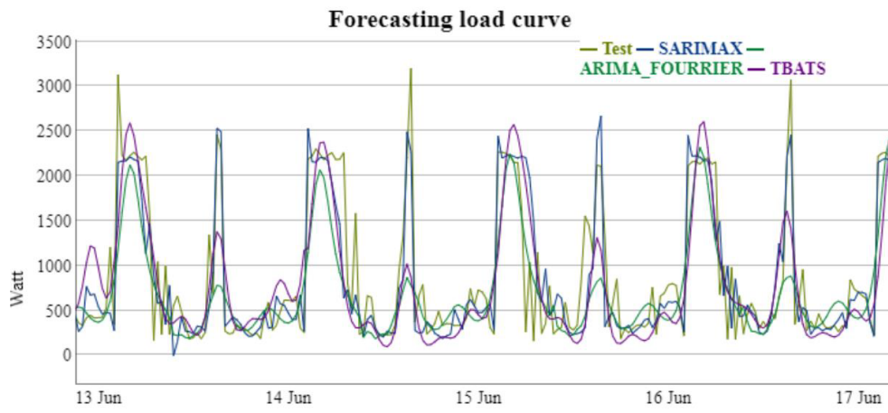
Figure 1.4 : Résultats préliminaires de prévision.
