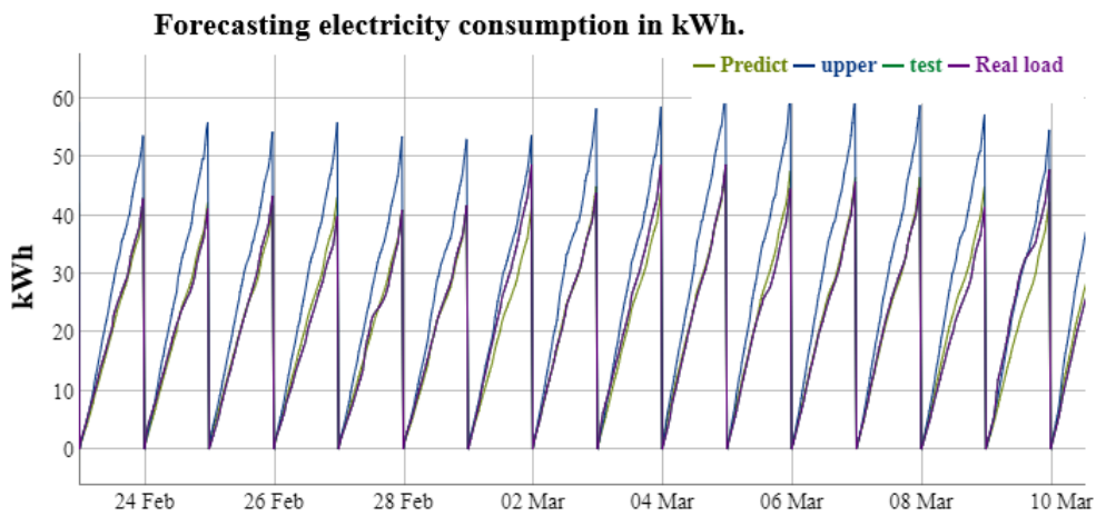
Figure 1.6 : Énergie journalière consommée en fonction du temps.
