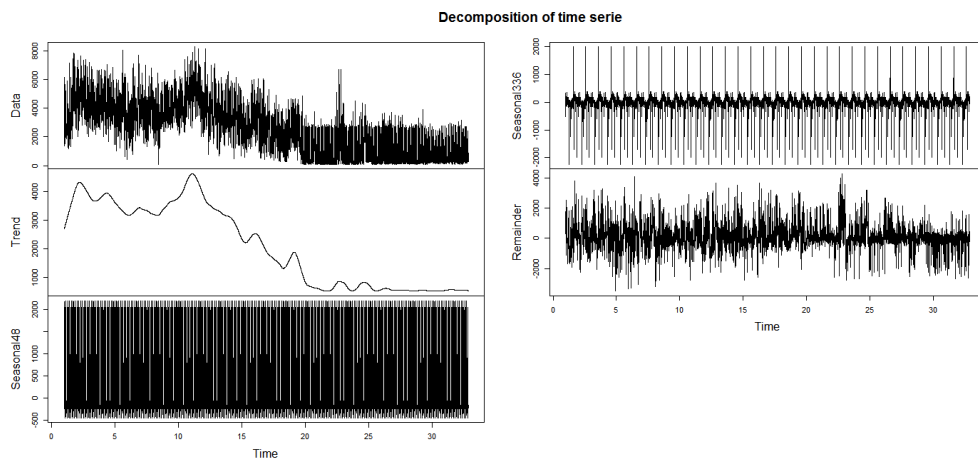
Figure 1.2 : La décomposition d'une courbe de charge d'un client montre les deux saisonnalités hebdomadaire (seasonal 336) et journalière (seasonal 48).
