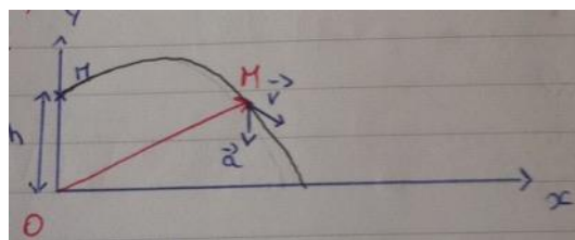
Figure 2-5 – Exemple de réponse contenant l'erreur « écart tangente » sur le vecteur vitesse
