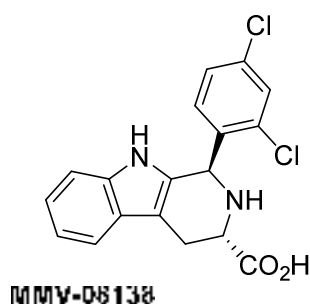
Figure 33 : Inhibiteur de l'IspD chez P. falciparum .
