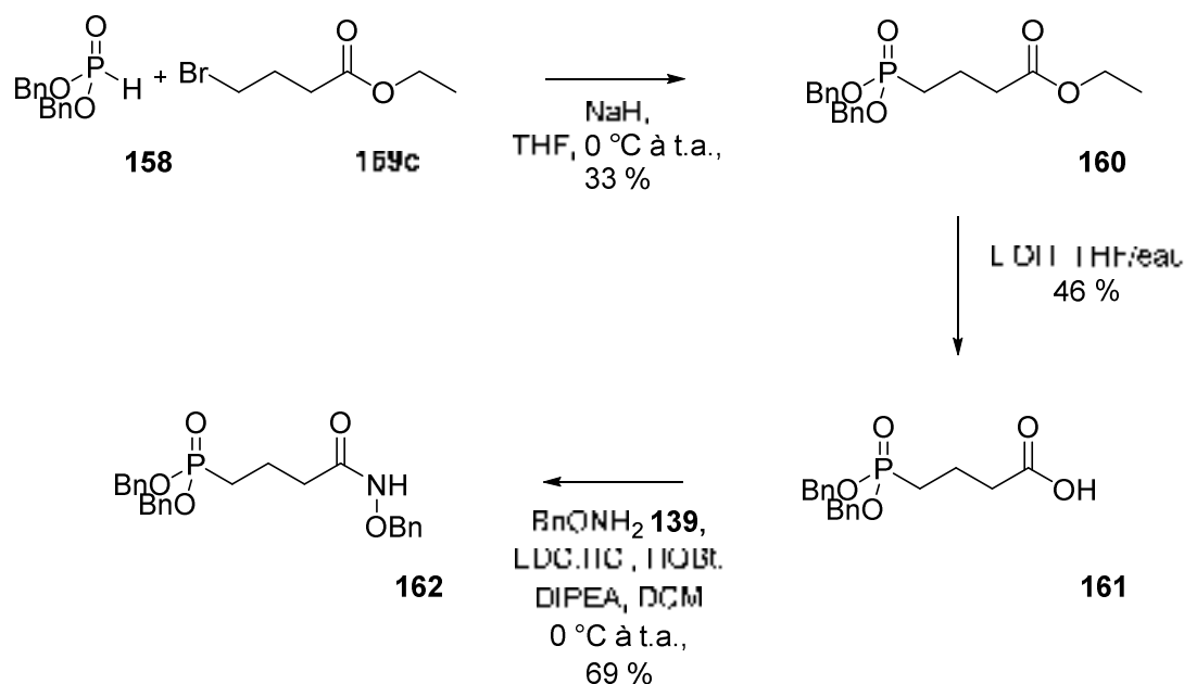
Figure 115 : Synthèse du phosphono hydroxamate 162 .
