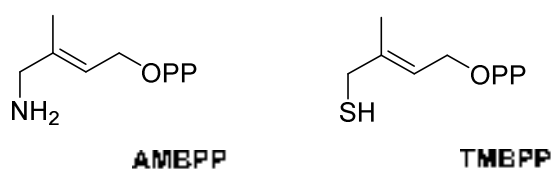
Figure 58 : Inhibiteurs de l'IspH.
