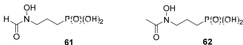
Figure 59 : Fosmidomycine 61 et son analogue méthylé le FR-900098 62 .
