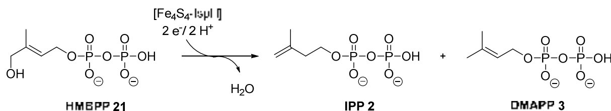
Figure 55 : Etape catalysée par l'IspH.
