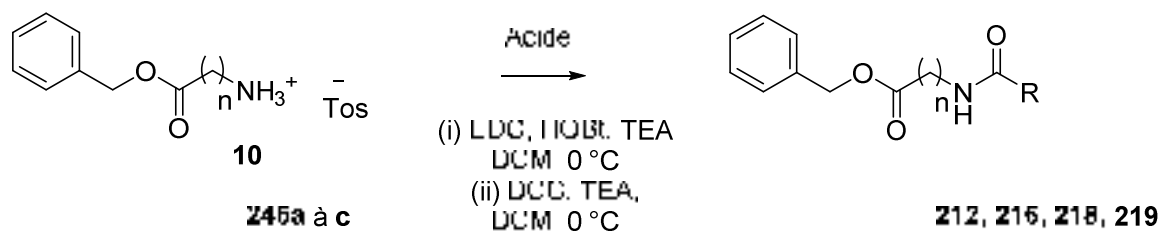
Figure 158 : Test de couplage de type peptidique avec les aminoacides protégés.
