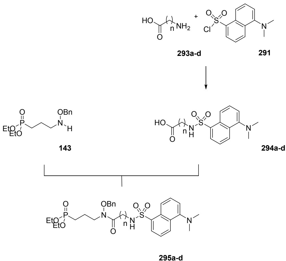
Figure 180 : Stratégie de synthèse convergente.
