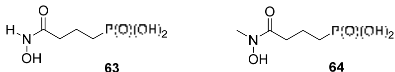
Figure 114 : Inhibiteurs en pince dite inversée.
