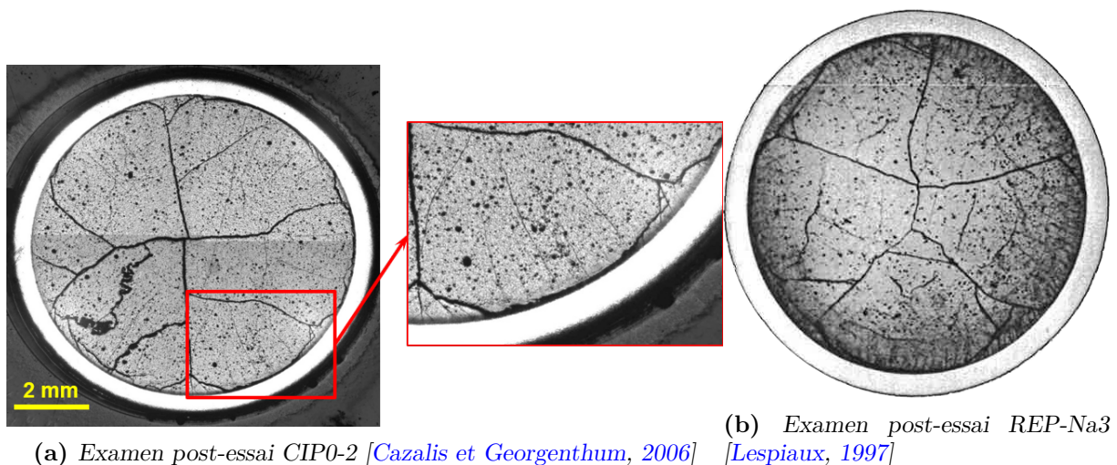
Figure 50 – Micrographie d'une tranche d'un crayon combustible après un essai d'insertion de réactivité. Observations de fissures radiales primaires formées en conditions nominales et de fissures radiales secondaires en périphérie pouvant être dues au transitoire rapide de puissance.
