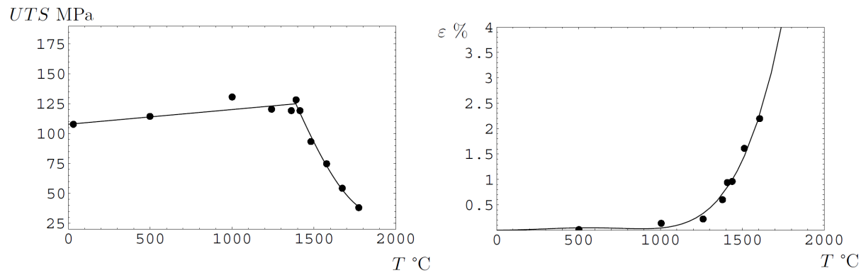
Figure 7 – Résultats d’essais de Canon et al. [1971] , flexion de l’UO 2 vierge avec une porosité de fabrication 3%, et une taille de grain de 8 μm (figures tirées de Vincent [2007] ). Mise en évidence d’un comportement fragile à basse température et ductile à haute température. ε% : déformation plastique totale.
