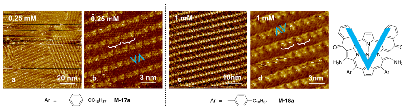
Figure 13. Images STM des assemblages de M-17a et M-18a à l'interface HOPG-phényloctane, a) I = 1,0 pA et V = -900 mV, b) I = 1,0 pA et V = -622 mV, c) I = 1,1 pA et V = -103 mV, d) I = 1,2 pA et V = -164 mV
