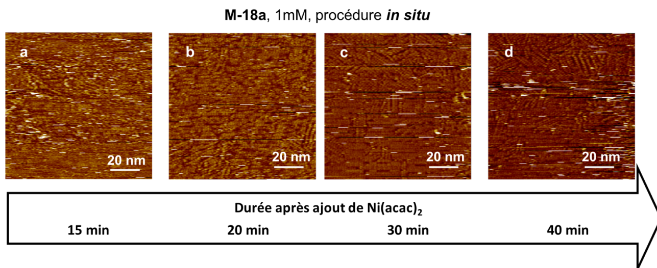
Figure 26. Images STM des assemblages des oligomères de M-18a en fonction du temps, après ajout de \text{Ni}(\text{II}) , en in situ , à l'interface HOPG-phényloctane, a) I = 1,8 \text{ pA} et V = -841 \text{ mV} , b) I = 1,8 \text{ pA} et V = -841 \text{ mV} , c) I = 1,6 \text{ pA} et V = -1184 \text{ mV} , d) I = 1,6 \text{ pA} et V = -1184 \text{ mV}
