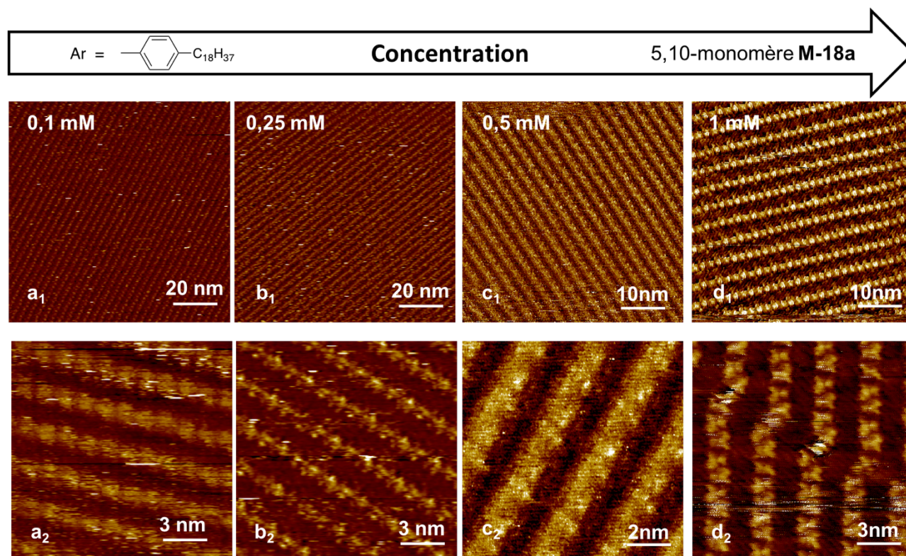
Figure 17. Images STM des assemblages M-18a à l'interface HOPG-phényloctane, à différentes concentrations, a_1 ) I = 2,0 \text{ pA} et V = -220 \text{ mV} , a_2 ) I = 1,8 \text{ pA} et V = -1226 \text{ mV} , b_1 ) I = 1,8 \text{ pA} et V = -244 \text{ mV} , b_2 ) I = 3,5 \text{ pA} et V = -346 \text{ mV} , c_1 ) I = 1,0 \text{ pA} et V = -51 \text{ mV} , c_2 ) I = 1,0 \text{ pA} et V = -115 \text{ mV} , d_1 ) I = 1,1 \text{ pA} et V = -103 \text{ mV} , d_2 ) I = 2,0 \text{ pA} et V = -487 \text{ mV}
