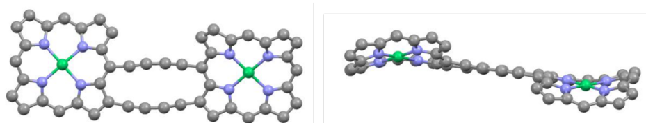
Figure 18. Structure (diffraction des rayons X) de I-40 (générée à partir des données de la base CCDC), les groupements 3,5- t\text{Bu}_2\text{Ph} ont été omis pour plus de clarté [63]
