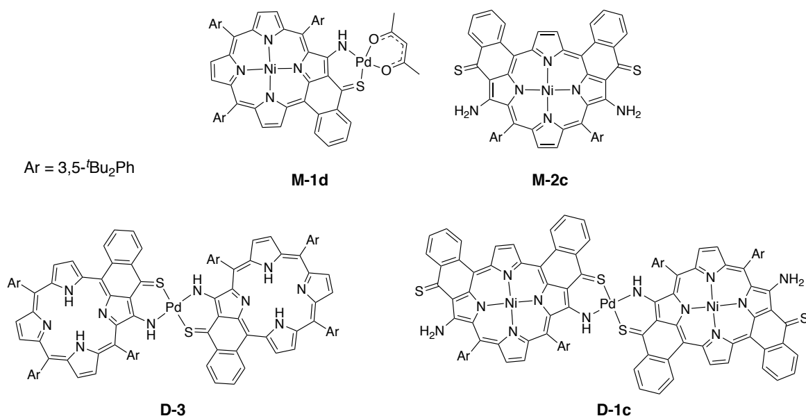
Figure 27. Rappel M-1d, M-2c, D-3 et D-1b
