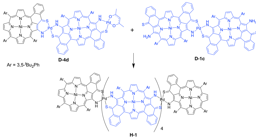
Schéma 15. Schéma de synthèse de l'hexamère
