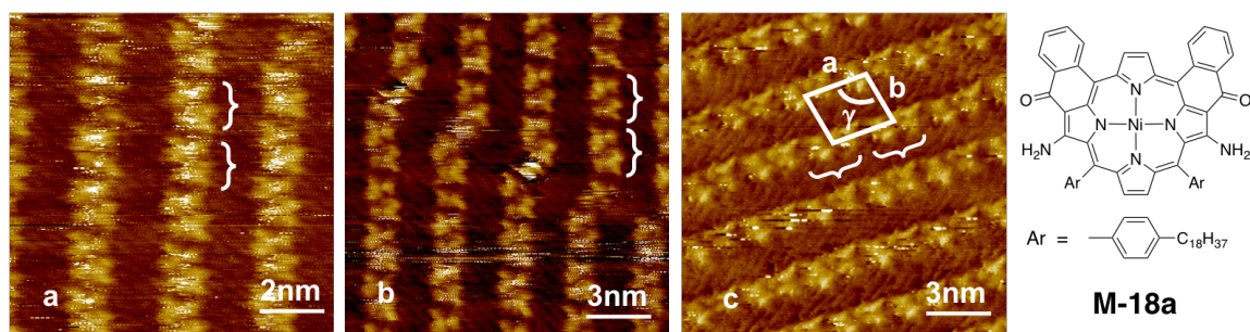
Figure 14. Images STM des assemblages M-18a à l'interface HOPG-phényloctane, 1mM, a) I = 2,0 pA et V = -487 mV, b) I = 2,0 pA et V = -487 mV, c) I = 1,2 pA et V = -164 mV
