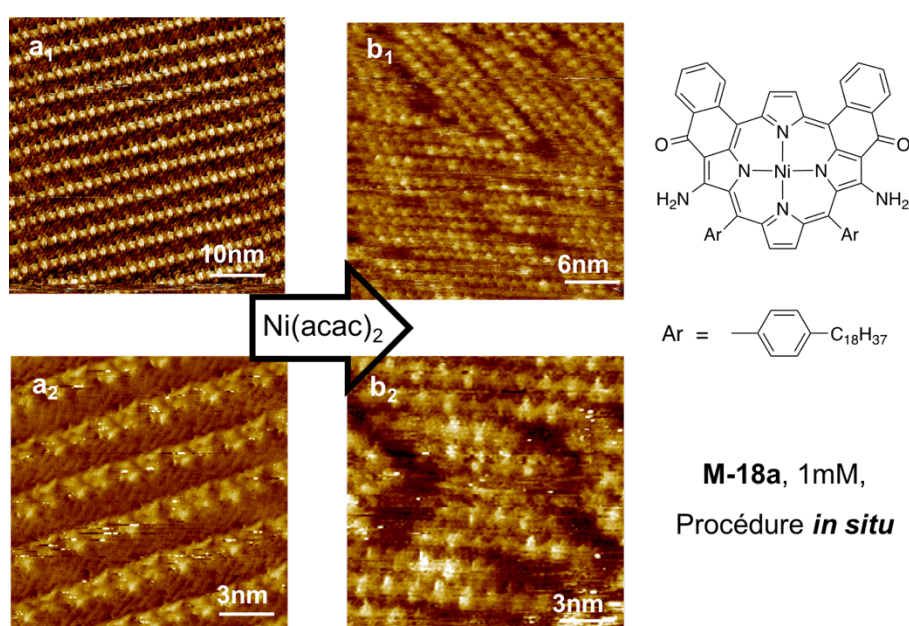
Figure 25. Images STM des assemblages des oligomères de M-18a après ajout de Ni(II), en in situ , à l'interface HOPG-phényloctane, conditions STM : I = 1,4 \text{ pA} et V = -818 \text{ mV}
