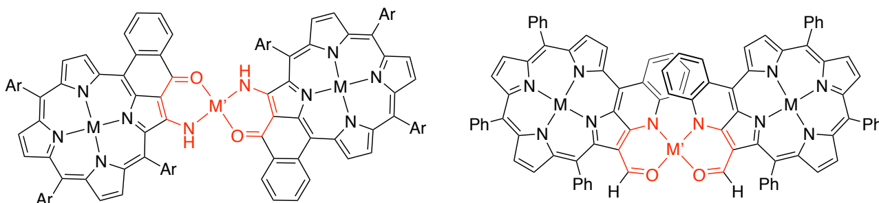
Figure 36. Dimères de porphyrines liés par un cation métallique (gauche : énaminocétone externe, géométrie trans – droite : énaminaldéhyde externe, géométrie cis )
