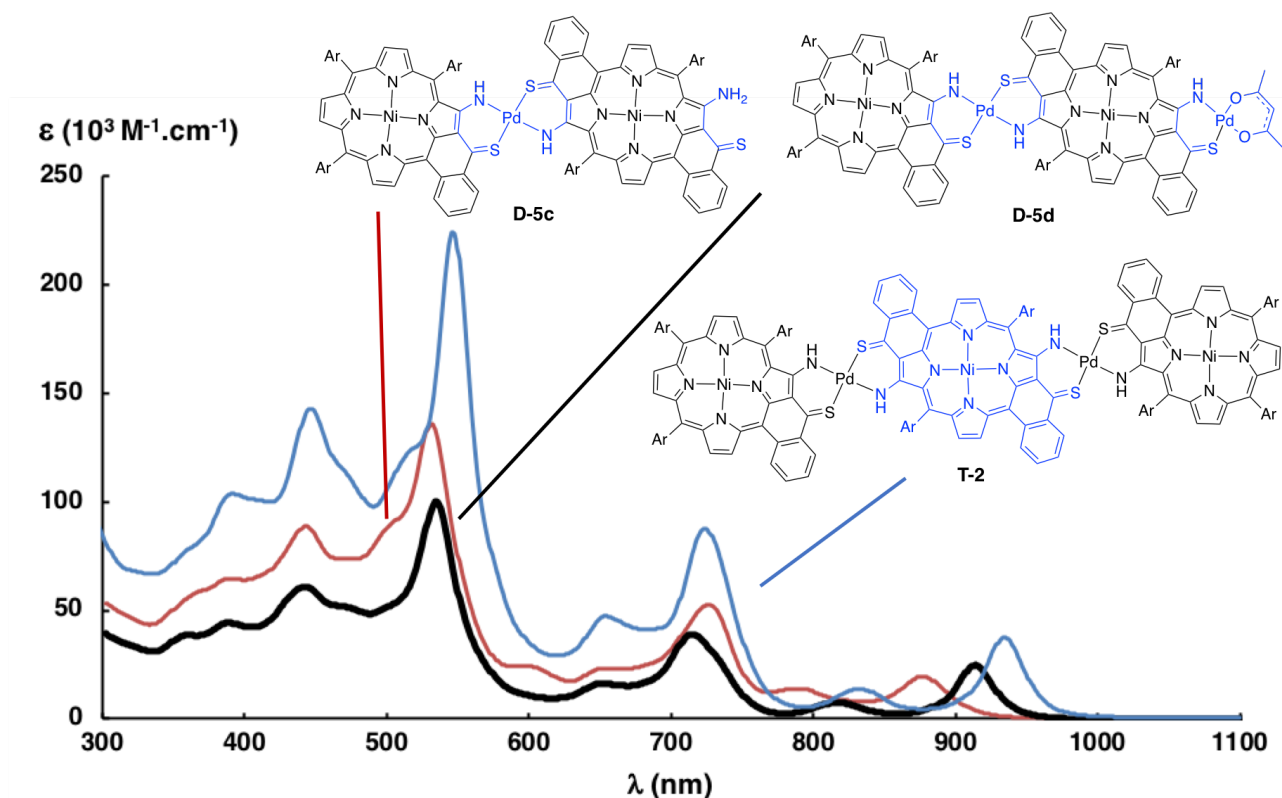
Figure 20. Spectres électroniques de T-2 , D-5c et D-5d
