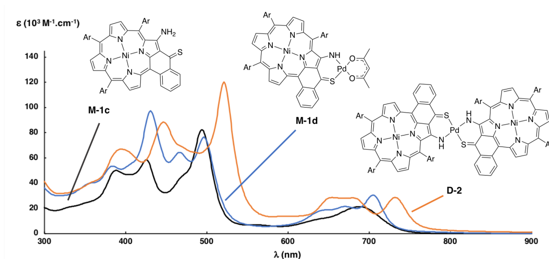
Figure 12. Spectres électroniques de M-1c , M-1d et D-2
