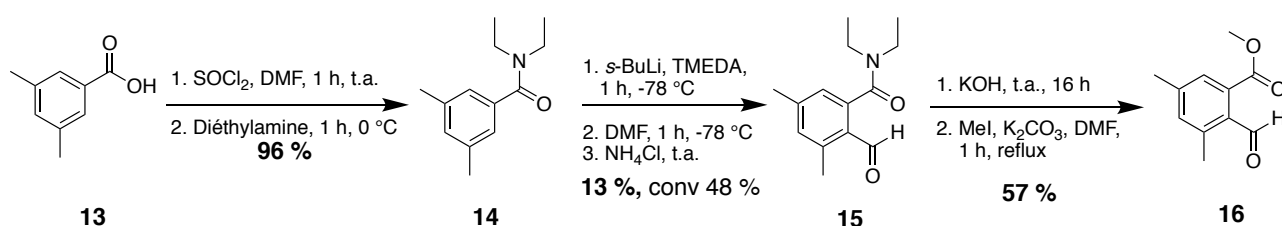
Schéma 9. Synthèse du composé 16
