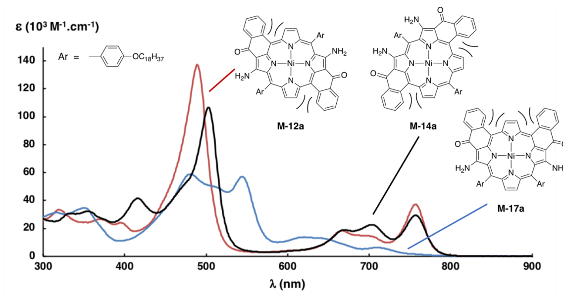
Figure 4. Spectres électroniques de M-12a , M-14a et M-17a
