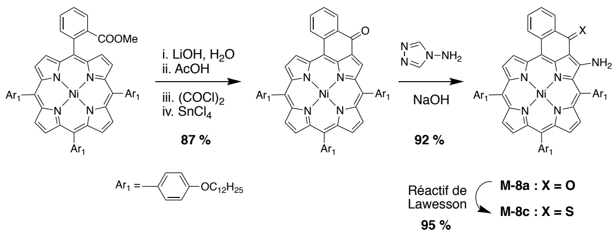
Schéma 3. Synthèse du monomère M-8c
