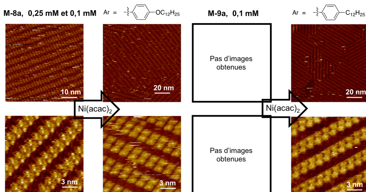
Figure 19. Organisation à l'interface HOPG-phényloctane, avant et après ajout de Ni(acac) 3 pour M-8a et M-9a
