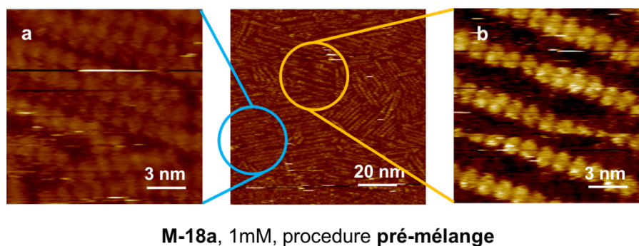
Figure 28. Images STM des assemblages des oligomères de M-18a en fonction du temps, après ajout de Ni(II), en pré-mélange, à l'interface HOPG-phényloctane, conditions STM : I = 3,7 \text{ pA} et V = -1111 \text{ mV}
