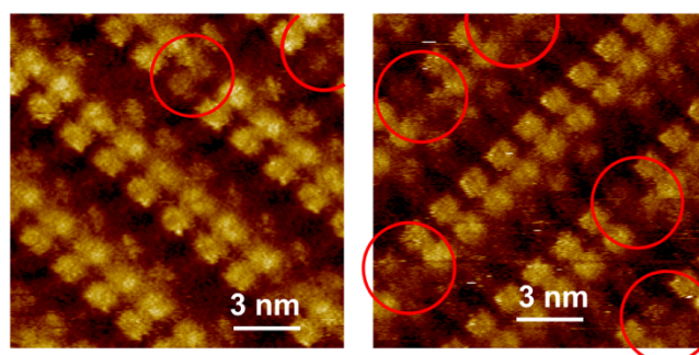
Figure 23. Lacunes dans l'assemblage de dimères de M-10a à l'interface HOPG-phényloctane, 0,1mM
