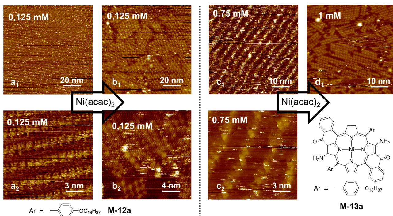
Figure 19. Images STM des assemblages des oligomères de M-12a ( b_1 et b_2 ) et M-13a ( d_1 ), après ajout in situ de \text{Ni}(\text{II}) , à l'interface HOPG-phenyloctane, b_1 ) I = 1,0 pA et V = -1000 mV, b_2 ) I = 1,3 pA et V = -1000 mV, d_1 ) I = 1,3 pA et V = -404 mV
