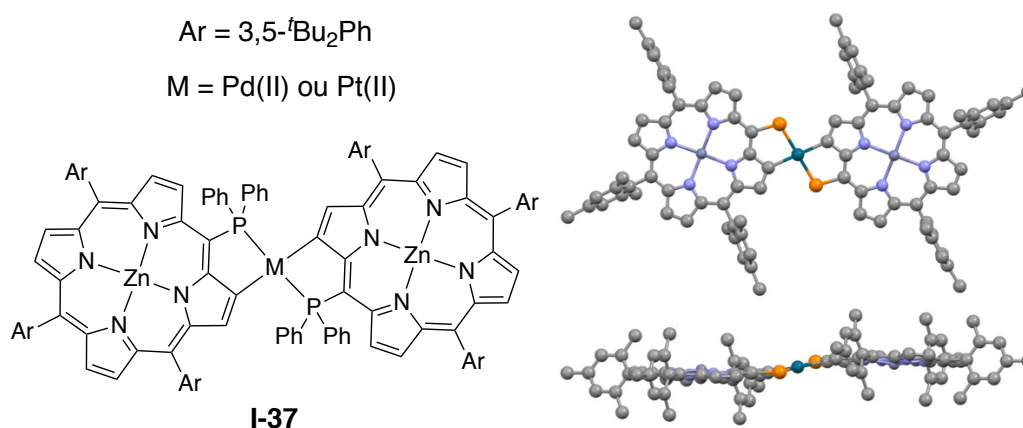
Figure 35. Porphyrines directement liées par un cation métallique en position \beta , structure générée en utilisant les données de la base CCDC (deux vues orthogonales) [104]
