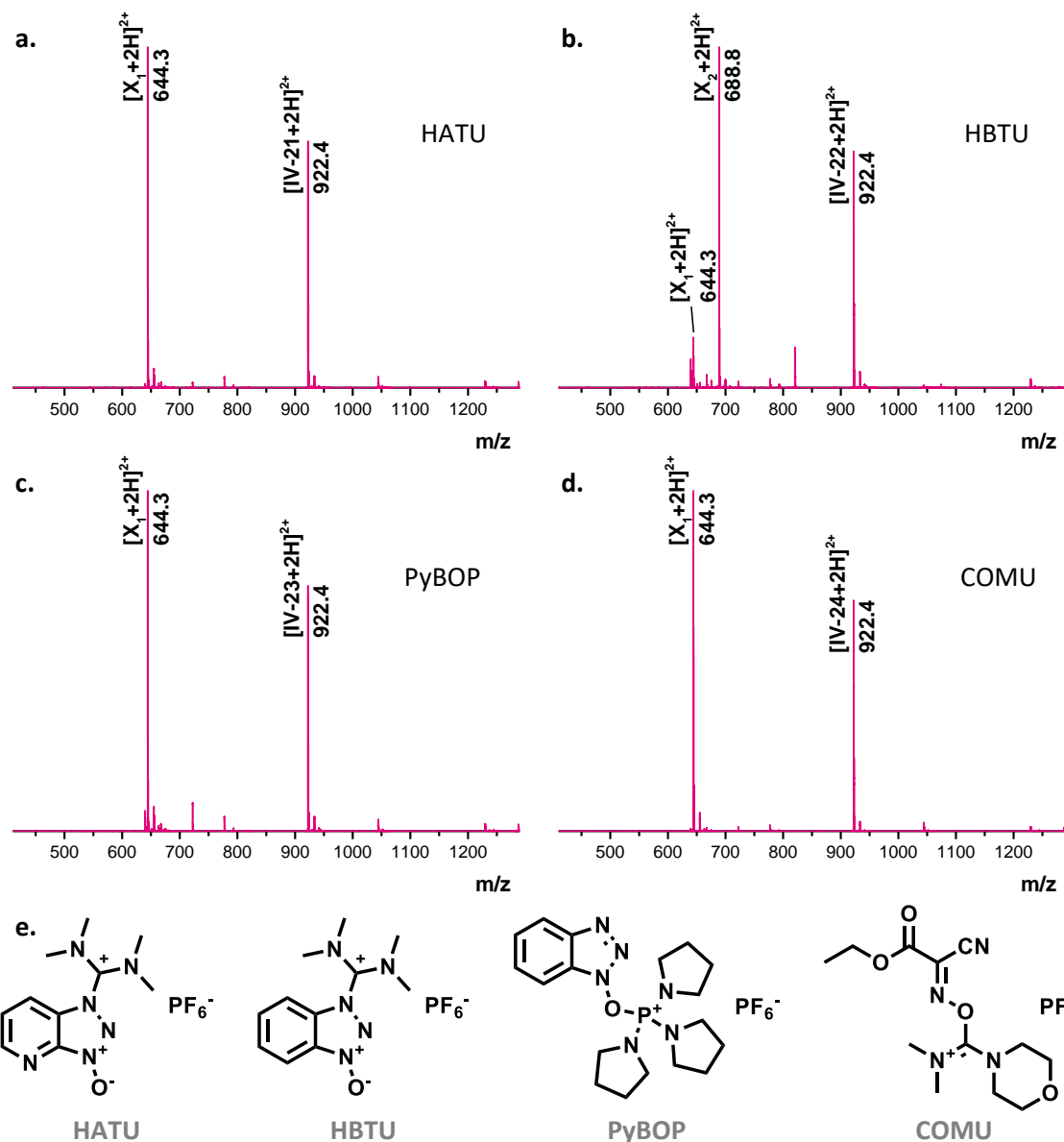
Figure IV.17. Spectres ESI-HRMS de la séquence de PTzNA [Phe-TTTTAT] synthétisée avec différentes conditions pour l'ajout du bloc AB-A. a. Agent de couplage pour l'addition de bloc AB-A : HATU (IV-21). b. Agent de couplage pour l'addition de bloc AB-A : HBTU (IV-22). c. Agent de couplage pour l'addition de bloc AB-A : PyBOP (IV-23). d. Agent de couplage pour l'addition de bloc AB-A : COMU (IV-24). e. Structure des différents agents de couplage utilisés.
