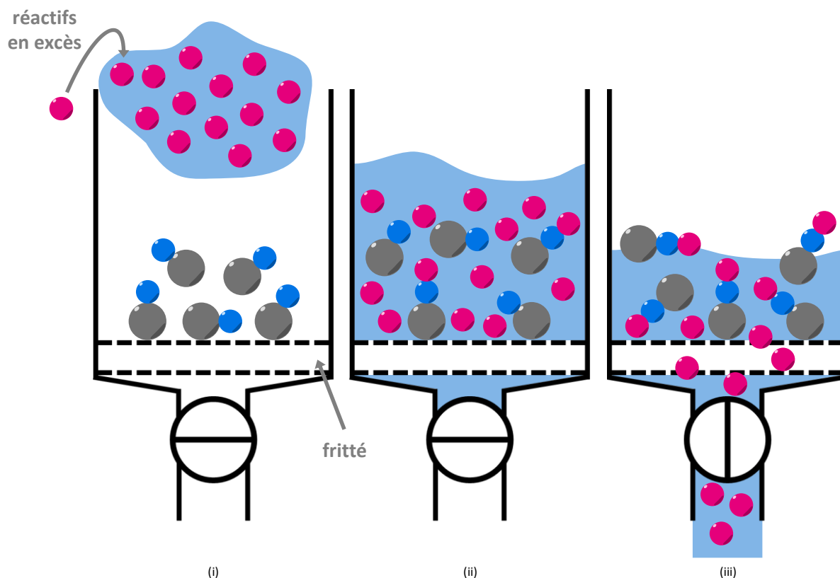
Figure I.10. Protocole général pour la synthèse itérative sur support solide. (i) Ajout des réactifs en solution en excès. (ii) Couplage. (iii) Purge et lavage par filtration avec les solvants adéquats. Les différentes étapes peuvent alors être répétées.
