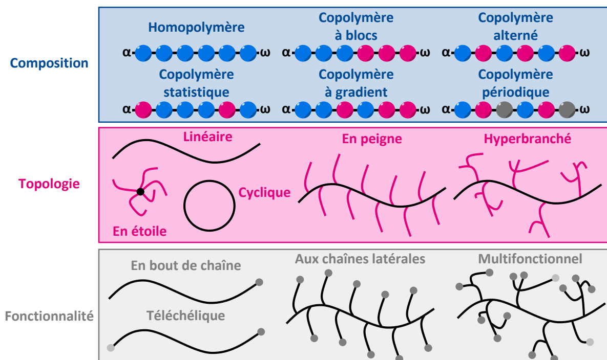
Figure I.1. Guide (non exhaustif) des trois aspects principaux de l'architecture macromoléculaire : la composition, la topologie et la fonctionnalité. [3]
