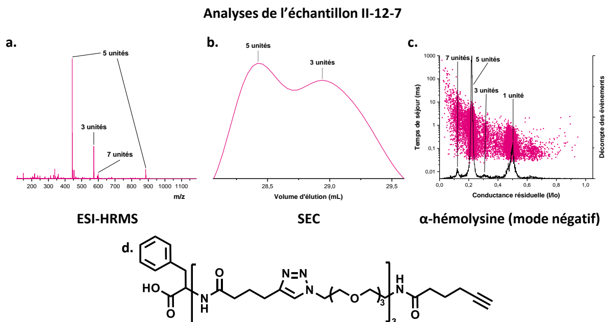
Figure II.22. Corrélation entre les analyses ESI-HRMS (a), SEC (b) et avec l' \alpha -hémolysine (c) de l'échantillon contenant le composé II-12-7 (d).
