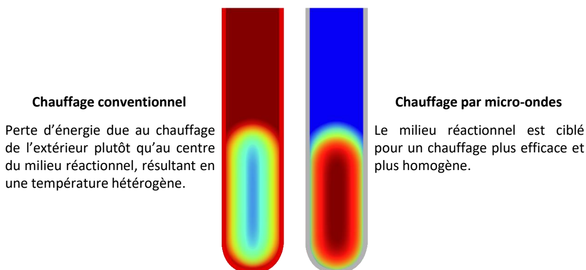
Figure II.10. Principe du chauffage par micro-ondes. Les teintes bleues réfèrent à des températures basses tandis que les teintes rouges dénotent des températures élevées.
