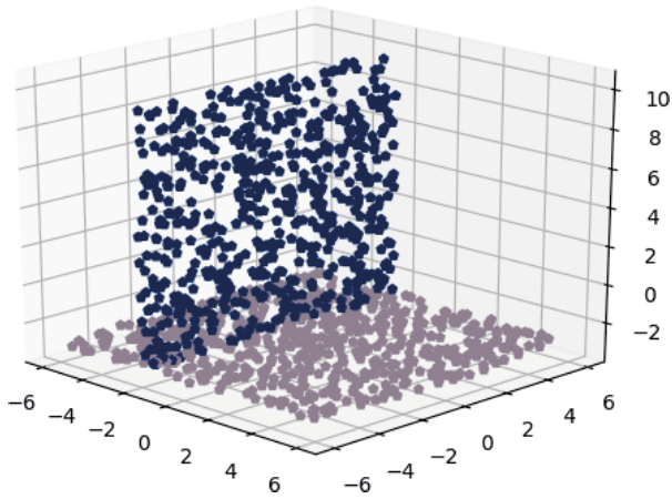
(a) Deux plans identifiés par l'algorithme Prosecco
