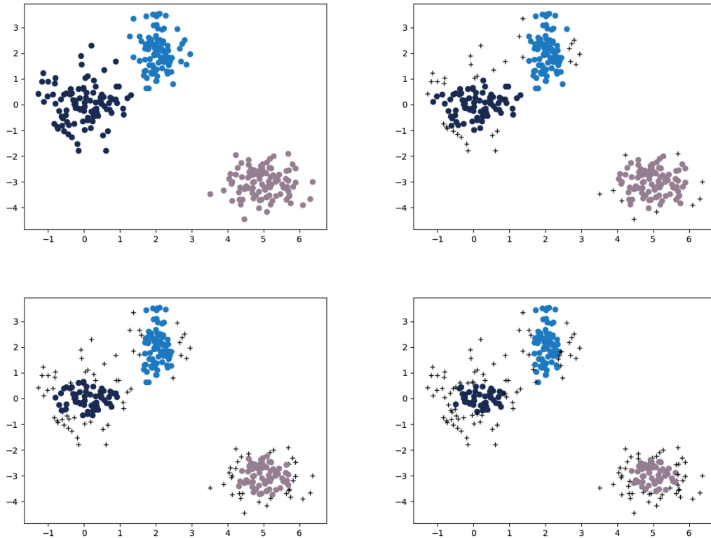
FIG. 5.3 : Application de l'algorithme Possecco et équetage du résultat pour \eta \in \{0, 0,3, 0,6, 0,9\} .
