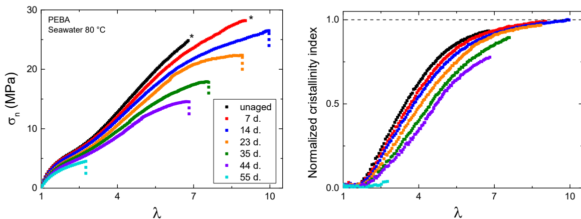
Figure R10 – Effet du vieillissement (immersion en eau de mer à 80°C) sur le PEBA, courbe de traction (gauche) et indice de cristallinité normalisée (droite). L'indice de cristallinité maximum atteint est de 40 %.
