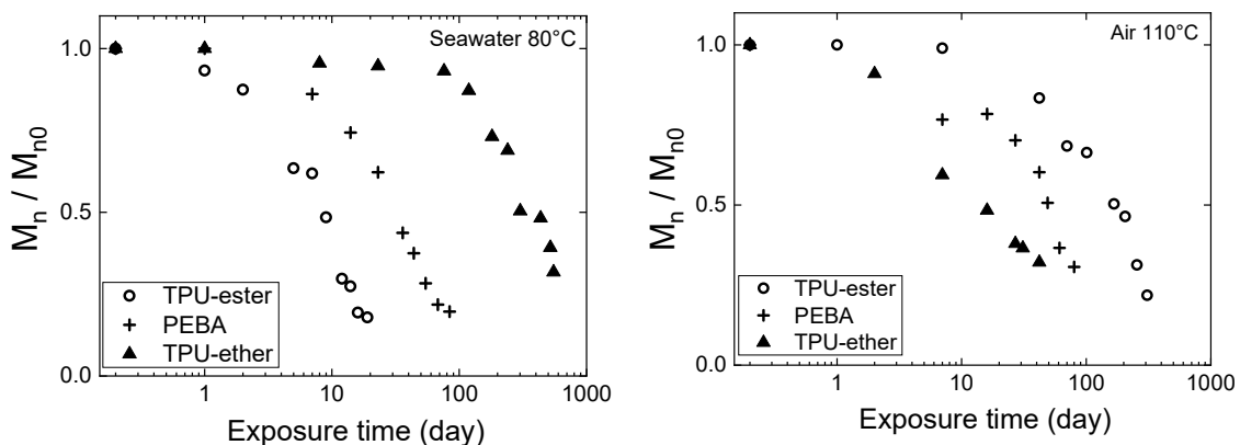
Figure R6 – Diminution de masse molaire présentée par tous les TPEs. Cas de l'immersion en eau de mer à 80°C (gauche) et de l'exposition à l'air à 110°C (droite).
