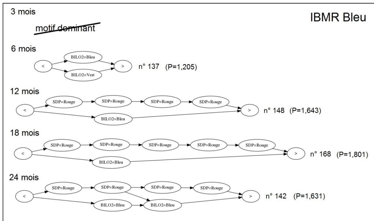
Figure 49 : Motifs extraits pour le contexte IBMR en très bon état, choisis parmi les 5 motifs sélectionnés sur la base de leur combinaison P (indiquée entre parenthèses) la plus élevée, pour les longueurs de séquences 3, 6, 12, 18 et 24 mois, avec les grilles DCE
