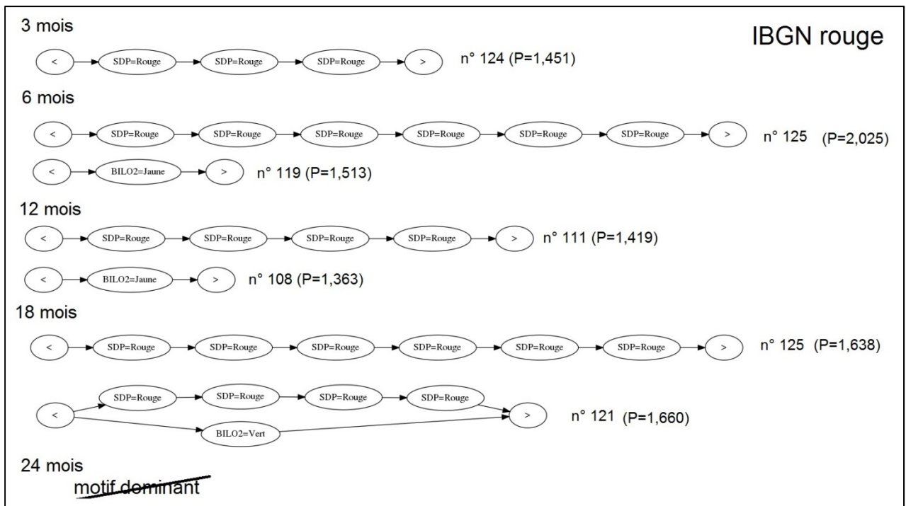
Figure 52 : Motifs extraits pour le contexte IBGN en mauvais état, choisis parmi les 5 motifs sélectionnés sur la base de leur combinaison P (indiquée entre parenthèses) la plus élevée, pour les longueurs de séquences 3, 6, 12, 18 et 24 mois, avec les grilles DCE
