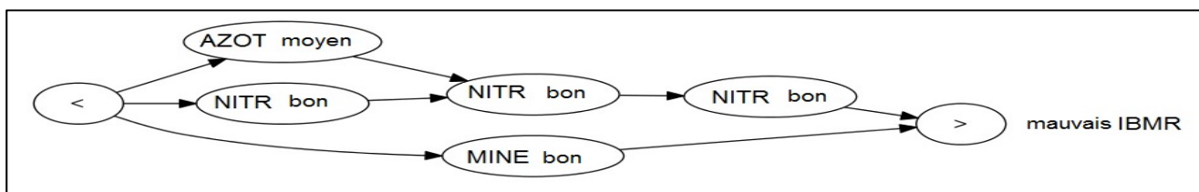
Figure 15 : Motif numéro 442 ayant précédé un IBMR en mauvais état (critères d'extraction : toute la France, période 2007-2013, SEQ-eau, longueur de séquence 24 mois, fréquence minimale 0,6) ; altérations AZOT : matières azotées hors nitrates et NITR : nitrates
