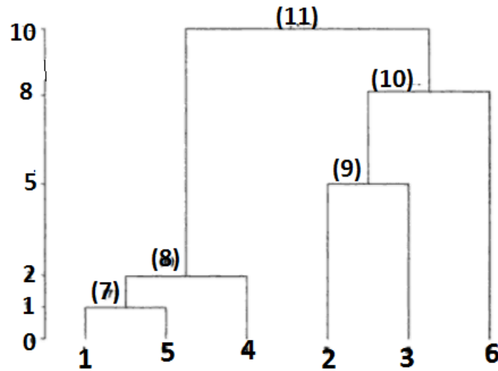
FIGURE 3.6 – Dendrogramme de la hiérarchie indiquée (H_E, v) où H_E est la hiérarchie de l'exemple 1 et v l'indice de niveau de l'exemple 2.
