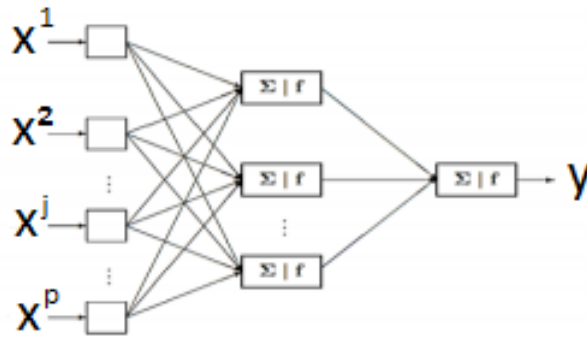
FIGURE 3.4 – Exemple de perceptron multicouche élémentaire avec une couche cachée et une couche de sortie.
