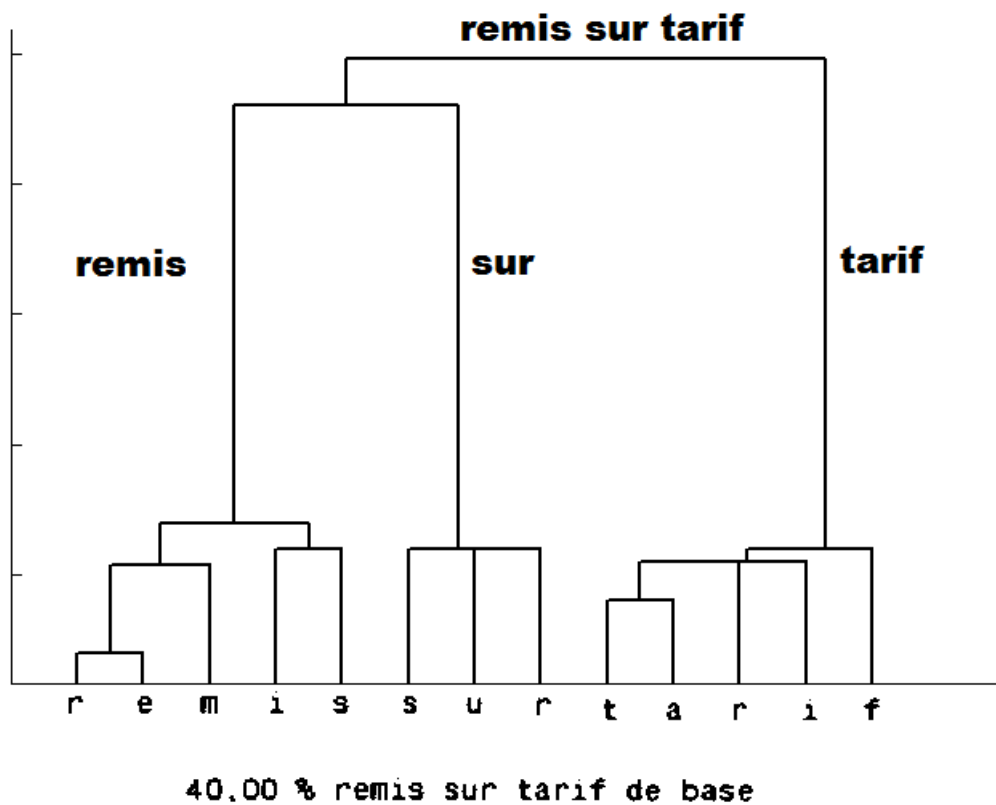
FIGURE 1.3 – Dendrogramme produit par l'algorithme DTMSEr. Les nœuds feuilles correspondent aux composants connectés de l'image, alors que les regroupements de nœuds dépendent uniquement de la distance entre régions, ce qui donne lieu à des groupes sémantiquement pertinents.
