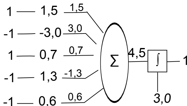
FIGURE 3.5 – Exemple de réseau de neurones pour la classification d’un ensemble de documents.
