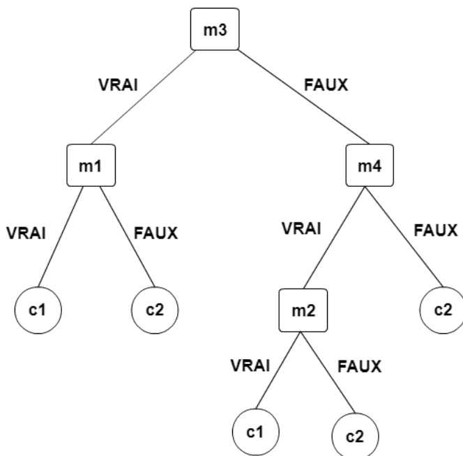
FIGURE 3.2 – Arbre de décision obtenu à partir des données d’entraînement de la Figure 3.1.
