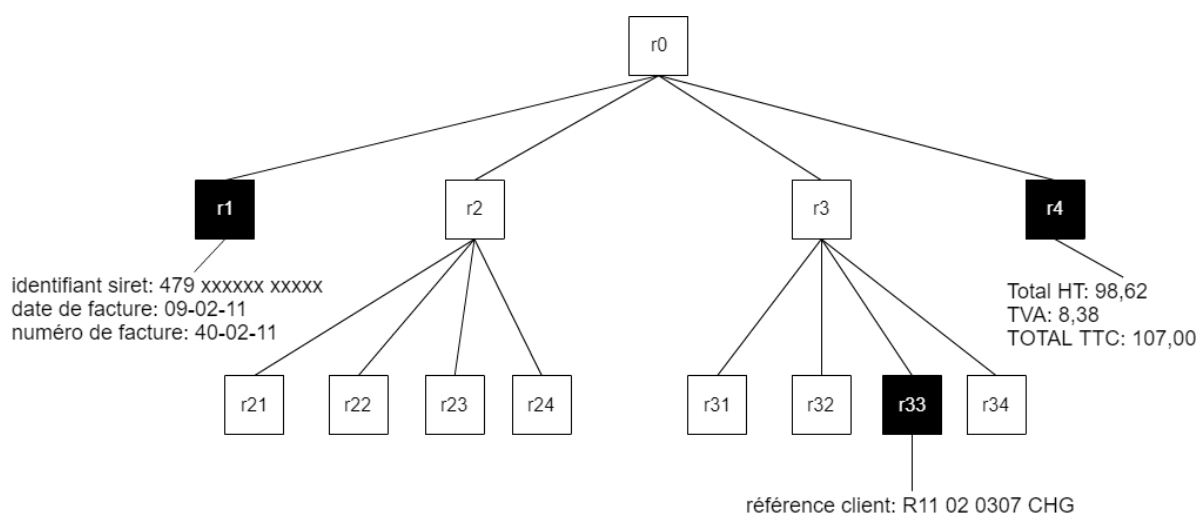
FIGURE 5.3 – Exemple de quadtree obtenu en appliquant notre algorithme sur une image de facture.
