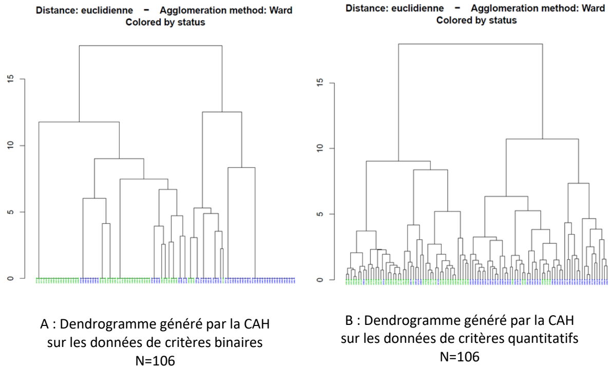
Figure 39 : Dendrogrammes issus des CAH réalisées sur les critères du SMet binarisés ou sous forme de valeurs quantitatives à T1. Coloration en fonction du statut (bleu = témoins; vert = cas).
