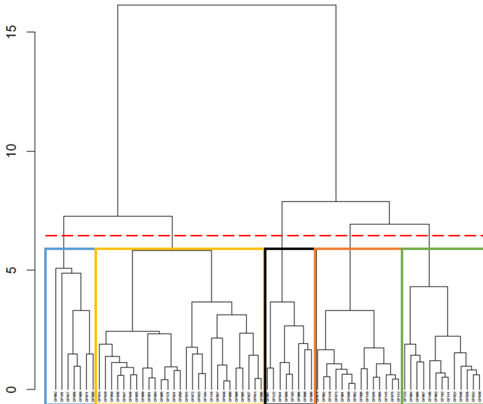
Figure 40 : Dendrogramme généré par la CAH sur les données de critères quantitatifs (nombre de sujets = 69).
