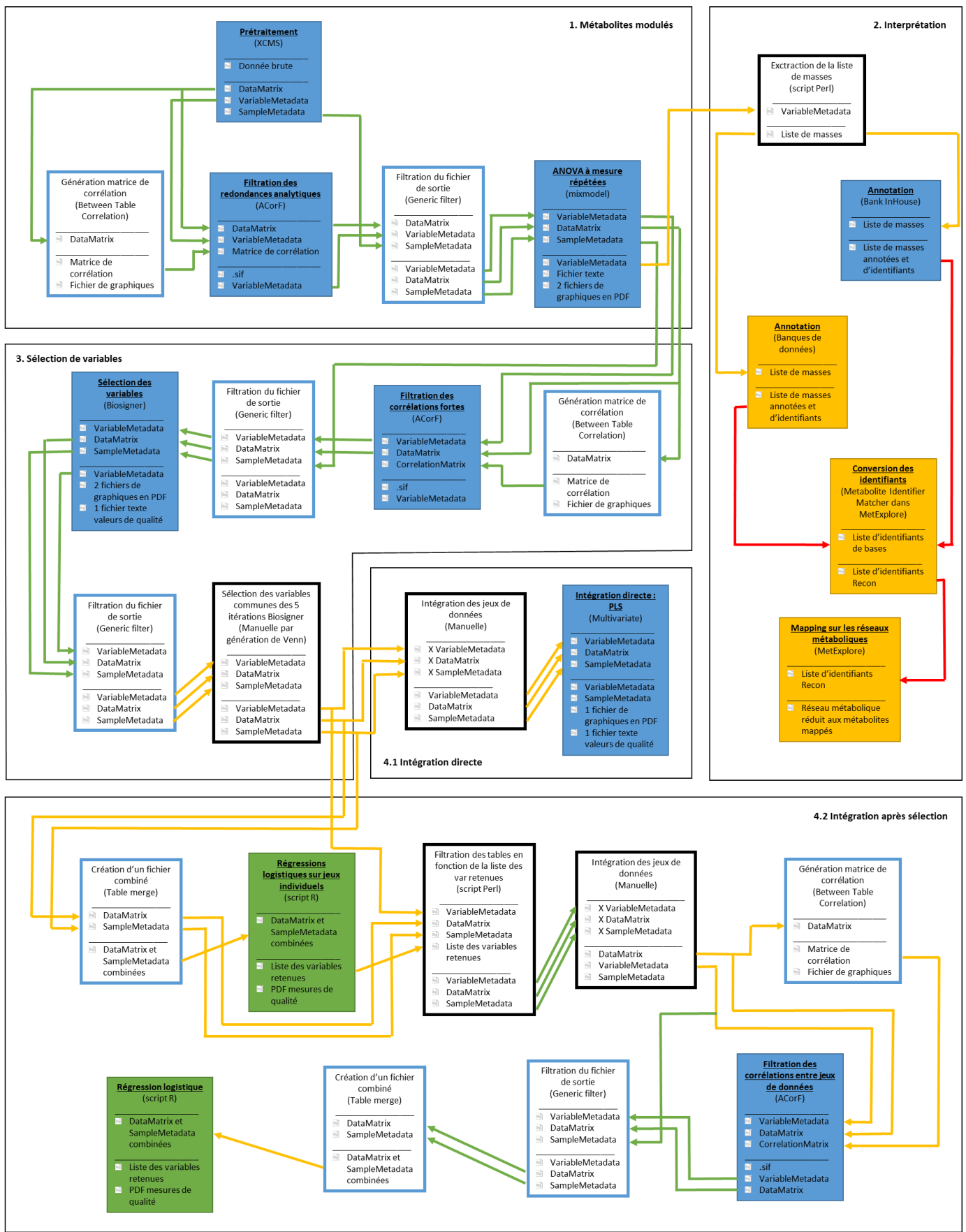
Figure 38 : Présentation générale du workflow d'analyse.
