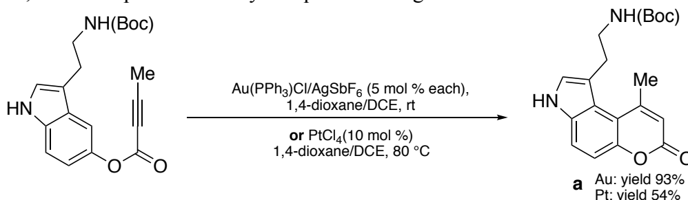
Scheme 21.
