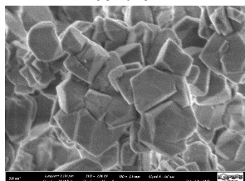
Zéolithe Y
