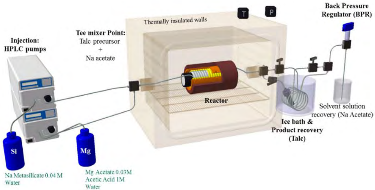
Figure 23 : Schéma du dispositif permettant la synthèse de talc en conditions supercritiques (Claverie et al. , 2018).
