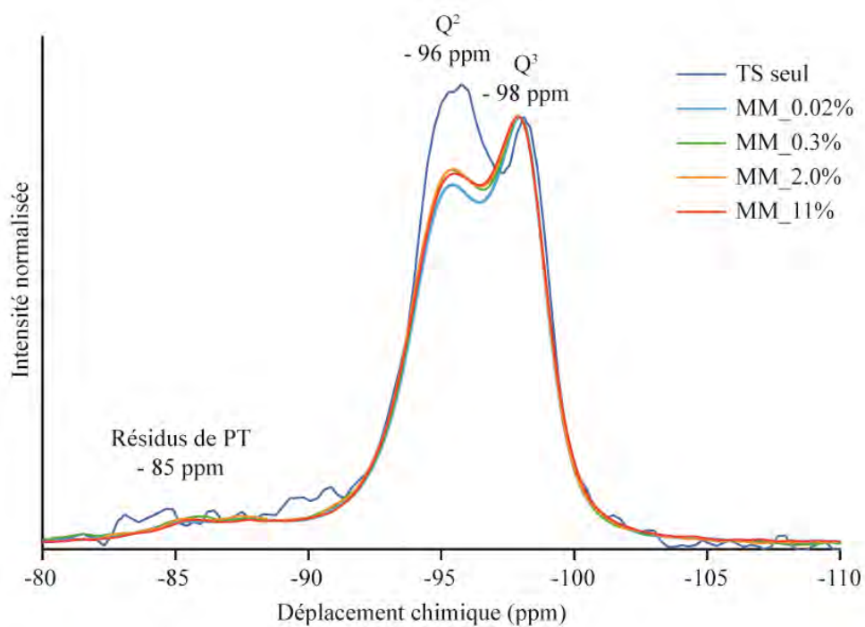
Figure 28 : Comparaison du spectre RMN ^{29}\text{Si} des échantillons hybrides élaborés avec le protocole MM (PT : Prototalc).
