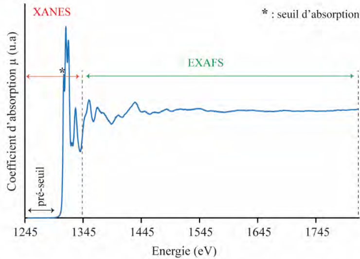
Figure 16 : Spectre XAS présentant l'évolution du coefficient d'absorption \mu en fonction de l'énergie E du faisceau de rayons X incident.
