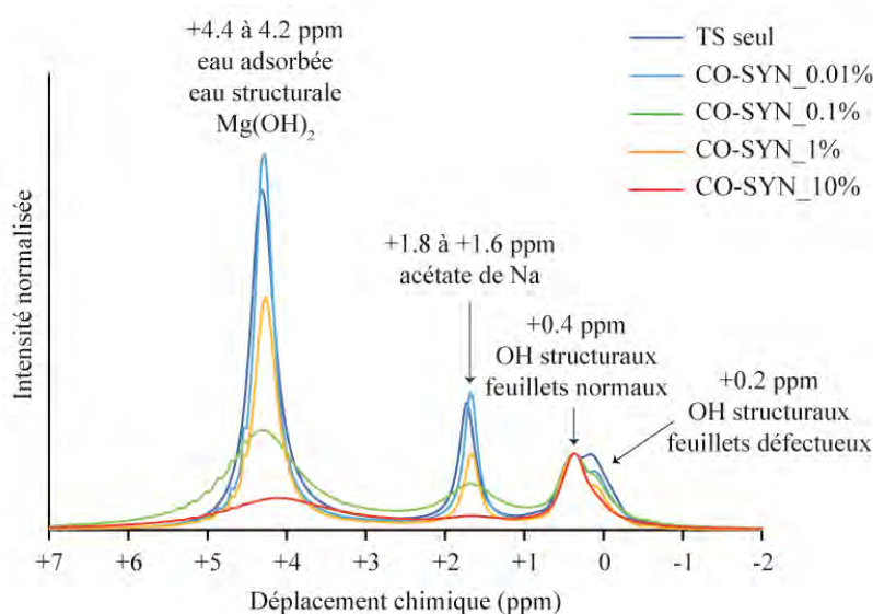
Figure 14 : Spectres RMN 1 H de la série d’échantillons CO-SYN enregistrés à une vitesse MAS de 45 kHz.
