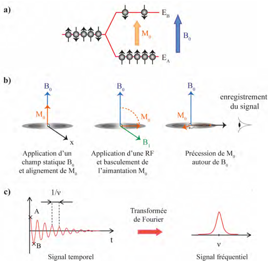
Figure 11 : Principe de la spectroscopie RMN : a) Séparation des moments magnétiques de spin sur deux niveaux d'énergie et formation d'une aimantation macroscopique résultante ( \vec{M}_0 ) ; b) Basculement et enregistrement du signal RMN ; c) Transformation du signal.
