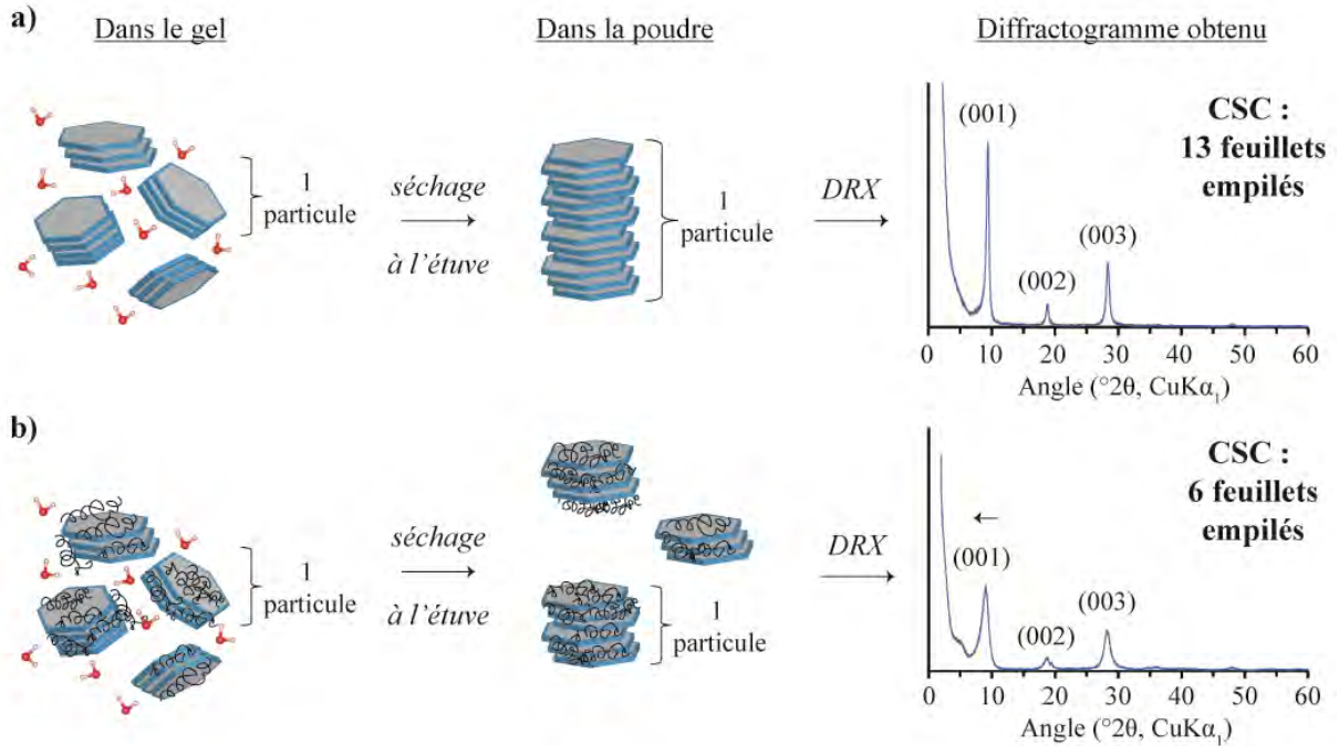
Figure 8 : Modèle évoquant l'influence du séchage sur l'empilement de particules de talc synthétique a) non fonctionnalisées, et b) fonctionnalisées par un adsorbat organique ou inorganique.
