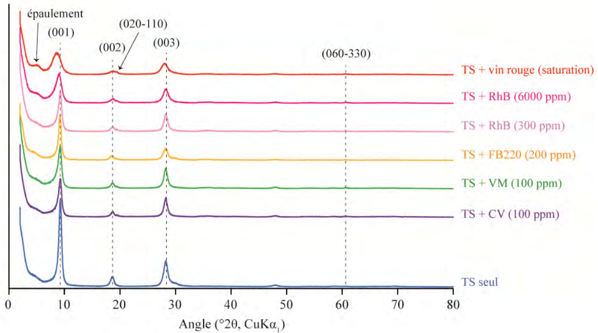
Figure 7 : Diffractogrammes des hybrides de talc synthétique (TS) obtenus avec divers composés organiques (CV : Crystal Violet ; VM : Vert Malachite ; FB220 : Fluorescent Brightener 220 ; RhB : Rhodamine B). Les résultats sont comparés au diffractogramme du talc synthétique seul, non fonctionnalisé.
