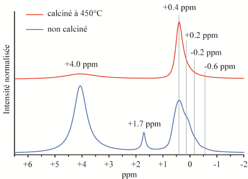
Figure 8 : Influence de la calcination sur le spectre RMN ^1\text{H} de l'échantillon 'TS – calcination' (vitesse MAS : 45 kHz).
