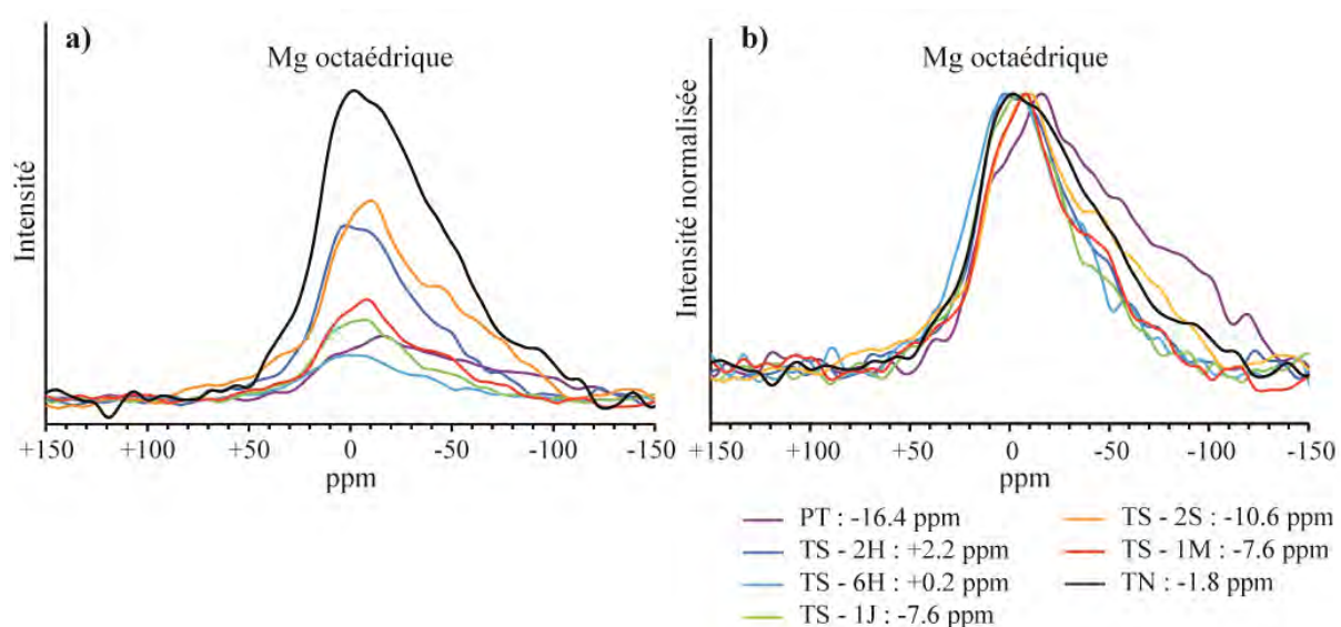
Figure 16 : Influence de la cristallinité sur le spectre RMN ^{25}\text{Mg} du talc synthétique a) avant et b) après normalisation. Les résultats sont comparés à un prototalc amorphe (PT) et un talc naturel (TN).
