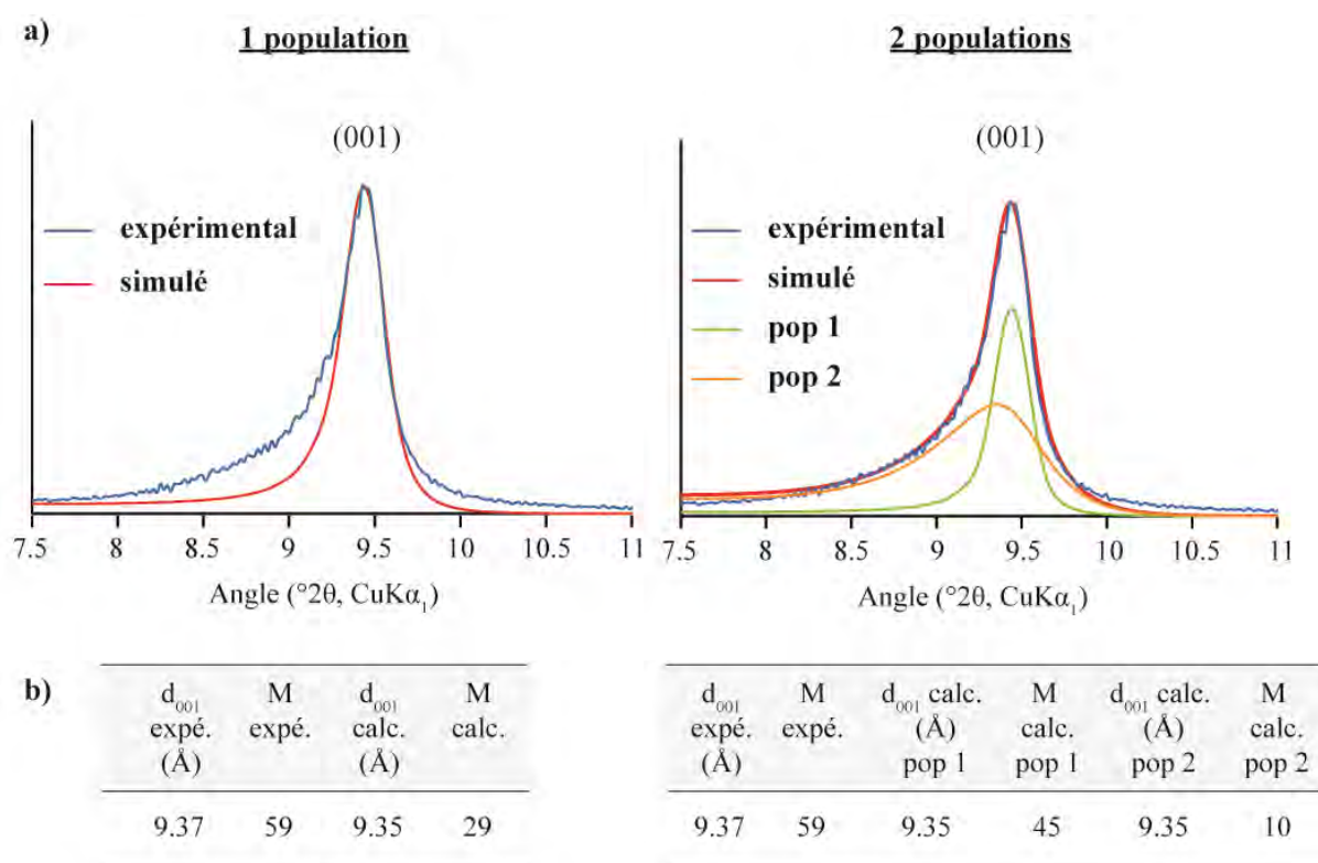
Figure 4 : a) Simulation de la raie (001) d'un talc synthétique d'1 mois de synthèse (TS – 1M) en prenant en compte une population ou deux populations de particules de CSC différentes. b) Valeurs des paramètres d_{001} et M (nombre de feuillets empilés moyens) obtenus par la simulation.
