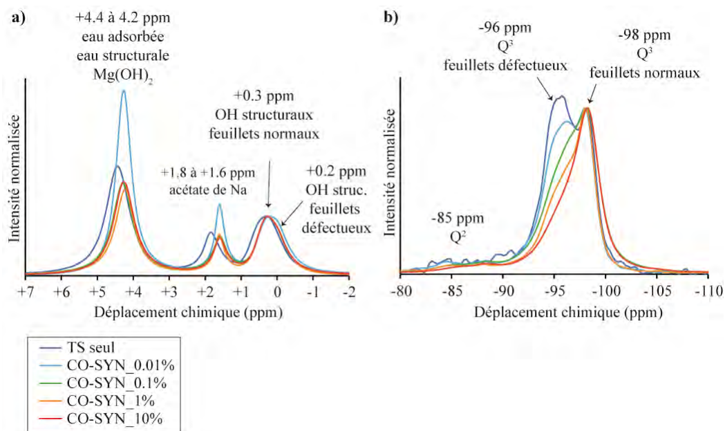
Figure 13 : Nouvelle interprétation a) des spectres RMN 1 H et b) RMN 29 Si des hybrides ‘talc synthétique – AuNPs’ élaborés avec le protocole CO-SYN (vitesses MAS : 8 kHz). Les pourcentages indiqués dans la légende correspondent à la concentration massique de AuNP introduite dans les échantillons.
