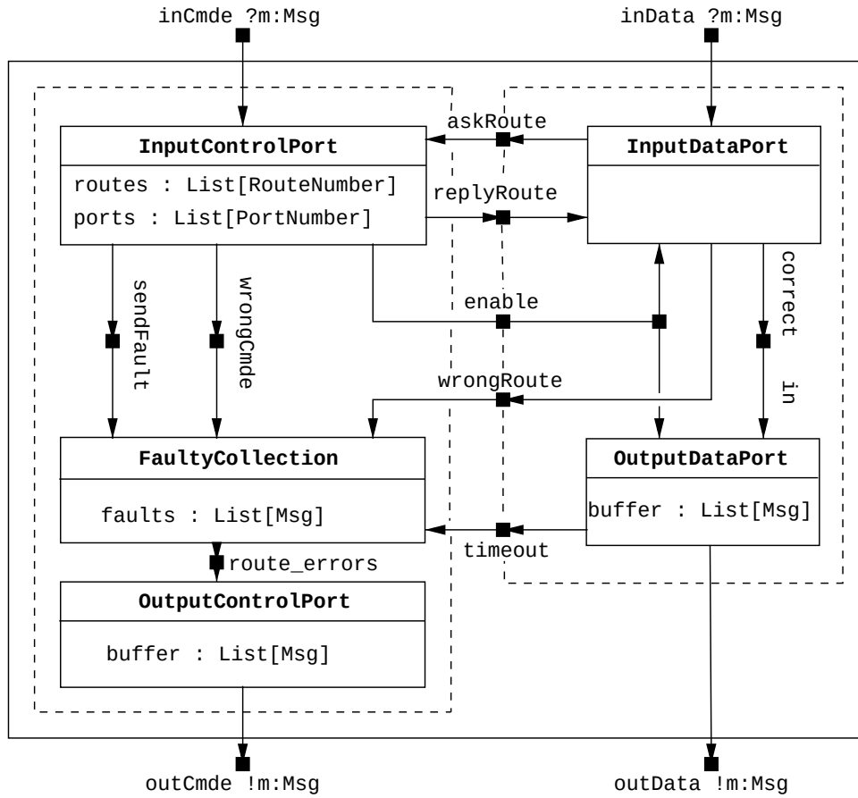
Figure D.6 : Vue interne du nœud de transit.
