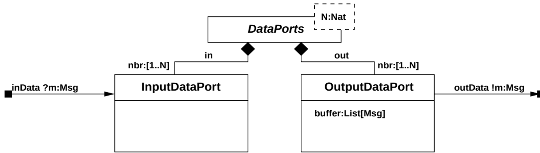
Figure 3.13 : DataPorts – Diagramme de composition
