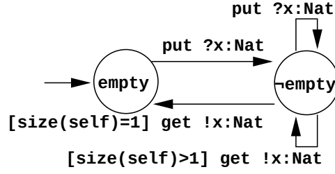
Figure 2.3 : Buffer non borné – Système de transitions symboliques
