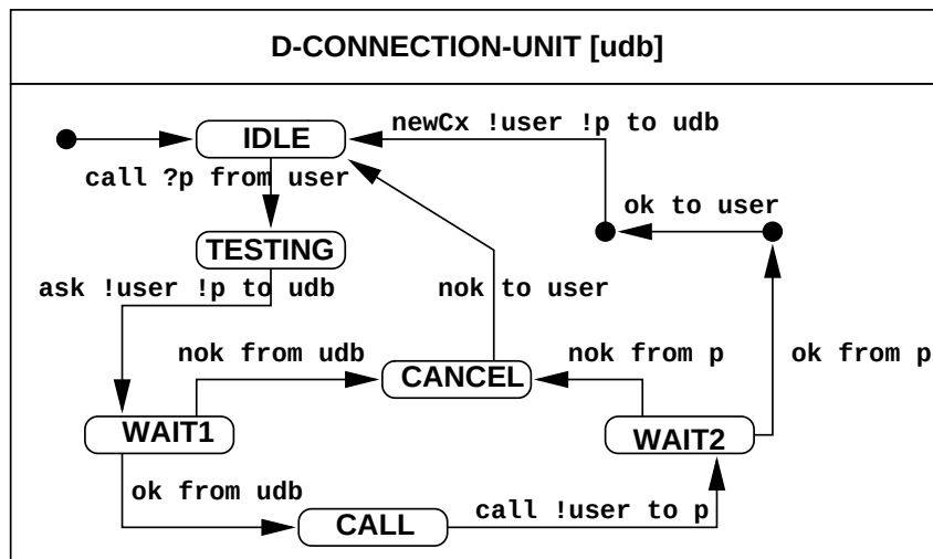
Figure C.13 : Unité de connexion – STS dynamique
