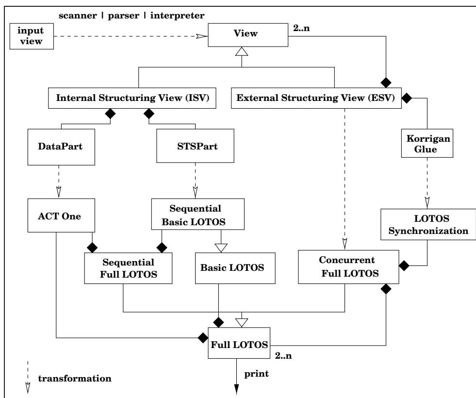
Figure 4.7 : ASK– Processus de traduction KORRIGAN en LOTOS
