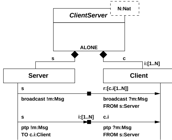
Figure 3.19 : Patron Client-Serveur
