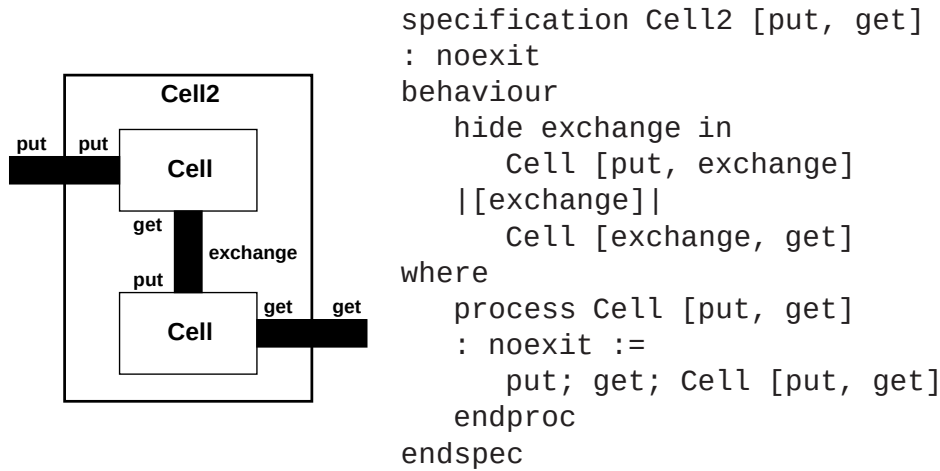
Figure 1.3 : Cellule de taille 2 – LOTOS
