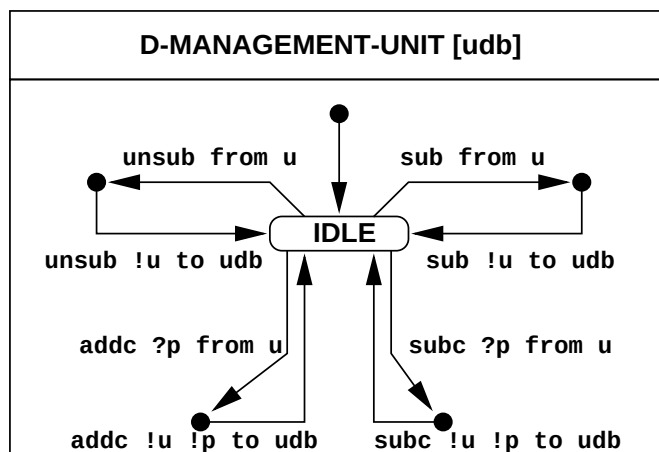
Figure C.19 : Unité de gestion – STS dynamique
