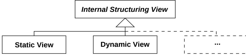
Figure 2.9 : Diagramme de classes – Structuration interne
