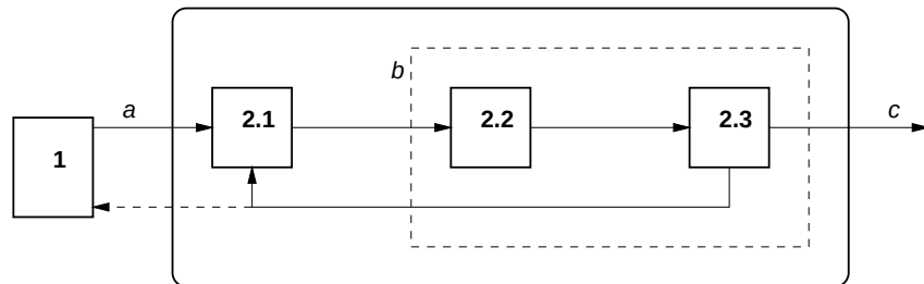
Figure 3.5 : Dépendances entre étapes : activité concurrente.
