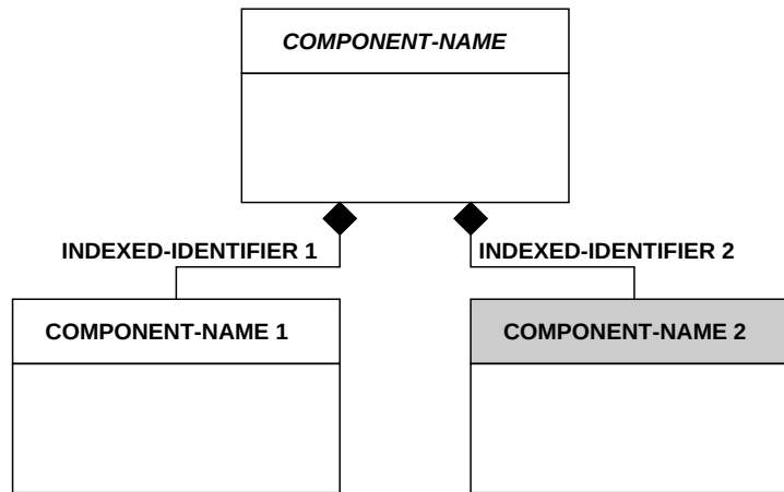
Figure A.20 : Notation graphique – Diagrammes de composition (IV, 2)
