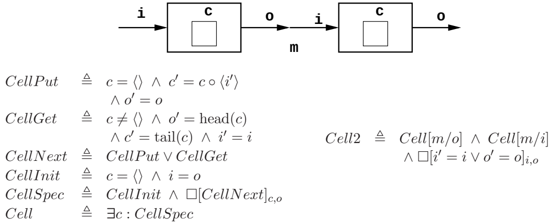
Figure 1.4 : Cellule de taille 2 – TLA
