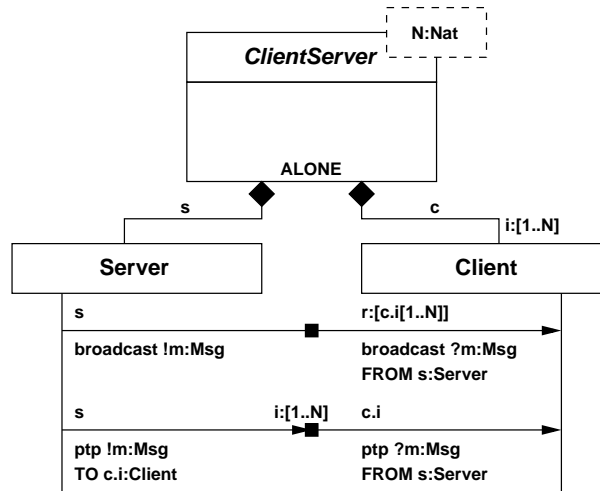
Figure 3.19 : Patron Client-Serveur
