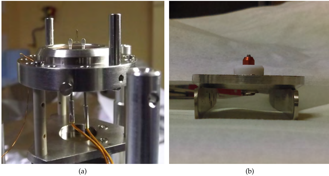
FIGURE 2.7 – Porte-pointe dans le cas d'une pointe de tungstène (a) et d'une pointe de diamant (b). Sur le premier, on remarque les deux tiges accrochées au pont de tungstène et permettant le flash de la pointe.
